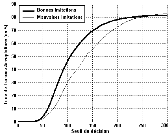
FIGURE 6.2: Courbes de taux de fausses acceptations en fonction du seuil de décision sur les imitations de “bonne” et de “mauvaise” qualité de la base MCYT-100.
