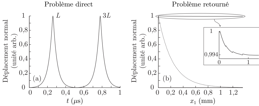
Fig. 6.1 – (a) Déplacement normal généré sur la face arrière par une source volumique enfouie d'extension latérale infinie. (b) Image de la source volumique enfouie d'extension latérale infinie après résolution du problème retourné.
