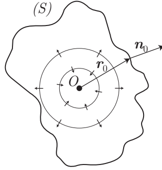
Fig. 5.3 – Schéma de principe de la cavité à retournement temporel.
