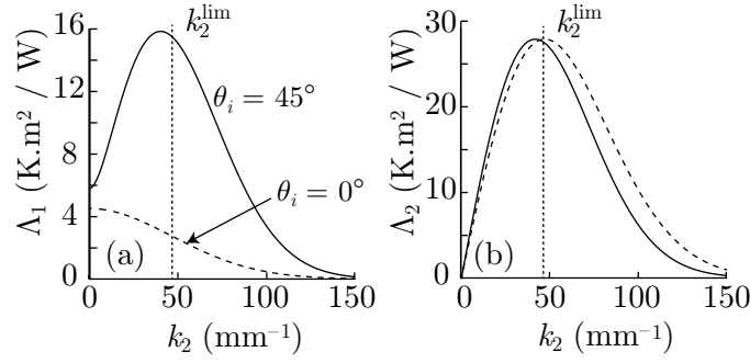
Fig. 3.3 – Projection normalisée de \widehat{\nabla T} sur (a) la direction \mathbf{x}_1 et (b) la direction \mathbf{x}_2 en fonction de k_2 pour \theta_i = 0^\circ (traits pointillés) et \theta_i = 45^\circ (traits pleins) à la pulsation \omega_c ( \theta_i = 0^\circ ). Les lignes pointillées verticales montrent le nombre d'onde limite k_2^{\text{lim}} .
