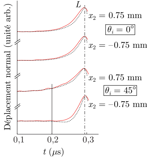
Fig. 4.4 – Zoom sur les premières impulsions de compression pour les deux positions du point d'observation x_2 = \pm 0,75 mm et les deux orientations de la source : \theta_i = 0^\circ et \theta_i = 45^\circ .
