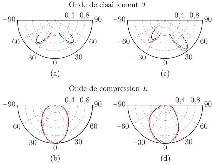
Fig. 4.6 – Les amplitudes des ondes (a) de cisaillement et (b) de compression pour \theta_i = 0^\circ et les amplitudes des ondes (c) de cisaillement et (d) de compression pour \theta_i = 45^\circ sont tracées en fonction de \theta_{\text{obs}} pour les résultats simulés (traits pleins) et expérimentaux (points).
