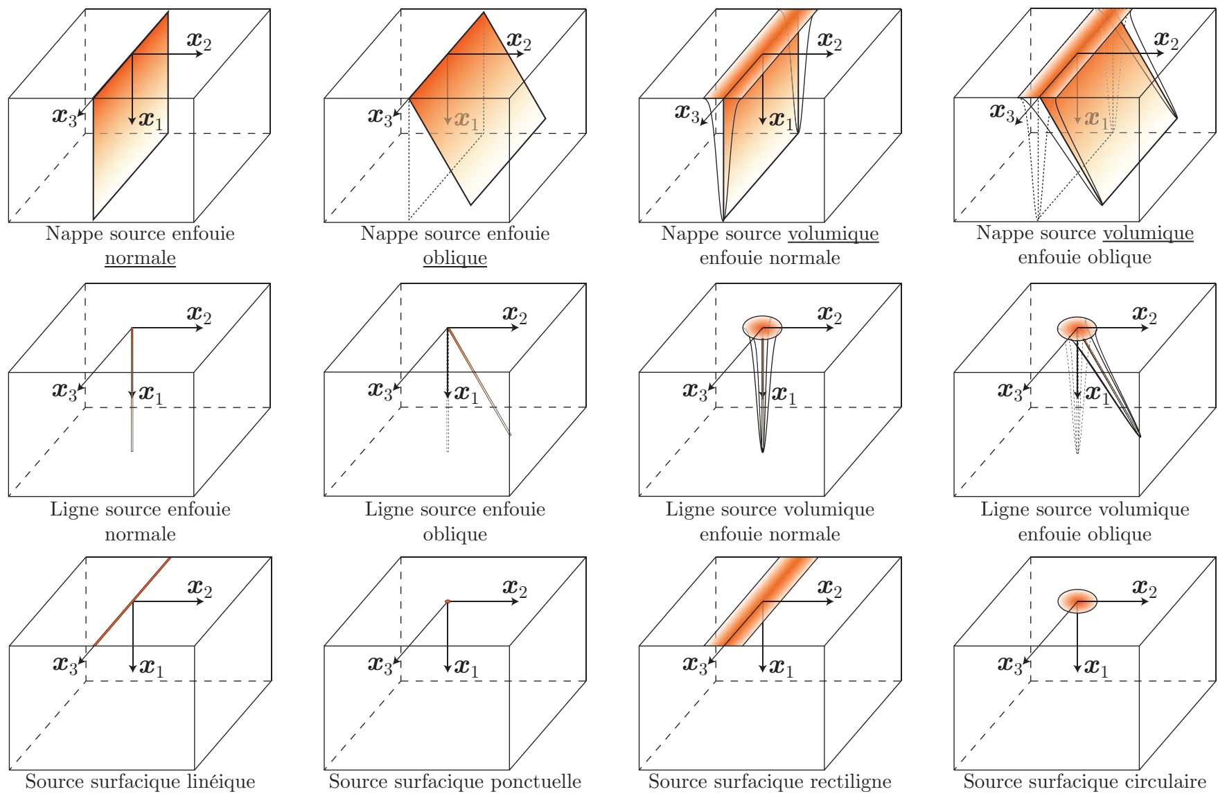
Fig. 1.1 – Représentation schématique des différentes sources acoustiques considérées dans ce manuscrit.
