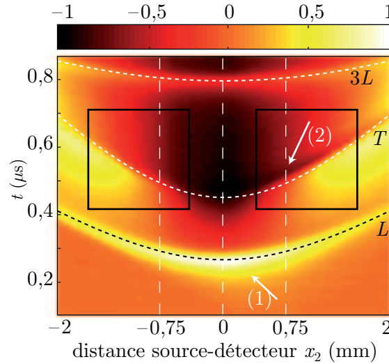
Fig. 4.2 – Déplacement normal normalisé mesuré sur la face arrière de la plaque pour \theta_i = 45^\circ en fonction de t et de x_2 . Les lignes pointillées L , T et 3L décrivent les temps d'arrivée théoriques des ondes de compression, des ondes de cisaillement et des ondes de compression s'étant réfléchies deux fois sans conversion de mode, respectivement. Les flèches (1) et (2) pointent des asymétries. Les rectangles noirs limitent les zones où les amplitudes des ondes de cisaillement sont extraites.
