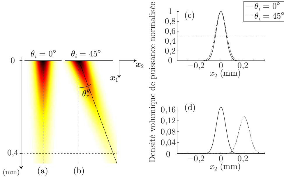
Fig. 3.2 – Densité volumique de puissance initiale déposée par le faisceau laser pour (a) \theta_i = 0^\circ et (b) \theta_i = 45^\circ . Comparaison selon la direction x_2 pour (c) x_1 = 0 mm et (d) x_1 = 0,4 mm de la densité de puissance pour \theta_i = 0^\circ (traits pleins) et \theta_i = 45^\circ (traits point-tirets).
