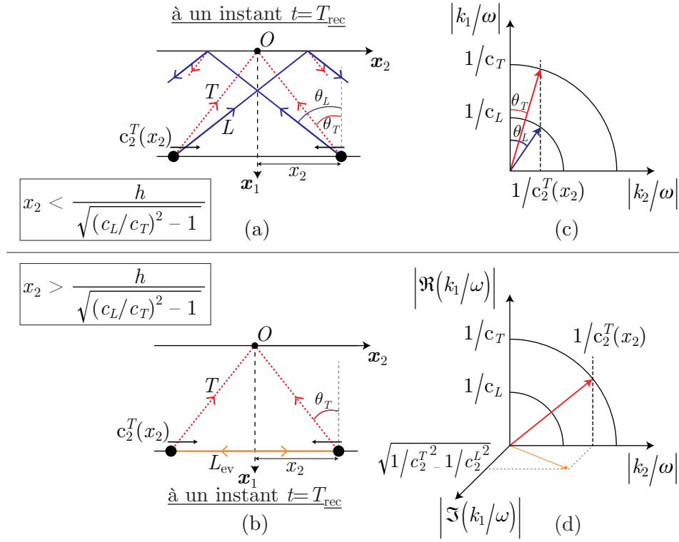
Fig. 6.4 – Illustrations des ondes générées par deux sources en mouvement à la vitesse \pm c_2^T(x_2) au point de mesure d'abscisse x_2 : (a) dans le cas |x_2| < h/\sqrt{(c_L/c_T)^2 - 1} et (b) dans le cas opposé. (c)-(d) Diagrammes des lenteurs de phases pour un matériau isotrope associé respectivement aux cas (a) et (b). Les traits pointillés verticaux représentent dans les deux cas la lenteur des sources en mouvement.
