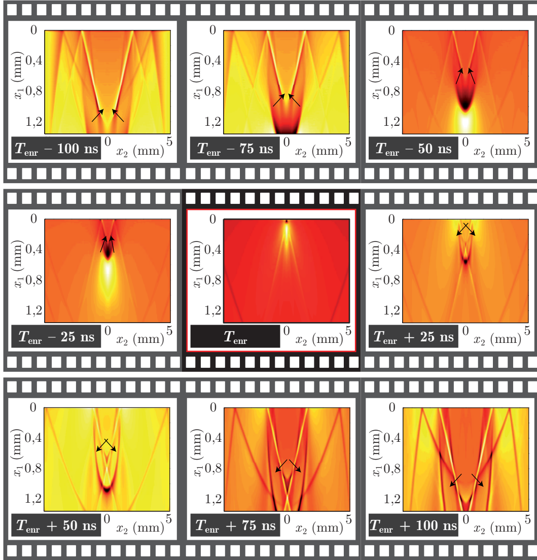
Fig. 7.3 – Composantes normales du champ de déplacement solution d'un problème retourné en fonction de x_1 et de x_2 , le temps évoluant d'une vignette à la suivante.
