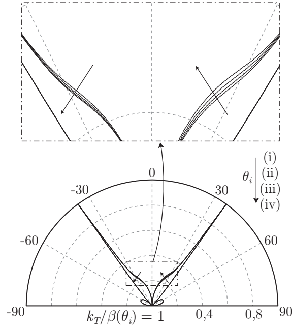
Fig. 1.12 – Variation du diagramme de directivité dans le verre Schott NG1 des ondes de cisaillement pour un rapport k_T/\beta(\theta_i) de 1 en fonction de \theta_i . Les valeurs de \theta_i sont (i) 0^\circ , (ii) 15^\circ , (iii) 30^\circ et (iv) 45^\circ .
