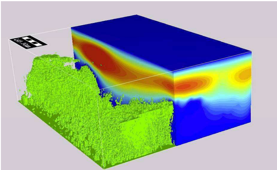
Figure 6.13 : Simulation numérique de la distribution du champ des vitesses longitudinales
