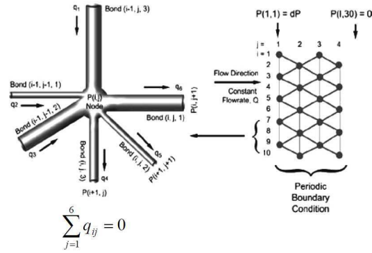
Figure 2.12 : schéma d'un réseau composé de plusieurs tubes capillaires interconnectés.
