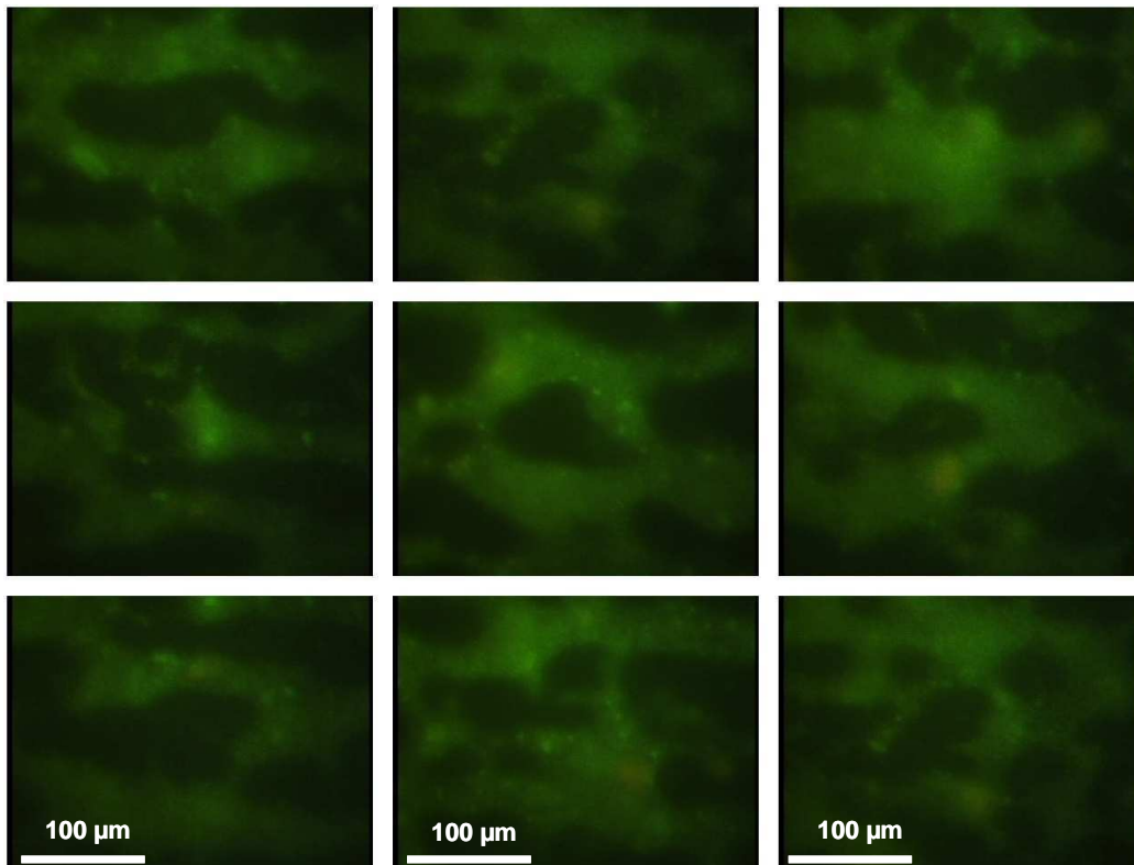
Figure 6.9 : - Structure de biofilms de P. putida sous écoulement à 160 µl/min et adhérents sur support de verre. Age = 8 j - Arrangement de la structure dans la direction de l'écoulement ; observations effectuées après fluorescence Live/Dead ; agrandissement 40X ; à différentes positions
