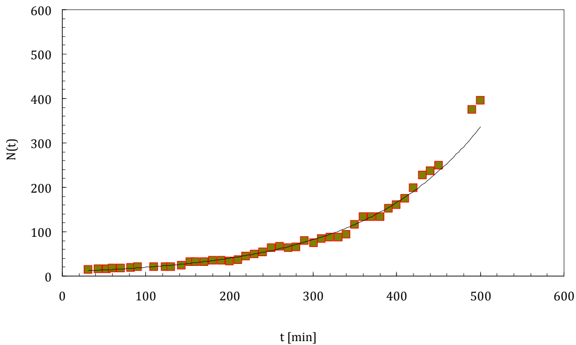
Figure 5.15 : Ajustement des données expérimentales pour une des expériences menées à T_w = 9,6 mPa.
