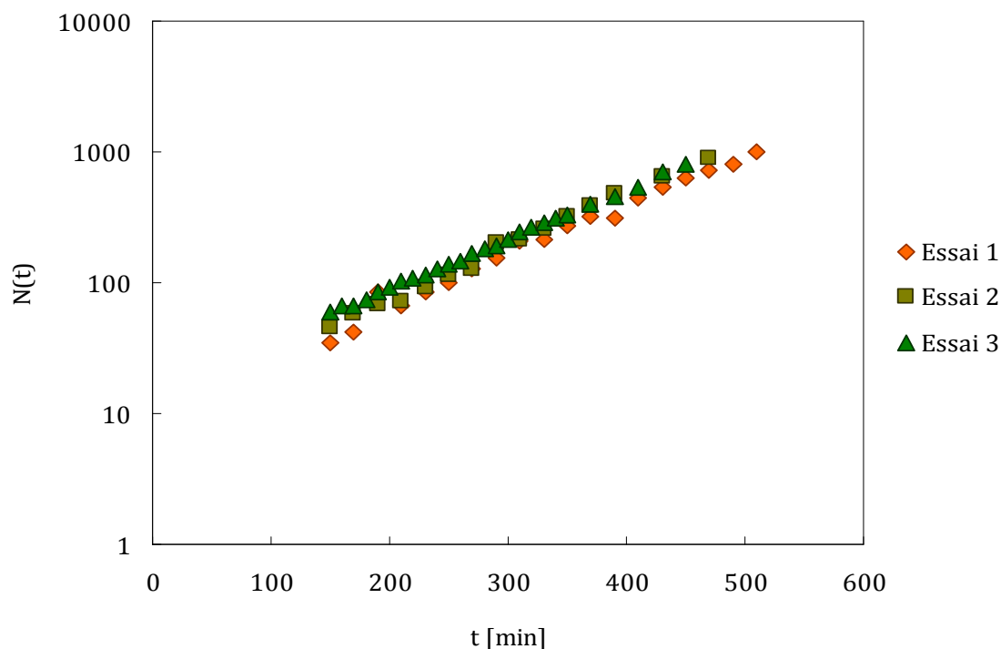
Figure 5.22 : Courbe de croissance pour 3 essais à T_w = 76,8 mPa
