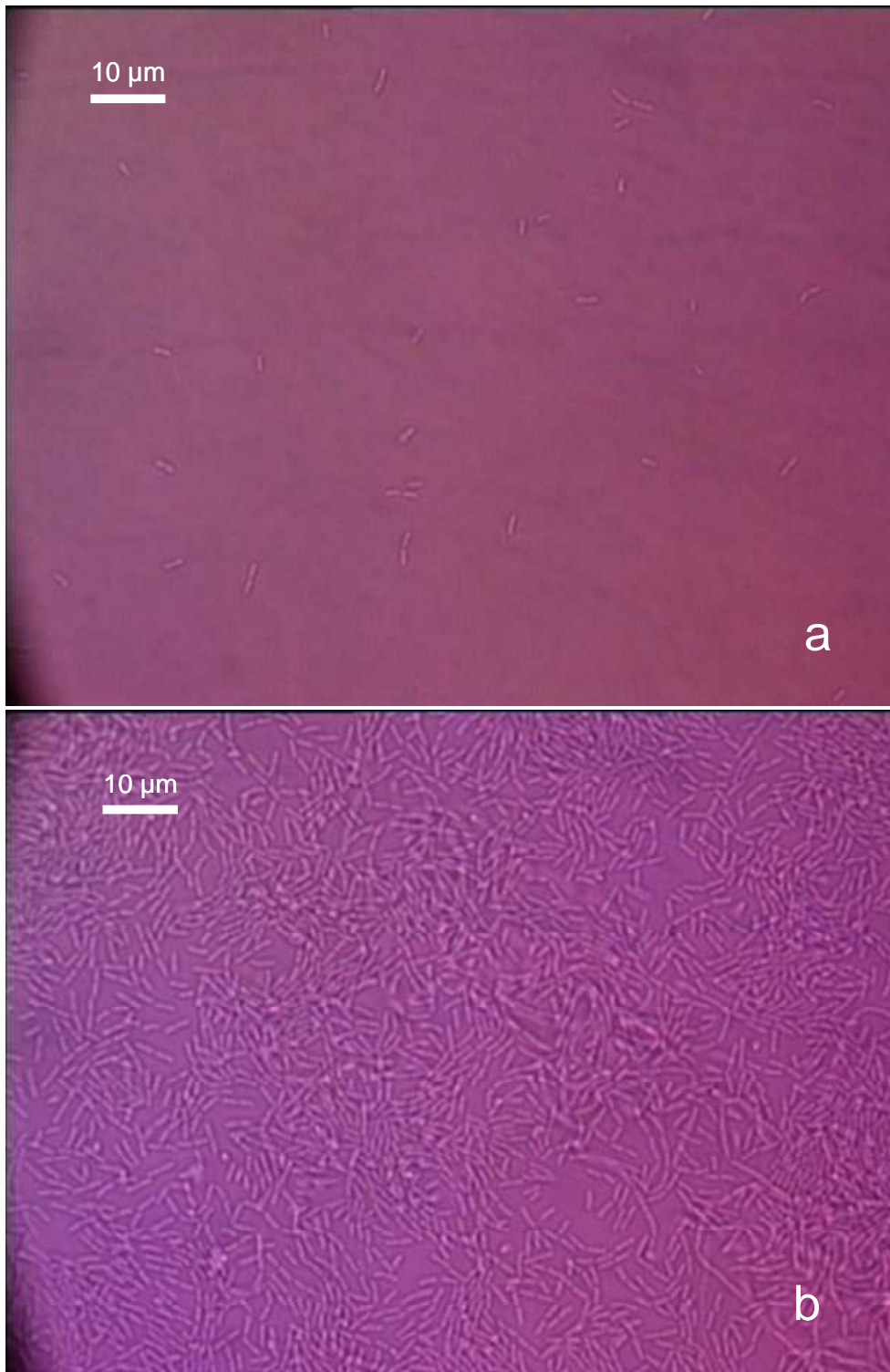
Figure 6.2 : Développement de P. putida adhérees sur paroi de verre et soumises à un écoulement cisailé de milieu LB sans peptone à 20 mg/l de phénol, à très faible débit, Q = 25,5 \mu\text{l}/\text{min} , observation à l'objectif 100x à 25 \pm 1 \text{ }^\circ\text{C} . a) t = 30 \text{ min} : 1eres phases de l'adhésion. b) t = 23\text{h} : phases de biofilm.
