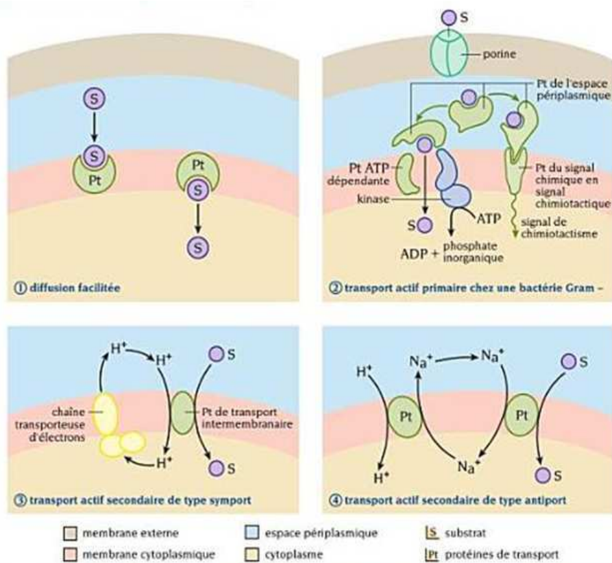
Figure 5.26 : Schéma montrant les différents modes de transport de substrat à travers une membrane bactérienne
