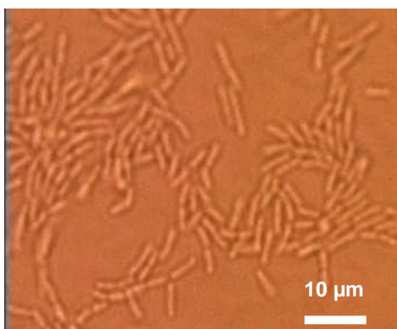
Figure 4.1 : Cellules de P. putida souche 6521 adhérées sur substrat de verre
