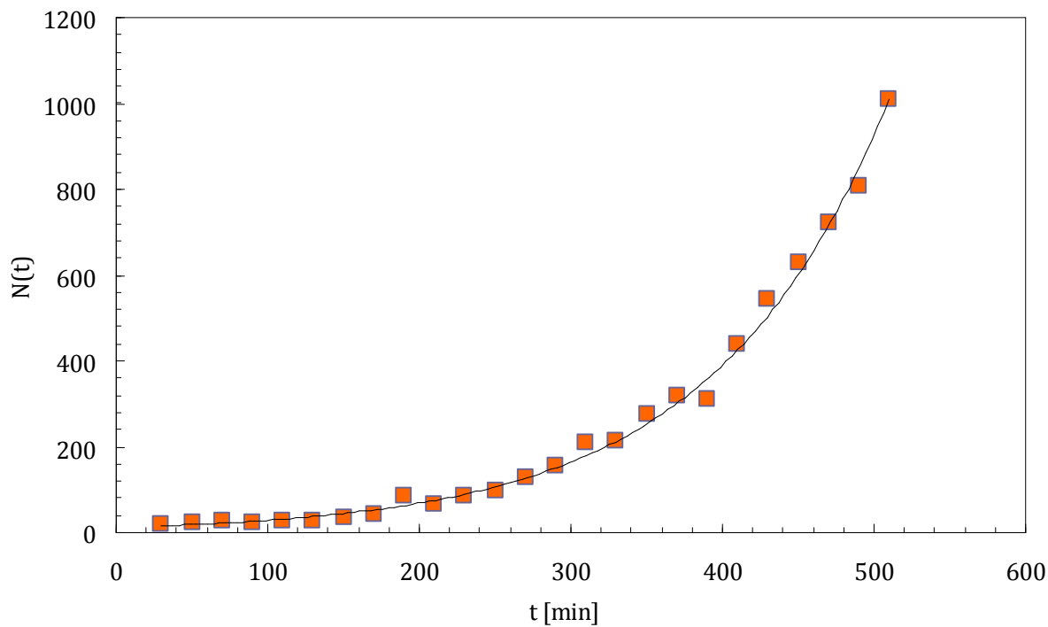
Figure 5.16 : Ajustement des données expérimentales pour une des expériences menées à T_w = 76,8 mPa.
