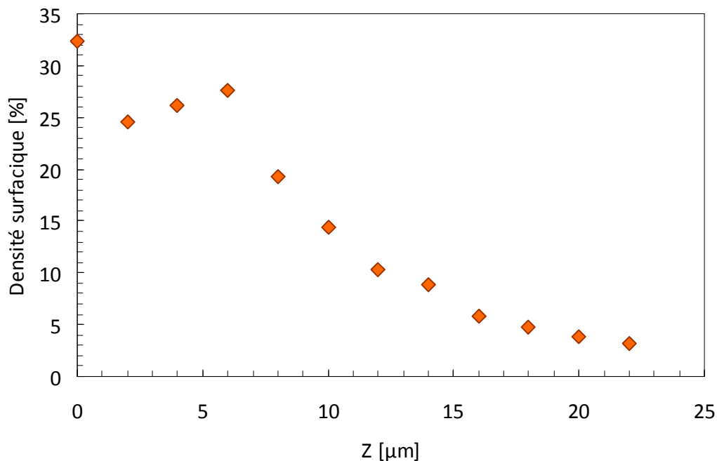
Figure 6.4 : Evolution de la densité cellulaire surfacique n fonction de la hauteur z par rapport au support.
