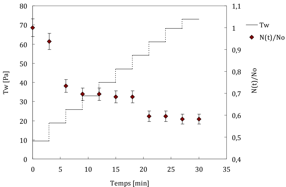
Figure 5.4 : Evolution de N/N_0 (proportion de cellules adhérentes rapportée au nombre de cellules initialement adhérentes N_0 , N_0 = 79 ) en fonction de la contrainte pariétale appliquée ; pour des cellules suspendues dans du NaCl à 0.15 mM. Le premier cisaillement est appliqué après un T_c de 45min sur support en claire de vinyle optique. Température = 24 \pm 1^\circ\text{C} .
