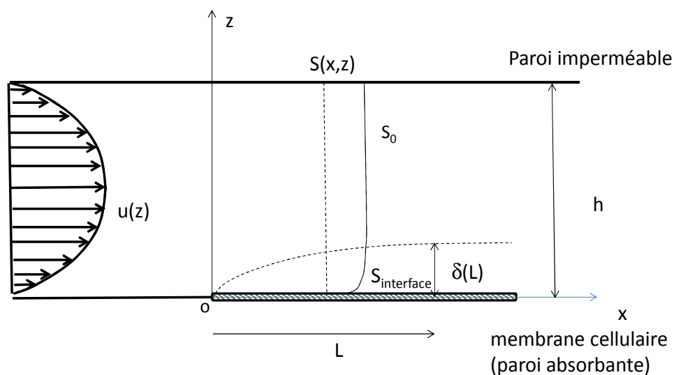
Figure E.1 : Schéma idéalisé du développement d'une couche limite de concentration sur paroi absorbante.
