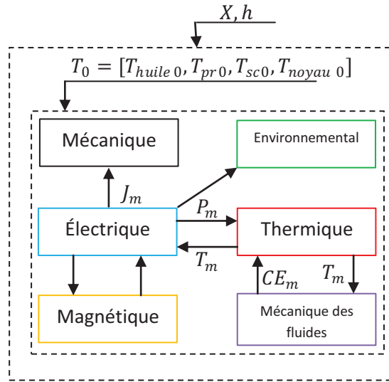
Figure IV.17 : Modèle multidisciplinaire du TT
