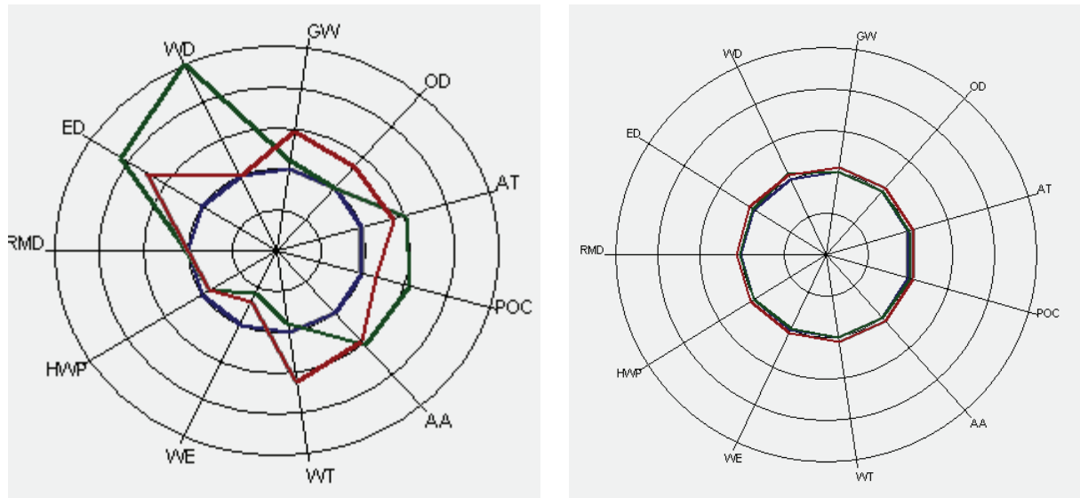
Figure II.7 : Comparaison des effets environnementaux des trois huiles sur la phase de fabrication et sur le cycle de vie du transformateur (bleu : huile C, rouge : huile B et vert : l'huile A)
