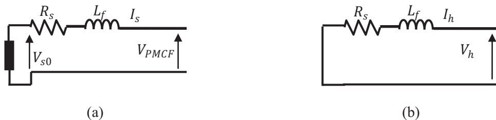
Figure IV.29 : Schéma équivalent d'un secondaire du transformateur pour le fondamental (a) et les harmoniques (b)
