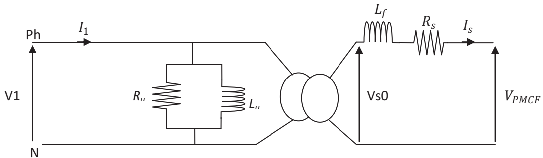
Figure IV.6 : Schéma électrique équivalent du transformateur de traction
