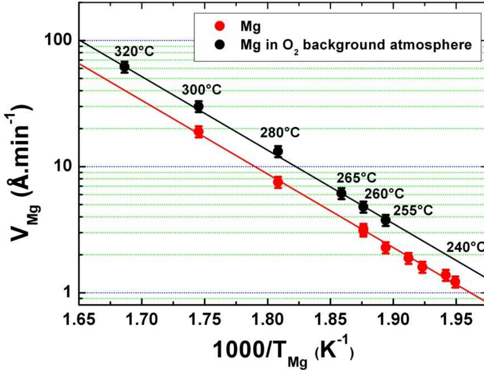
Figure 2.19: Evolution du taux de dépôt du Mg sur la balance à quartz pour l'évaporation de Mg sous ultravide et la co-évaporation de Mg sous flux d'O 2 en fonction de 1/T_{Mg} en échelle semi-logarithmique.
