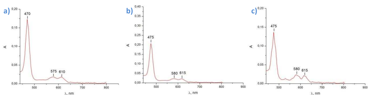
Figure 57 : Analyses UV-Visible de la métalloporphyrine \text{Mn(TPP)OAc} dans le dichlorométhane (a) \text{Mn(TPP)OAc} (b) \text{Mn(TPP)OAc} + imidazole ( t = 0 min) (c) \text{Mn(TPP)OAc} après 1 h d'époxydation dans \text{MOPyrroNTf}_2 sous ultrasons
