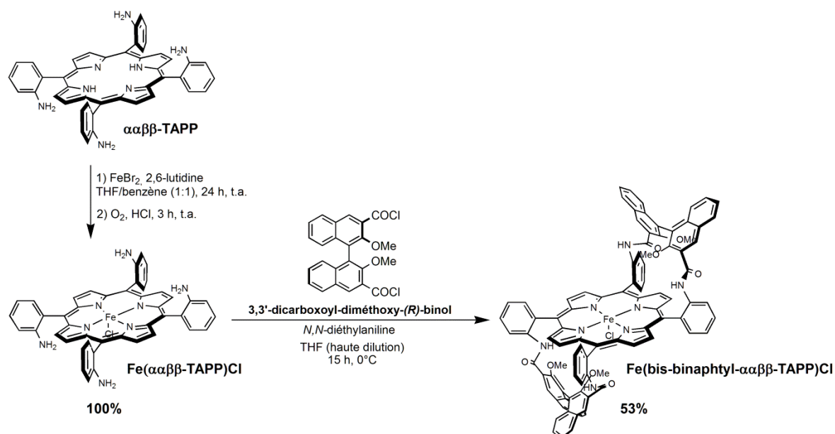
Figure 37 : Synthèse de la porphyrine chirale Fe(bis-binaphthyl- \alpha\alpha\beta\beta -TAPP)Cl
