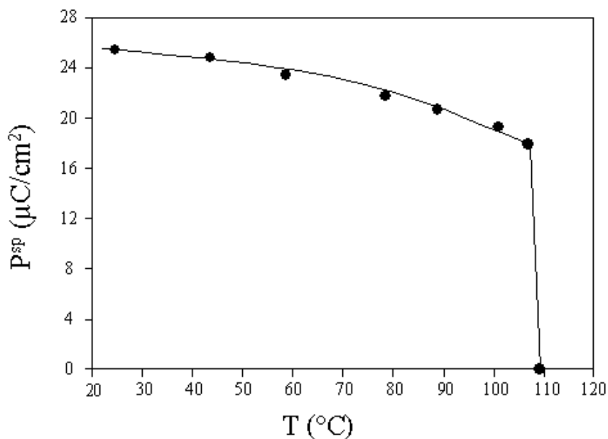
Figure I.9 : Évolution de la polarisation spontanée en fonction de la température dans un cristal ferroélectrique de \text{BaTiO}_3 [Merz1953].
