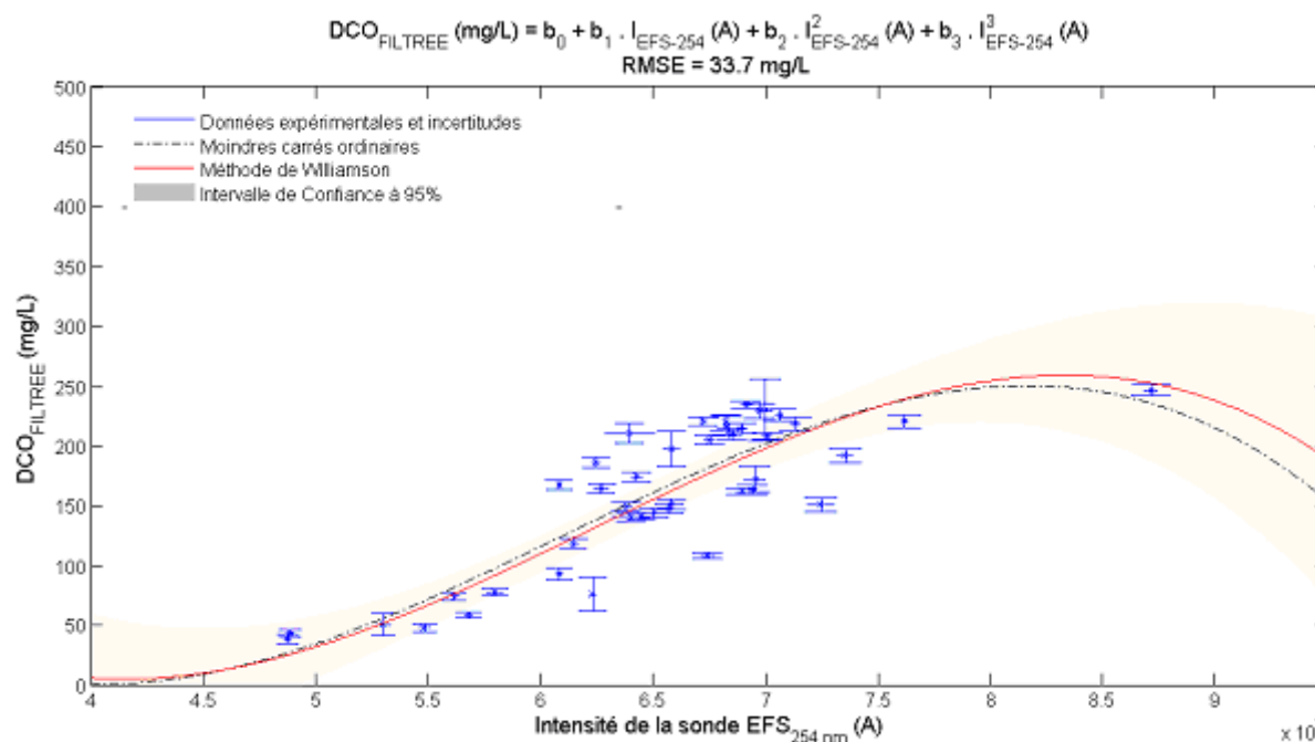
Figure III-15 : Polynôme du troisième degré : régression entre DCO dissoute et l'intensité de la sonde EFS à 254 nm
