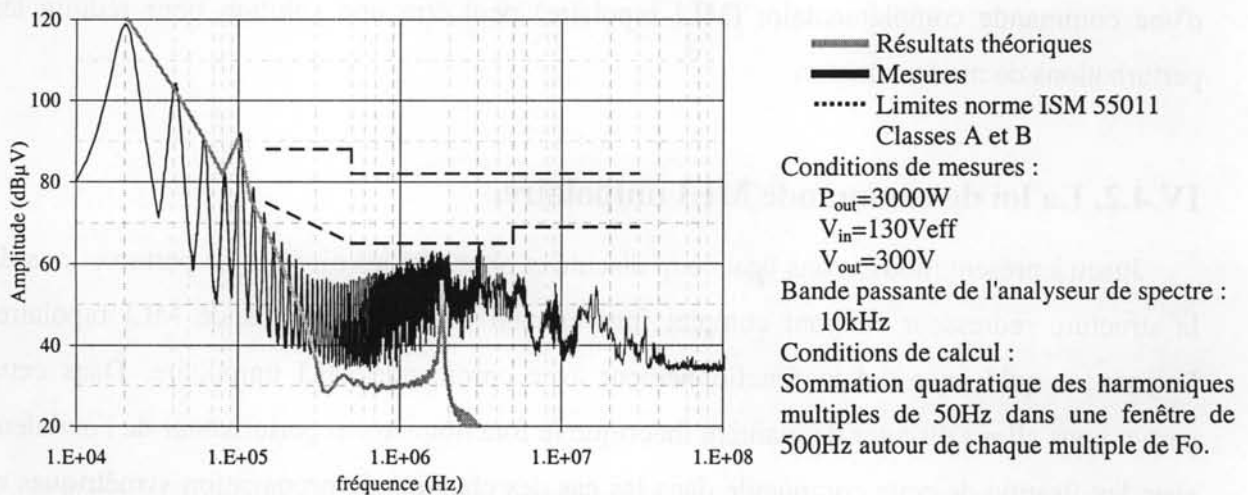
Figure IV.35. Représentation spectrale des perturbations conduites mesurées dans le RSIL (résistance de mesure supérieure).
