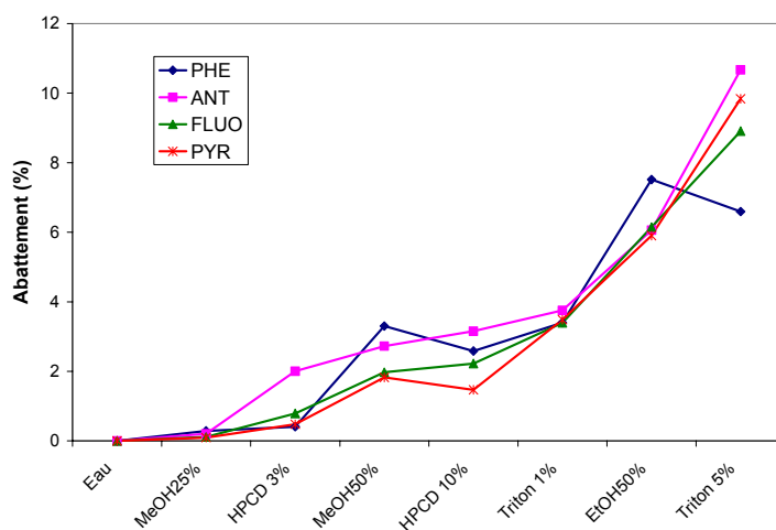
Figure 140 : Abattements de 4 HAP après une expérience en batch avec divers produits sur le sol CNRSP4 (ratio L/S=3, TA)
