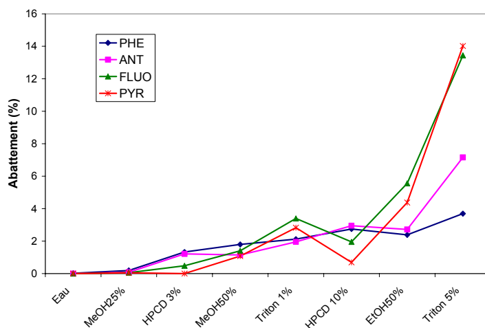
Figure 139 : Abattements de 4 HAP après une expérience en batch avec divers produits sur le sol CNRSP2 (ratio L/S=3, TA)
