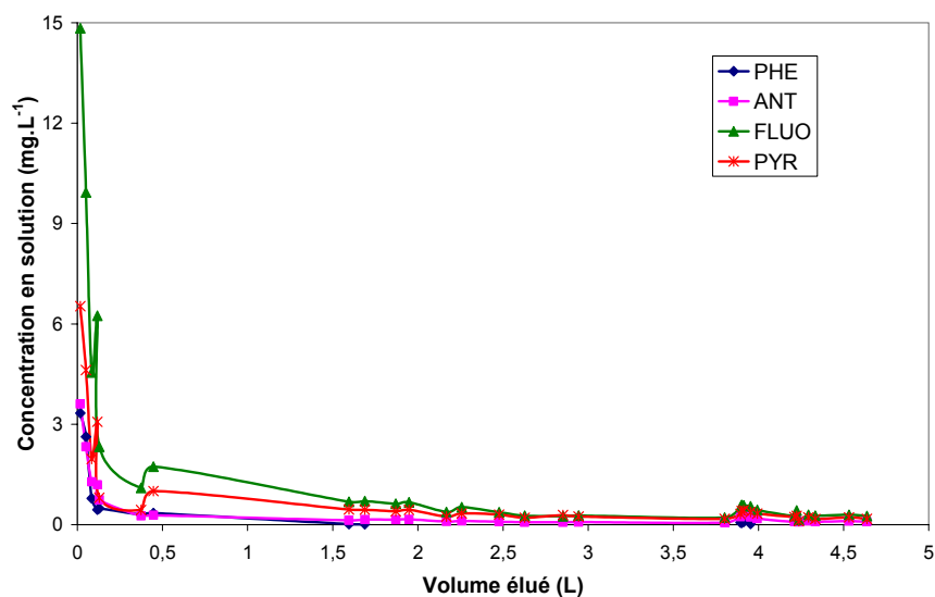
Figure 156 : Concentrations de 4 HAP en sortie de la colonne de sol CNRSSP4 ( [HPCD] = 100 \text{ g.L}^{-1} , débit = 0,22\text{-}0,28 \text{ mL.min}^{-1} )
