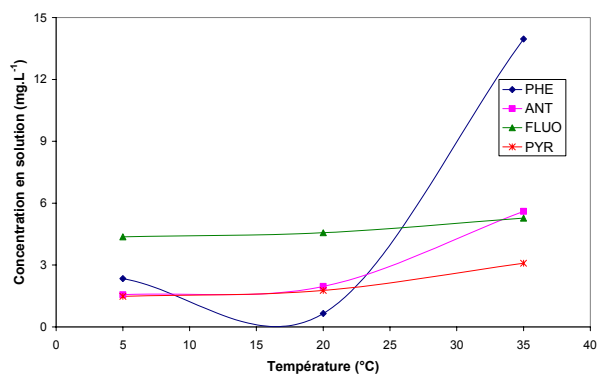
Figure 37 : Influence de la température sur l'extraction des HAP du sol CNRSSP4 ([HPCD]=30 g.L -1 , L/S=3)
