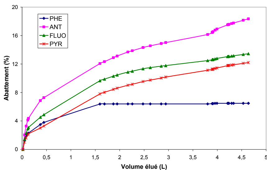
Figure 157 : Abattements de 4 HAP calculés à partir des concentrations en sortie de colonne de sol et de l'état initial du sol (sol CNRSSP4, [HPCD] = 100 \text{ g.L}^{-1} , débit = 0,22\text{-}0,28 \text{ mL.min}^{-1} )
