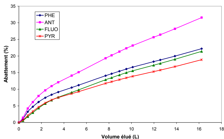
Figure 154 : Abatements de 4 HAP calculés à partir des concentrations en sortie de colonne de sol et de l'état initial du sol (sol CNRSSP2, [HPCD] = 30 \text{ g.L}^{-1} , débit = 0,25\text{-}0,43 \text{ mL.min}^{-1} )
