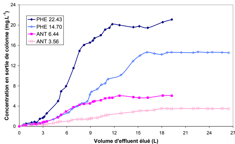
Figure 112 : Concentrations en PHE et ANT à la sortie de colonnes de 15,6 g de résine en fonction du volume élué à un débit de 5 \text{ mL.min}^{-1} (concentration entrante indiquée en légende)
