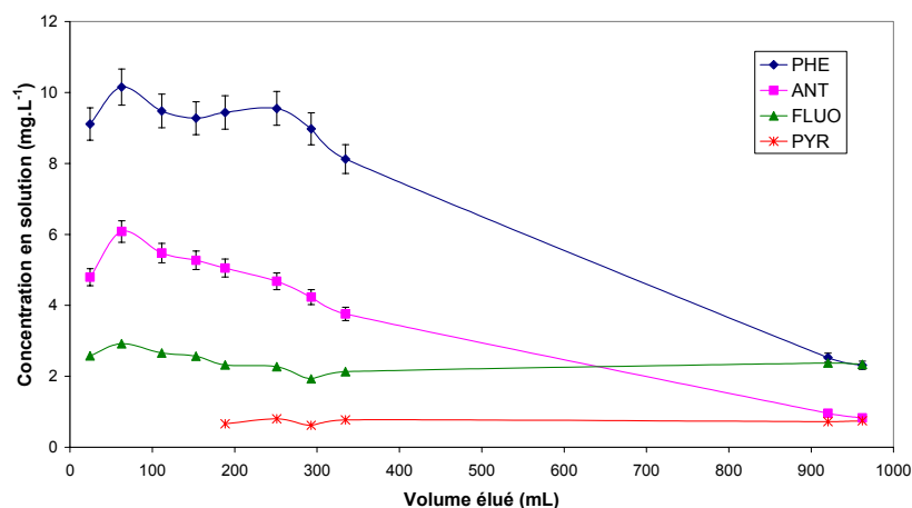
Figure 89 : Concentrations de 4 HAP en sortie de colonne de lixiviation (sol SITA, [HPCD] = 20 g.L -1 , débit = 0,70 mL.min -1 ), barres d'erreurs à \pm 5\%
