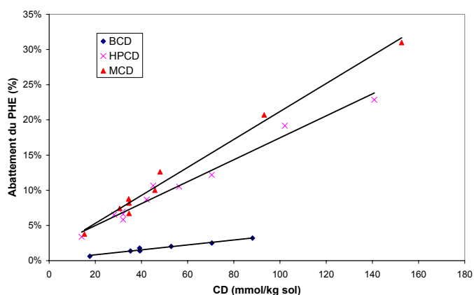
Figure 70 : Pourcentage de phénanthrène extrait en batch percolant par la BCD, HPCD et MCD en fonction de la quantité de cyclodextrine.
