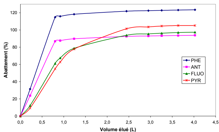
Figure 149 : Abattements de 4 HAP calculés à partir des concentrations en sortie de colonne de sol et de l'état initial du sol (sol SITA, [HPCD] = 100 \text{ g.L}^{-1} , débit = 0,27\text{-}0,62 \text{ mL.min}^{-1} )
