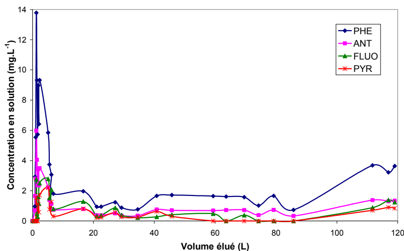
Figure 133 : Concentrations de 4 HAP en sortie de la colonne de sol ( [HPCD] = 50 \text{ g.L}^{-1} , débit = 3,4 - 4,6 \text{ mL.min}^{-1} )
