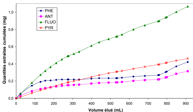
Figure 97 : Quantités cumulées de 4 HAP en sortie de colonne de lixiviation (sol POLDEN, [\text{HPCD}] = 20 \text{ g.L}^{-1} , débit = 0,65 \text{ mL.min}^{-1} )
