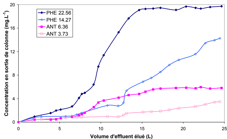
Figure 113 : Concentrations en PHE et ANT à la sortie de colonnes de 15,6 g de résine en fonction du volume élué à un débit de 3 \text{ mL.min}^{-1} (concentration entrante indiquée en légende)
