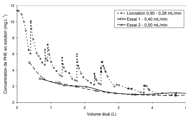
Figure 121 : Détail des concentrations en phénanthrène en sortie de la colonne de sol CNRSSP2 entre 0 et 5 L élués, pour différents débits (débits en légende, [HPCD]=30\text{g.L}^{-1} )
