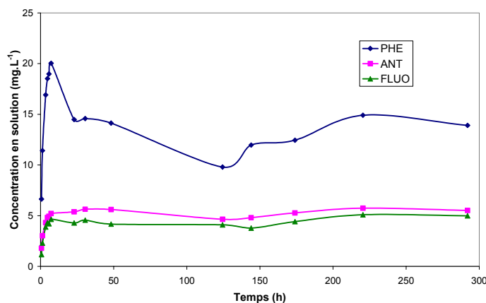
Figure 58 : Evolution temporelle de l'extraction des HAP sur le sol CNRSSP2 ( [HPCD]=30 \text{ g.L}^{-1} , L/S=3 , T_A )
