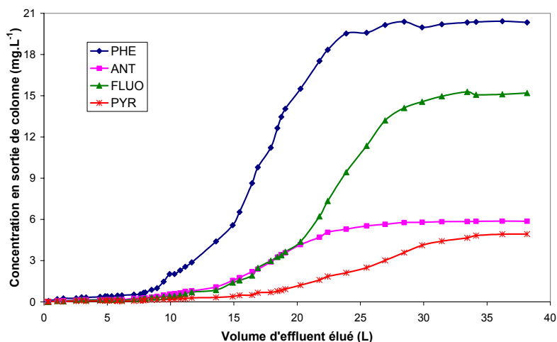
Figure 108 : Concentrations en HAP à la sortie d'une colonne de 15,6 g de résine en fonction du volume élué à un débit de 1 mL.min -1 (concentration entrante en mg.L -1 : [PHE]=20,47 ; [ANT]=5,95 ; [FLUO]=15,46 ; [PYR]=5,12)
