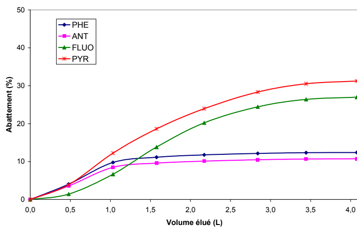
Figure 148 : Abattements de 4 HAP calculés à partir des concentrations en sortie de colonne de sol et de l'état initial du sol (sol SITA, [HPCD] 30 \text{ g.L}^{-1} , débit = 0,33\text{-}0,45 \text{ mL.min}^{-1} )
