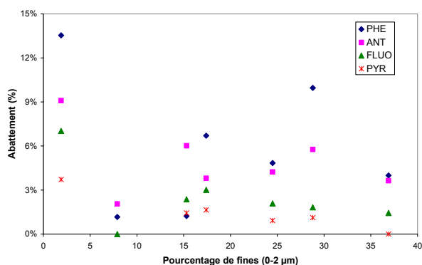
Figure 75 : Taux d'abattement pour 4 HAP en fonction du taux de fines (0-2 μm) pour 7 sols. ( [HPCD]=30 \text{ g.L}^{-1} , batch, L/S=3 , TA)
