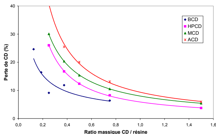
Figure 84 : Perte de CD en fonction du ratio massique entre la CD et la résine, en milieu agité (effluent de lavage de sol, 25°C, 3h)
