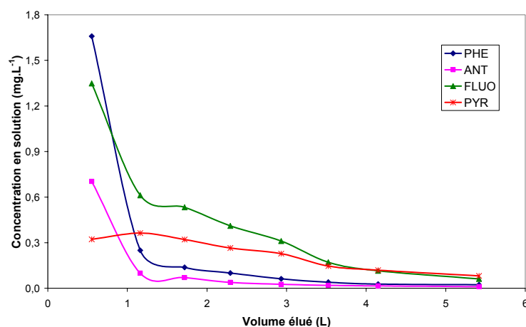
Figure 144 : Concentrations de 4 HAP en sortie de la colonne de sol SITA ( [HPCD] = 30 \text{ g.L}^{-1} , débit = 0,38\text{-}0,45 \text{ mL.min}^{-1} )
