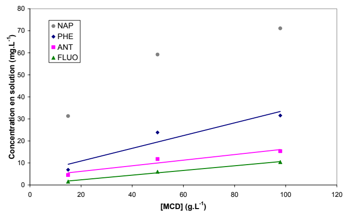
Figure 141 : Influence de la concentration en MCD sur l'extraction des HAP (sol SITA, L/S=3, TA)
