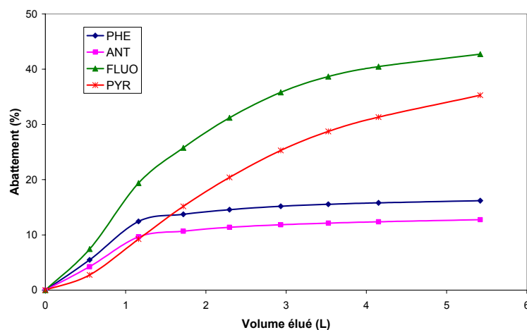
Figure 147 : Abattements de 4 HAP calculés à partir des concentrations en sortie de colonne de sol et de l'état initial du sol (sol SITA, [HPCD]=30 \text{ g.L}^{-1} , débit = 0,38\text{-}0,45 \text{ mL.min}^{-1} )
