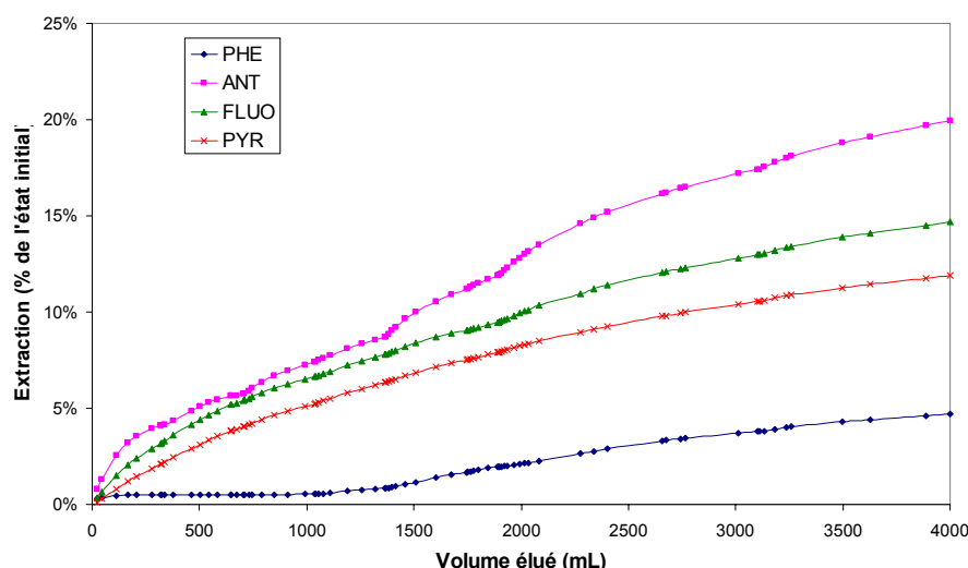
Figure 103 : Abattements de 4 HAP calculé à partir des concentrations de 4 HAP en sortie de colonne de lixiviation (sol CNRSSP 4, [\text{HPCD}] = 30 \text{ g.L}^{-1} , débit : 0-1890 mL : 0,65\text{-}0,80 \text{ mL.min}^{-1} , 1890-4000mL : 0,27 \text{ mL.min}^{-1} ).
