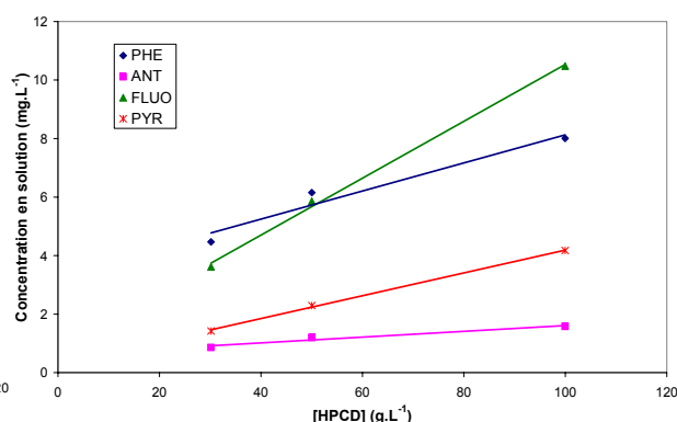
Figure 39 : Influence de la concentration en HPCD sur l'extraction des HAP (sol POLDEN, L/S=3, TA)
