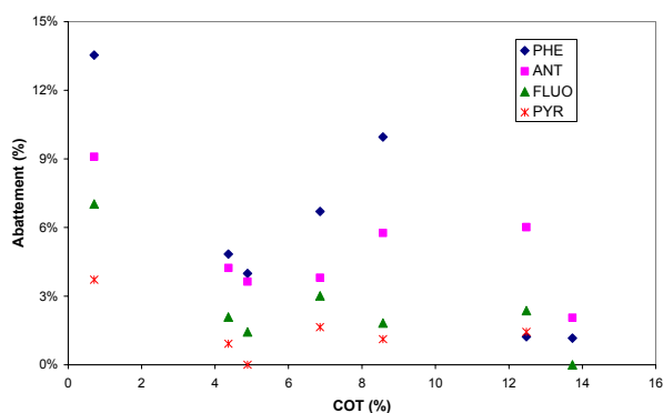
Figure 74 : Taux d'abattement pour 4 HAP en fonction du taux de COT pour 7 sols. ( [HPCD]=30 \text{ g.L}^{-1} , batch, L/S=3 , TA)
