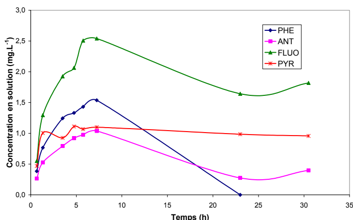
Figure 59 : Evolution temporelle de l'extraction des HAP sur le sol CNRSSP4 ( [HPCD]=30 \text{ g.L}^{-1} , L/S=3 , TA)
