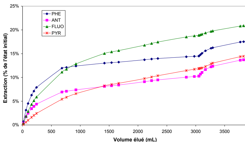
Figure 99 : Abattement de 4 HAP calculé à partir des concentrations en sortie de colonne de lixiviation et de l'état initial du sol (sol POLDEN, [HPCD] = 20 \text{ g.L}^{-1} , débit = 0,50 \text{ mL.min}^{-1} )
