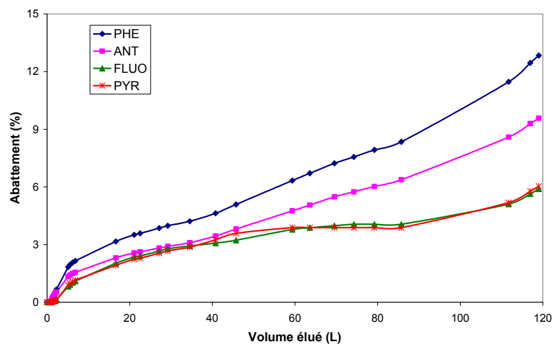
Figure 159 : Abattements de 4 HAP calculés à partir des concentrations en sortie de colonne de sol et de l'état initial du sol ( [HPCD] = 50 \text{ g.L}^{-1} , débit = 3,4 - 4,6 \text{ mL.min}^{-1} )
