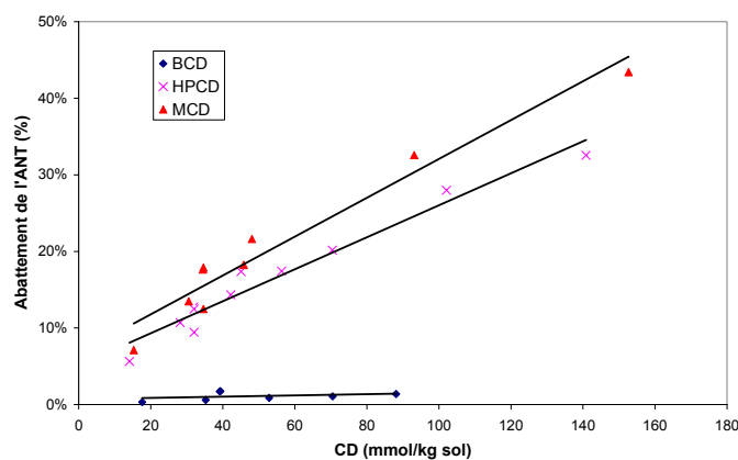
Figure 71 : Pourcentage d'anthracène extrait en batch percolant par la BCD, HPCD et MCD en fonction de la quantité de cyclodextrine.
