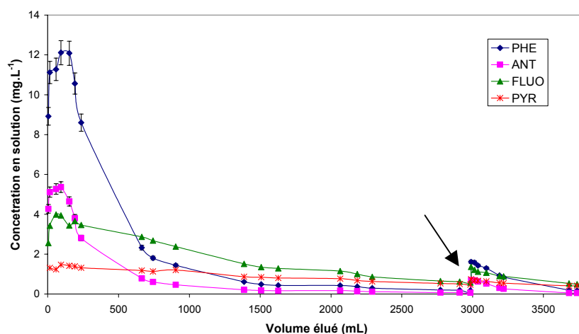
Figure 90 : Concentrations de 4 HAP en sortie de colonne de lixiviation (sol SITA, [HPCD] = 20 g.L -1 , débit = 0,50 mL.min -1 ), barres d'erreurs à \pm 5\% , flèche indiquant un arrêt du débit
