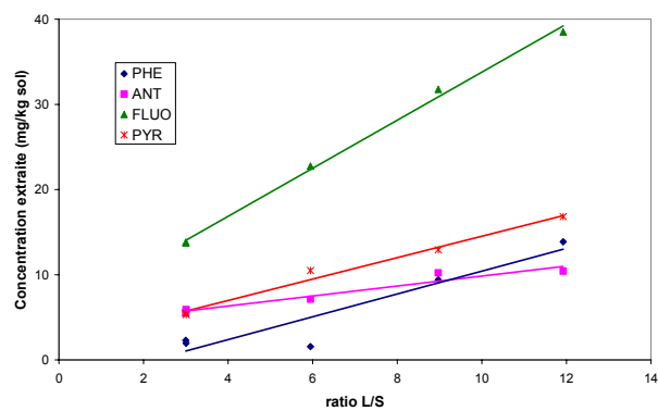
Figure 47 : Influence du ratio L/S sur l'extraction des HAP (sol CNRSP4, [HPCD]=30 g.L -1 , TA)
