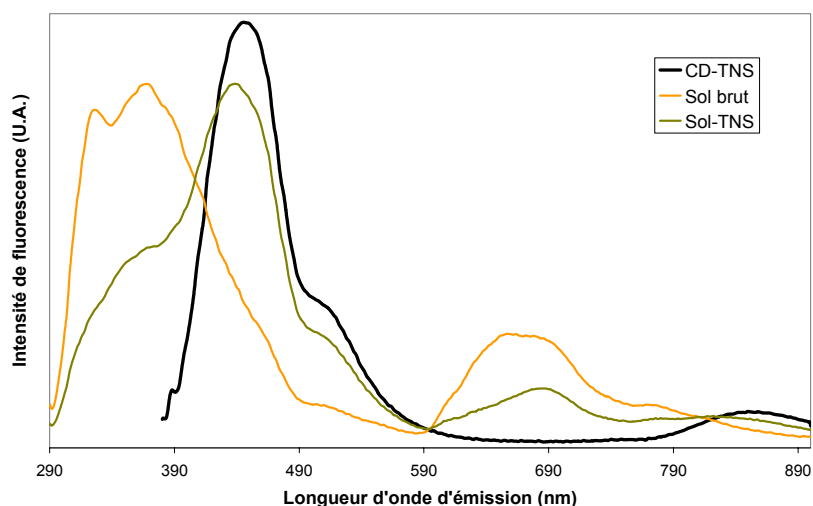
Figure 26 : Superposition des spectres de fluorescence du complexe HPCD-TNS et de lixiviat de sol en présence ou non de TNS
