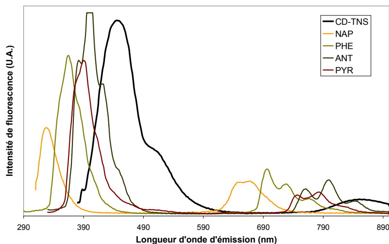
Figure 25 : Superposition des spectres de fluorescence du complexe HPCD-TNS et de 4 HAP ( [HPCD]=5 \text{ g.L}^{-1} , [NAP]=30 \text{ mg.L}^{-1} , [PHE]=40 \text{ mg.L}^{-1} , [ANT]=20 \text{ mg.L}^{-1} , [PYR]=30 \text{ mg.L}^{-1} , dans l'ACN)
