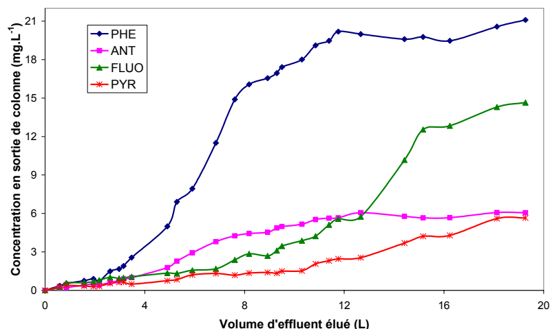
Figure 106 : Concentrations en HAP à la sortie d'une colonne de 15,6 g de résine en fonction du volume élué à un débit de 5 mL.min -1 (concentration entrante en mg.L -1 : [PHE]=22,43 ; [ANT]=6,44 ; [FLUO]=14,65 ; [PYR]=6,07)
