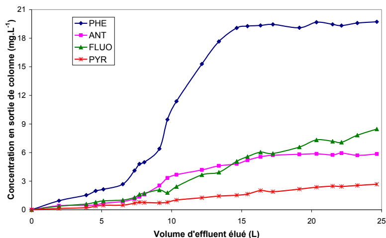
Figure 107 : Concentrations en HAP à la sortie d'une colonne de 15,6 g de résine en fonction du volume élué à un débit de 3 mL.min -1 (concentration entrante en mg.L -1 : [PHE]=22,56 ; [ANT]=6,36 ; [FLUO]=15,73 ; [PYR]=6,11)
