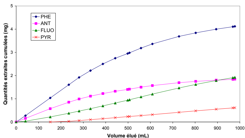
Figure 91 : Quantités cumulées de 4 HAP en sortie de colonne de lixiviation (sol SITA, [HPCD] = 20 \text{ g.L}^{-1} , débit = 1,0 \text{ mL.min}^{-1} )
