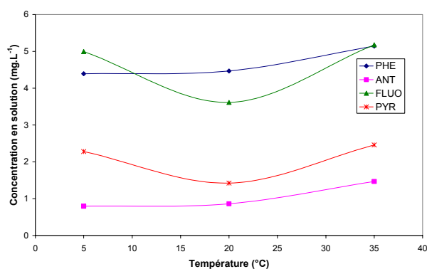
Figure 35 : Influence de la température sur l'extraction des HAP du sol POLDEN ([HPCD]=30 g.L -1 , L/S=3)
