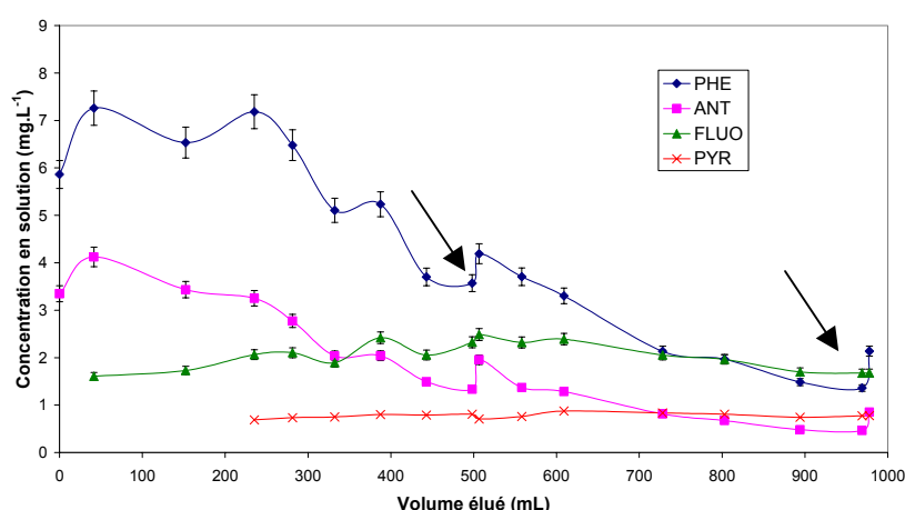
Figure 88 : Concentrations de 4 HAP en sortie de colonne de lixiviation (sol SITA, [HPCD] = 20 g.L -1 , débit = 1,0 mL.min -1 ), barres d'erreurs à \pm 5 %, flèches indiquant les arrêts du débit
