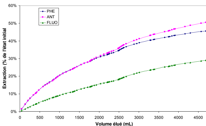
Figure 101 : Abattements de 4 HAP calculé à partir des concentrations de 4 HAP en sortie de colonne de lixiviation (sol CNRSSP 2, [HPCD] = 30 \text{g.L}^{-1} , débit : 0-2475 mL : 0,90-1,00 \text{mL.min}^{-1} , 2475-4690 mL : 0,28 \text{mL.min}^{-1} ).
