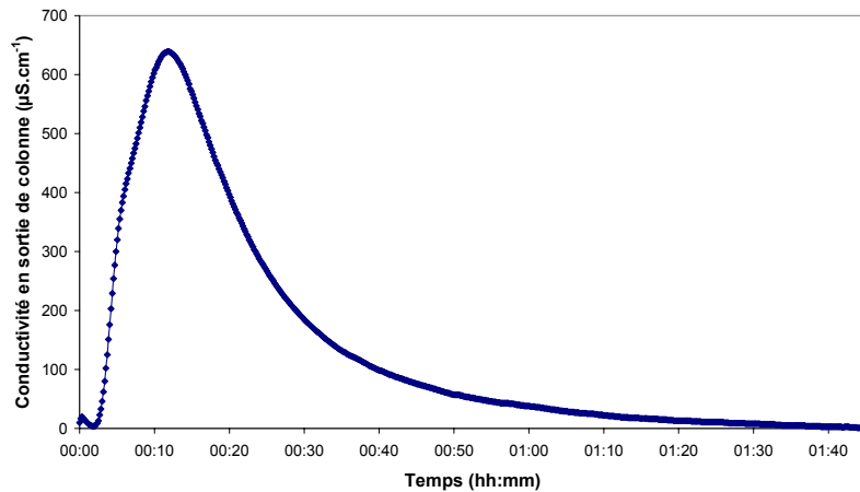
Figure 86 : Caractérisation de l'écoulement dans la colonne de sol CNRSSP 2 par un test de traceur (0,50 mL de [\text{KBr}] = 50 \text{ g.L}^{-1} , débit 1,09 \text{ mL.min}^{-1} )
