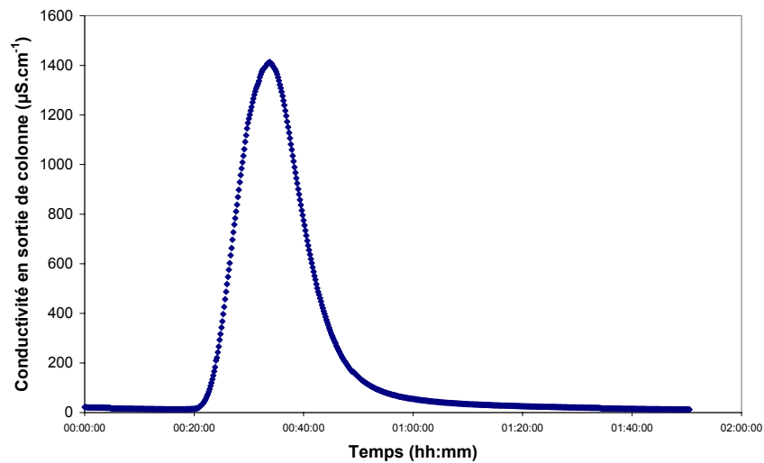
Figure 117 : Elution d'un traceur (injection de 0,25 mL de KBr à 50g.L -1 ) dans une colonne de 25 g de résine, à un débit de 0,55 mL.min -1
