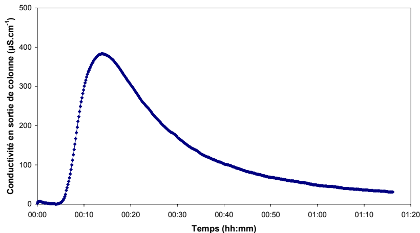
Figure 87 : Caractérisation de l'écoulement dans la colonne de sol CNRSSP 4 par un test de traceur (0,25 mL de [\text{KBr}] = 50 \text{ g.L}^{-1} , débit 1,09 \text{ mL.min}^{-1} )
