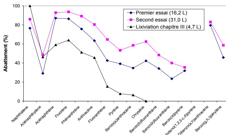
Figure 124 : Représentation de l'abattement des 16 HAP sur le sol CNRSSP2 pour les deux essais de lixiviation et rappel des résultats de l'expérience du chapitre III ([HPCD] = 30 g.L -1 , volume élué en légende)
