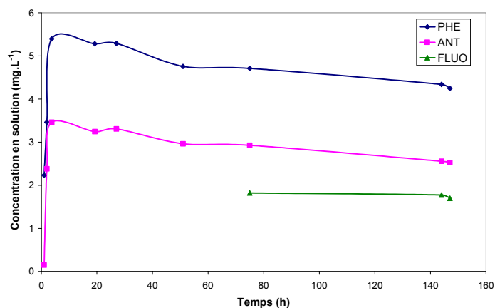
Figure 56 : Evolution temporelle de l'extraction des HAP sur le sol SITA ( [HPCD]=15,1 \text{ g.L}^{-1} , L/S=3 ; 20^{\circ}\text{C} )
