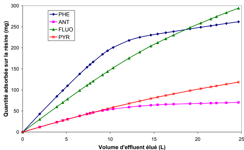
Figure 110 : Quantités cumulées de HAP adsorbés sur une colonne de 15,6 g de résine avec un débit de 3 \text{ mL.min}^{-1} (concentration entrante en \text{mg.L}^{-1} : [\text{PHE}] = 22,56 ; [\text{ANT}] = 6,36 ; [\text{FLUO}] = 15,73 ; [\text{PYR}] = 6,11 , masse totale de HAP adsorbée : 745 mg)
