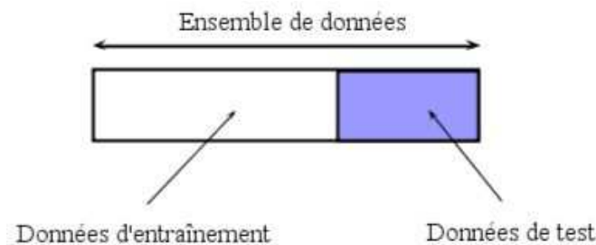
FIG. 7.7 – Méthode Holdout .
