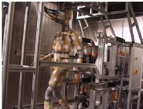
Figure 2.6 : SAM, mannequin articulé thermique (Photo Empa)
