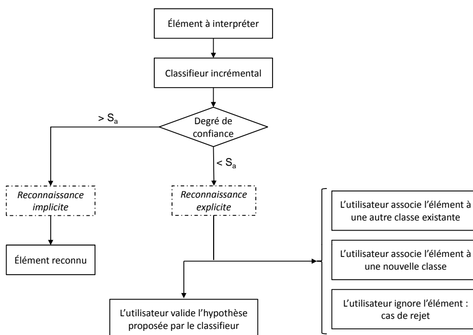
Figure 5.26 – Étape d'interaction
