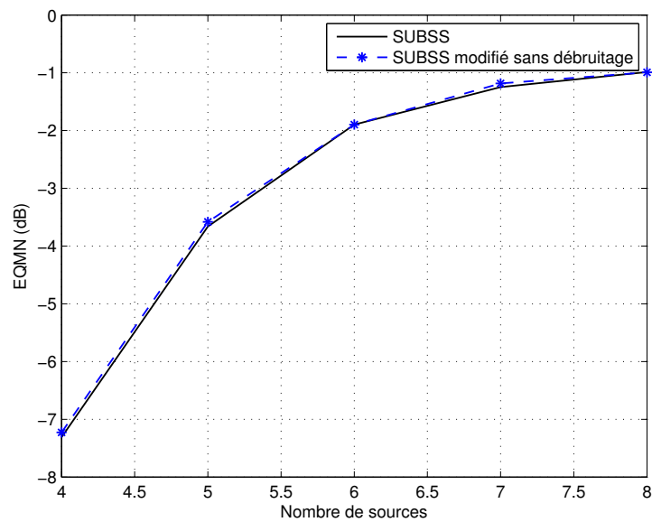
Figure 4.5 — EQMN en fonction du nombre de sources : Comparaison des performances de l’algorithme SUBSS standard et de l’algorithme SUBSS modifié sans débruitage.
