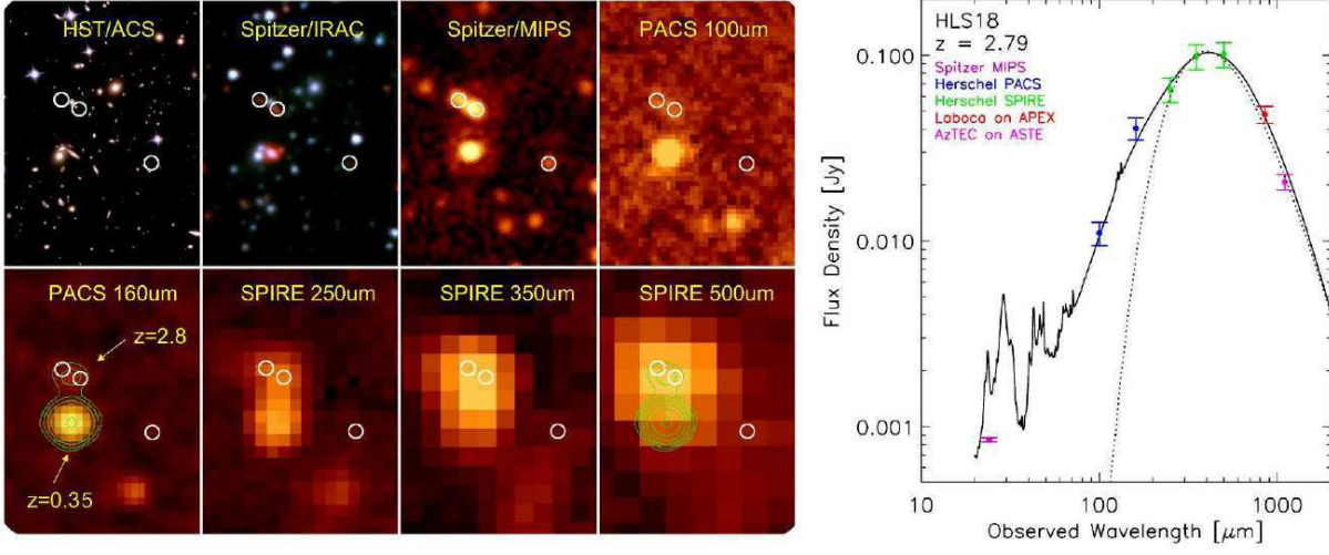
FIGURE 3.8 – Détection dans les bandes Herschel (PACS/SPIRE) et mesure de la SED des poussières dans une galaxie à z = 2.8 amplifiée par l’amas du ‘Boulet’. Cette source amplifiée à z \sim 3 a une luminosité intrinsèque de \sim 3 \cdot 10^{11} L_{\odot} .
