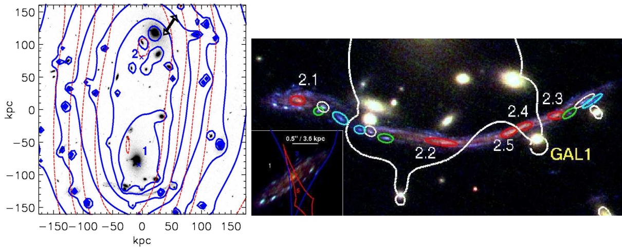
FIGURE 1.4 – A gauche : isocontours de la carte de masse reconstruite pour l’amas Abell 370 (en bleu), montrant son caractère bimodal également visible dans les observations en rayons X (contours rouges). A droite : interprétation de l’arc géant à z = 0.7 en localisant les régions identiques multipliées par effet de lentille (ellipses colorées) et la ligne critique correspondante (en blanc). La morphologie de la source d’origine est visible en bas à gauche comme étant une spirale. D’après Richard et al. (2010a).
