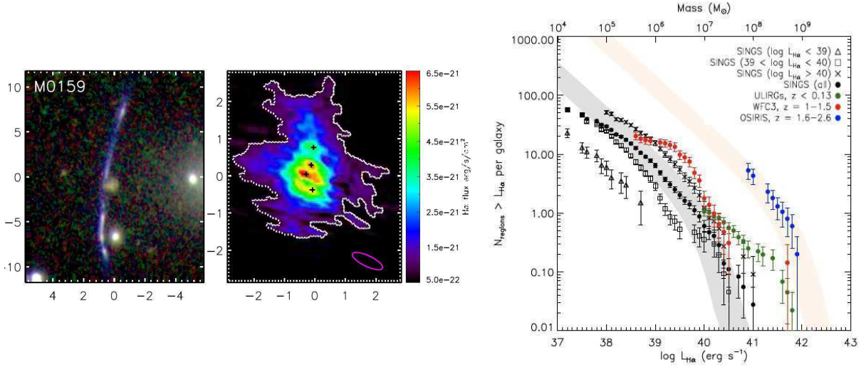
FIGURE 2.9 – A gauche : exemple d’arc à z = 1 observé par Hubble dans un filtre en bande étroite, et la reconstruction dans le plan source de l’excès de flux de ce filtre en bande étroite correspondant à l’émission \text{H}\alpha , avec la détection de plusieurs régions de formation stellaire. A droite : fonction de luminosité des régions de formation stellaire identifiées pour cet échantillon, celui de Jones et al. (2010b) et d’autres échantillons locaux ou distants. Les résultats sont comparables aux modèles de Hopkins et al. (2011) concernant la distribution de nuages moléculaires géants dans l’Univers local (en gris) et à grand décalage spectral (en rose).
