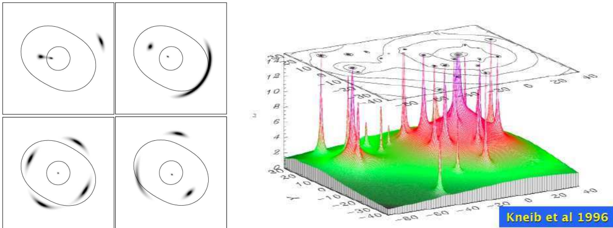
FIGURE 1.1 – A gauche : différentes configurations possibles pour des images multiples. Dans l’ordre de lecture : un arc radial et sa contre-image, un arc géant, une croix d’Einstein, une configuration avec un arc tangentiel en ‘fold’ (d’après Kneib 1993). A droite : Représentation de la distribution de masse dans un amas : on distingue un profil général à grande échelle et de multiples pics locaux correspondant aux sous-structures, et localisées à la position des pics de lumière des galaxies individuelles de l’amas.
