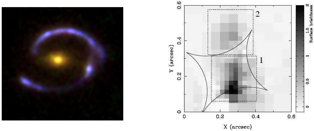
FIGURE 2.2 – A gauche, image à haute résolution de l’œil cosmique obtenue par le télescope Hubble en combinant les filtres visible (caméras ACS et WFPC2) et proche-infrarouge (caméra NICMOS). A droite, reconstruction de la source d’origine en corrigeant de l’effet de lentille (Dye et al., 2007) : on distingue deux composantes (marquées par 1 et 2) avec une amplification différente.
