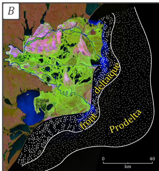
Figure 24 : A - Caractérisation générale du delta du Danube et délimitation de la plaine deltaïque. B - Limites du front deltaïque et du prodelta, lignes retracées d'après Panin (2003). C - Éléments de la géomorphométrie plane.
