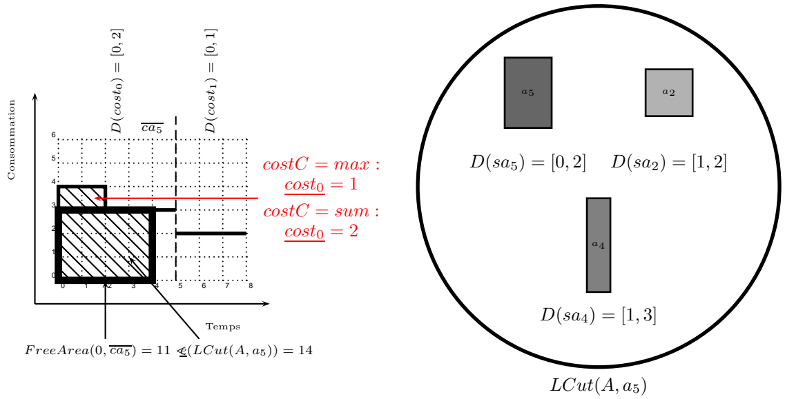
FIGURE 5.13 – Un problème cumulatif relaxé avec trois activités a_2 , a_4 et a_5 telles que D(sa_2) = [1, 2] , D(sa_4) = [1, 3] , D(sa_5) = [0, 2] , D(ca_2) = [3, 4] , D(ca_4) = [2, 4] , D(ca_5) = [2, 4] , da_2 = 2 , da_4 = 1 , da_5 = 2 , ra_2 = 2 , ra_4 = 4 , ra_5 = 3 , et deux intervalles utilisateur. Nous modifions légèrement l'exemple de la Figure 5.11, tel que : p_0 : [0, 5[ et p_1 = [5, 8[ . Nous avons : [0, \overline{ca_5}] \subseteq p_0 et \underline{e}(LCut(A, a_5)) = 14 > FreeArea(0, \overline{ca_5}) = 12 , Alors a_5 définit une borne inférieure sur la variable objectif : LB^V(a_5) , mais également sur la variable de coût cost_0 , telle que \underline{cost_0} = LB^V(a_5) . Si costC = max , \underline{cost_0} = 1 , si costC = sum , \underline{cost_0} = 2 .
