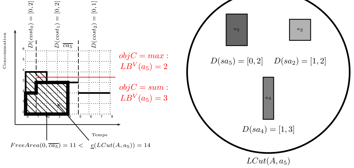
FIGURE 5.12 – Un problème cumulatif relaxé de la Figure 5.11 avec costC = sum . On a \underline{e}(LCut(A, a_5)) = 14 > FreeArea(0, \overline{ca_5}) = 11 , alors a_5 définit une borne inférieure sur la variable objectif. Ici, \mathcal{P} = \{p_0, p_1\} . Si objC = max , LB^V(a_5) = \left\lfloor \frac{\underline{e}(LCut(A, a_5)) - FreeArea(sp_0, \overline{ca_5})}{|\mathcal{P}|} \right\rfloor = 2 et si objC = sum , LB^V(a_5) = \underline{e}(LCut(A, a_5)) - FreeArea(sp_0, \overline{ca_5}) = 3
