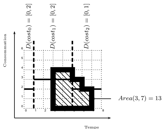
FIGURE 5.6 – Aire disponible entre deux points de temps 3 et 7, avec costC = sum . Dans ce cas, Area(3, 7) = 13 .
