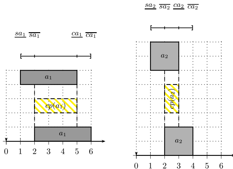
FIGURE 2.5 – Les activités a_1 et a_2 positionnées en leurs deux positions extrêmes, et leur partie obligatoire cp(a_1) et cp(a_2) .
