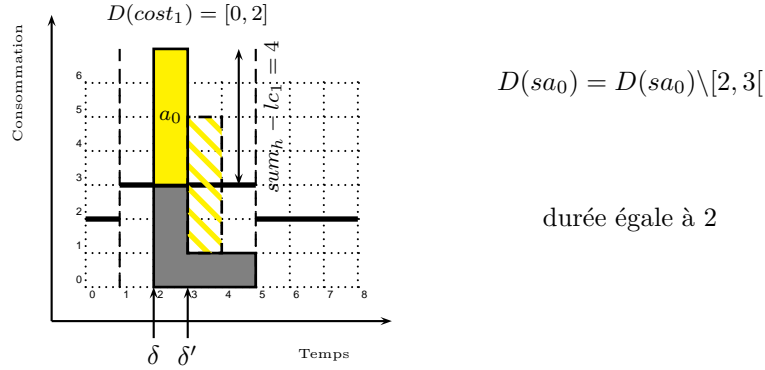
FIGURE 5.3 – Un pas de l'algorithme de Sweep pour la SOFTCUMULATIVE, avec costC = max . L'activité a_0 , représenté en jaune, est telle que D(sa_0) = [2, 6] , ra_0 = 4 et da_0 = 2 . En \delta' = 3 , il y a un événement de profil, nous considérons alors la hauteur de profil sum_h = 3 . Ici, costC = max . Nous ajoutons la consommation de ressource de a_0 : sum_h + ra_0 = 7 . Cela est strictement supérieur à la capacité locale plus le coût maximal. Alors on peut filtrer la date de début de a_0 : D(sa_0) = D(sa_0) \setminus [2, 3[ .
