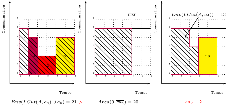
FIGURE 2.12 – Un exemple de mise à jour du début au plus tôt de l'activité a_0 , grâce à la relation de précedence \{a_2, a_4\} = LCut(A, a_4) \prec a_0 .
