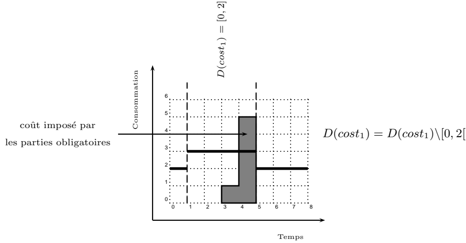
FIGURE 5.10 – Le polygone plein représente le profil cumulatif des parties obligatoires d'un problème SOFTCUMULATIVE. Dans cet exemple, pour costC = max , ou costC = sum , avant le filtrage, D(cost_1) = [0, 2] . En t = 3 , sum_h = 5 , lc_1 = 3 : sum_h - lc_1 > \underline{cost}_1 , alors nous filtrons D(cost_1) tel que D(cost_1) = D(cost_1) \setminus [0, 2[ .
