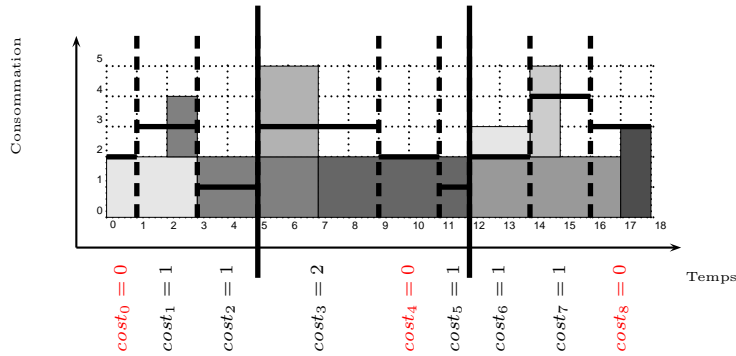
FIGURE 4.4 – Une solution satisfaisant des contraintes de cardinalité additionnelles sur la partition \{(cost_0, cost_1, cost_2), (cost_3, cost_4, cost_5), (cost_6, cost_7, cost_8)\} avec cost_C = \max : au moins un coût égal à 0 dans chaque classe de la partition : elles sont colorées en rouge. Elle satisfait aussi la contrainte SMOOTH(1, 1, Cost) . Le nombre de fois où la valeur absolue de la différence entre deux variables de coût consécutives est strictement supérieure à 1 est égale à 1 ( |cost_4 - cost_3| = 2 ). Enfin, elle satisfait également la contrainte FOCUS(I[Cost], 2, 3, 0) : nous avons deux séquences de variables de coût à valeur strictement positive, de longueur 3.
