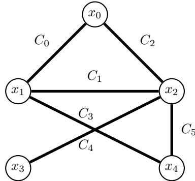
FIGURE 1.1 – Un réseau de contraintes binaires comportant 5 variables \{x_0, x_1, \dots, x_4\} et 6 contraintes binaires \{C_0, C_1, \dots, C_5\}
