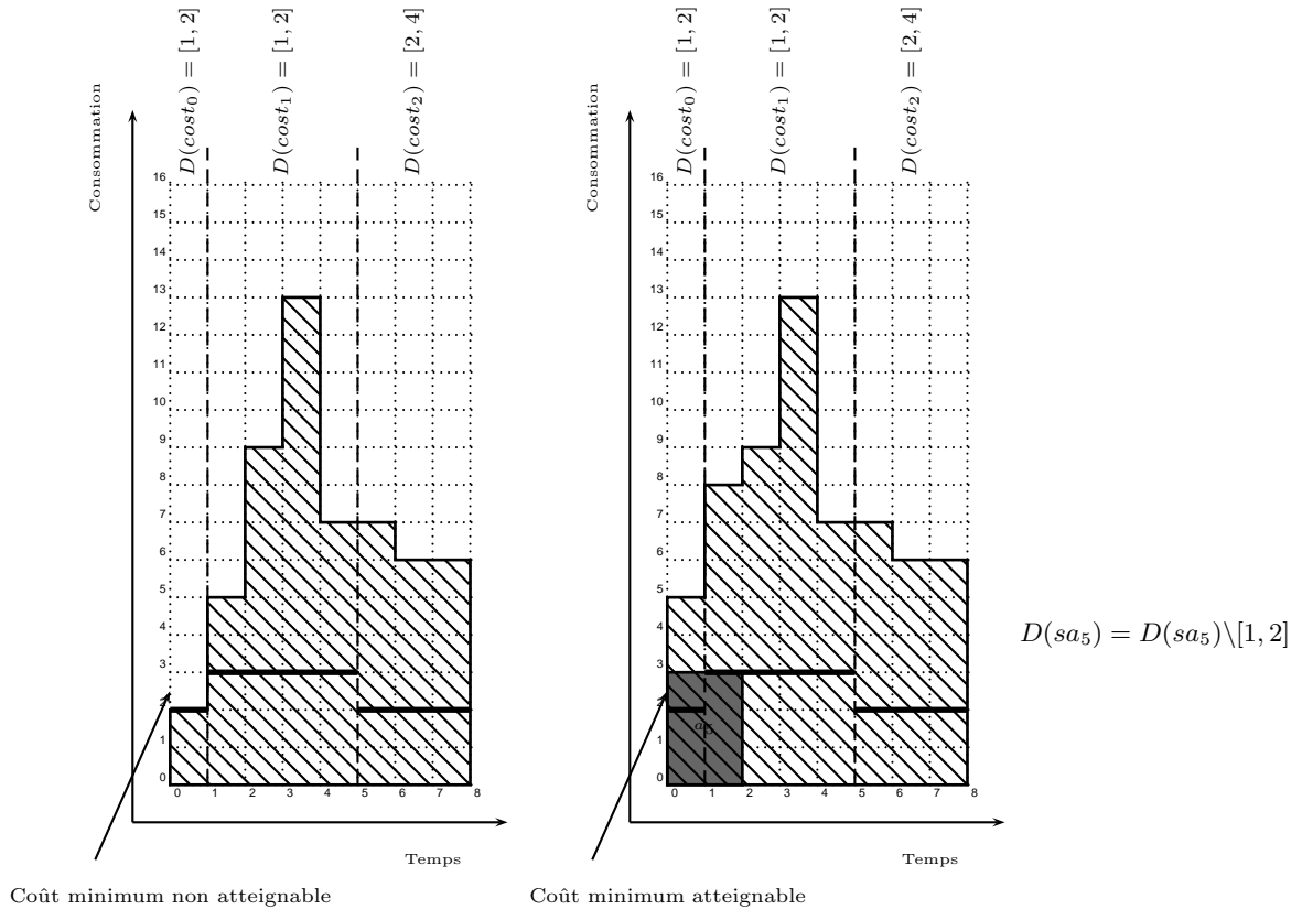
FIGURE 5.17 – Les différents pas de la procédure de filtrage de l'activité a_5 de la Figure 5.16, avec costC = max . Nous rappelons que D(sa_5) = [0, 2] . La partie enveloppante de l'activité a_5 à filtrer est retirée du profil enveloppant. Sur la première figure, il apparaît que le coût minimal dans le premier intervalle cost_0 = 1 ne peut être atteint. Nous mettons alors à jour le début de a_5 pour s'assurer que, si a_5 débute en sa_i ou \bar{sa}_i , alors, en chaque point de temps, le profil enveloppant peut atteindre la valeur minimale du domaine des coûts locaux. De ce fait, D(sa_5) = D(sa_5) \setminus [1, 2] .
