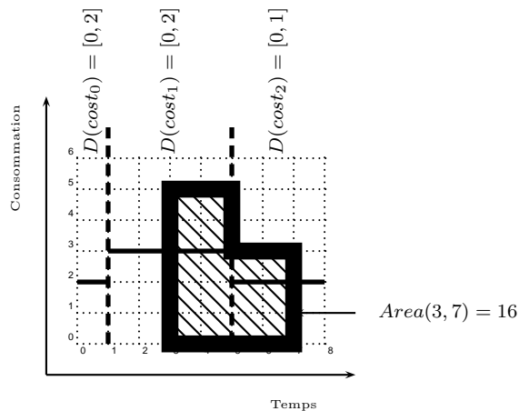
FIGURE 5.5 – Aire disponible entre deux points de temps 3 et 7, avec costC = max . Dans ce cas, Area(3, 7) = 16 .
