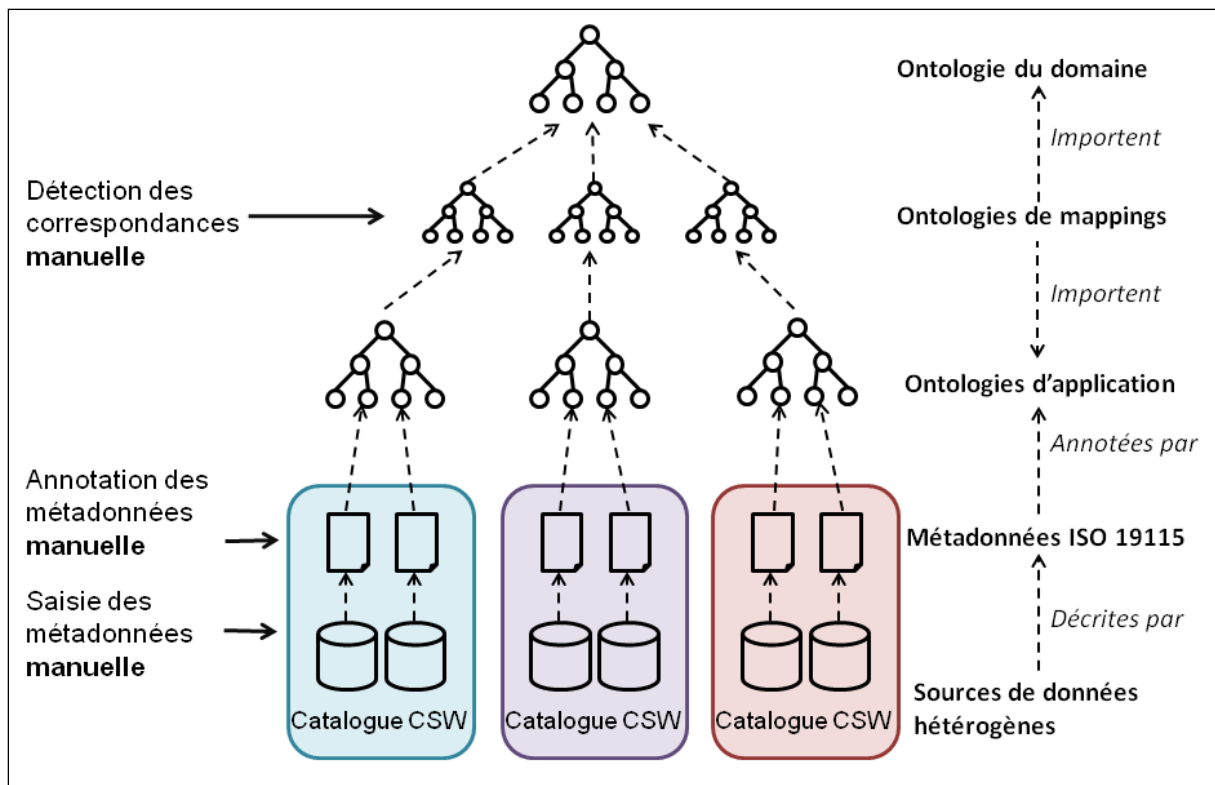
Figure 8: Approche proposée par (Lassoued et al., 2008) pour la découverte des données: identification des étapes automatiques et manuelles
