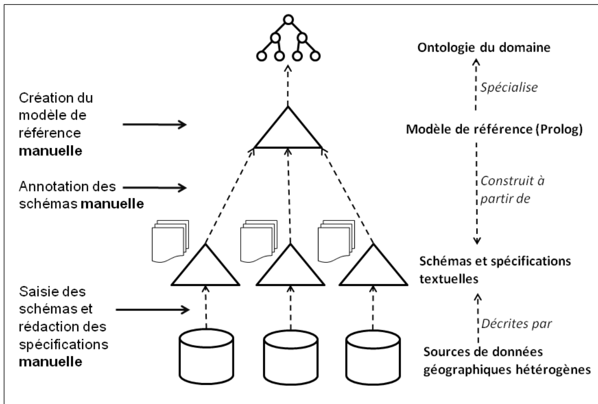
Figure 20: Approche proposée par Uitermark (2001): identification des étapes d'annotation automatiques et manuelles
