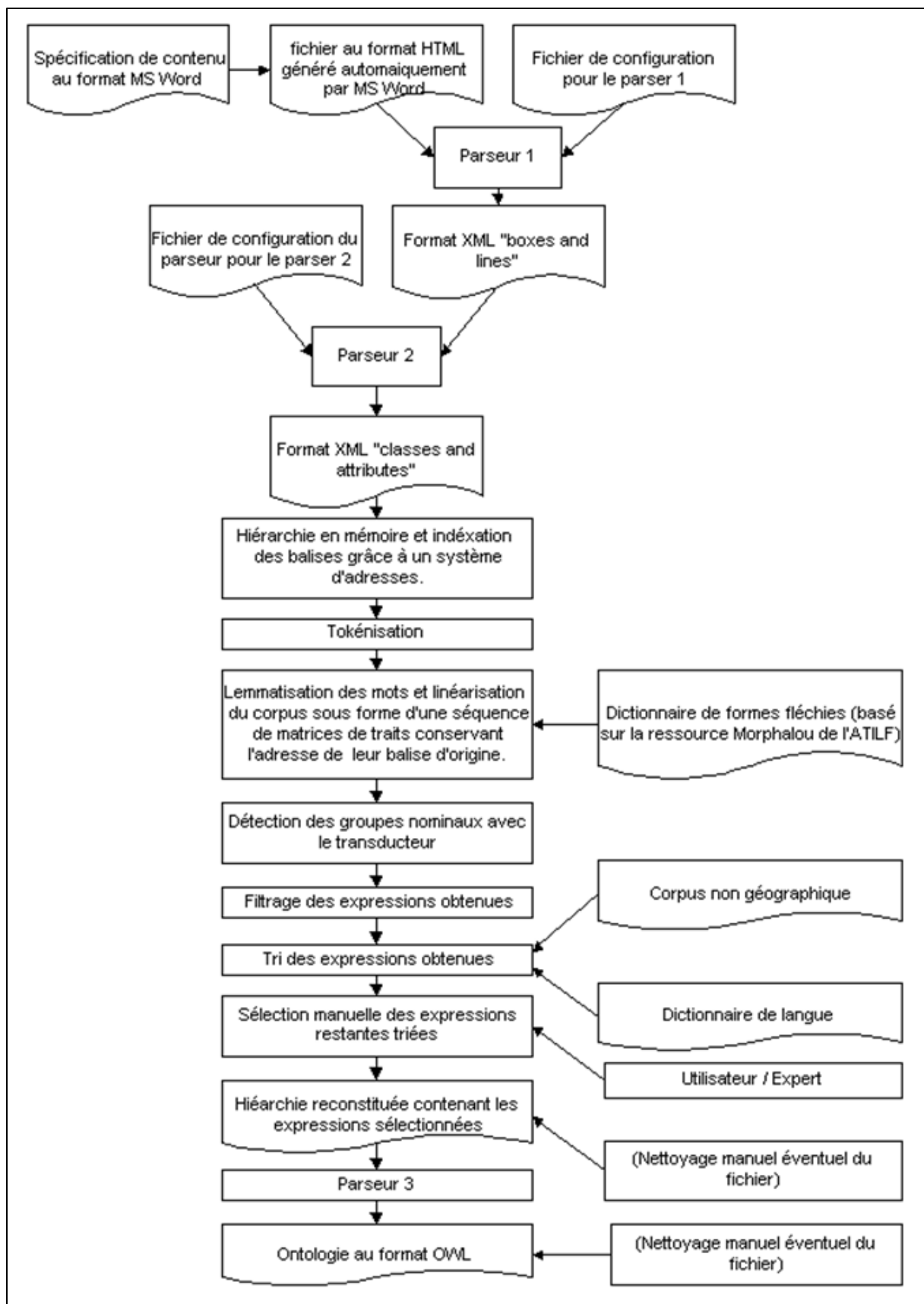
Figure 27: Enchaînement des traitements mis en œuvre pour la constitution d'une ontologie de concepts topographiques à partir des spécifications de base de données topographiques
