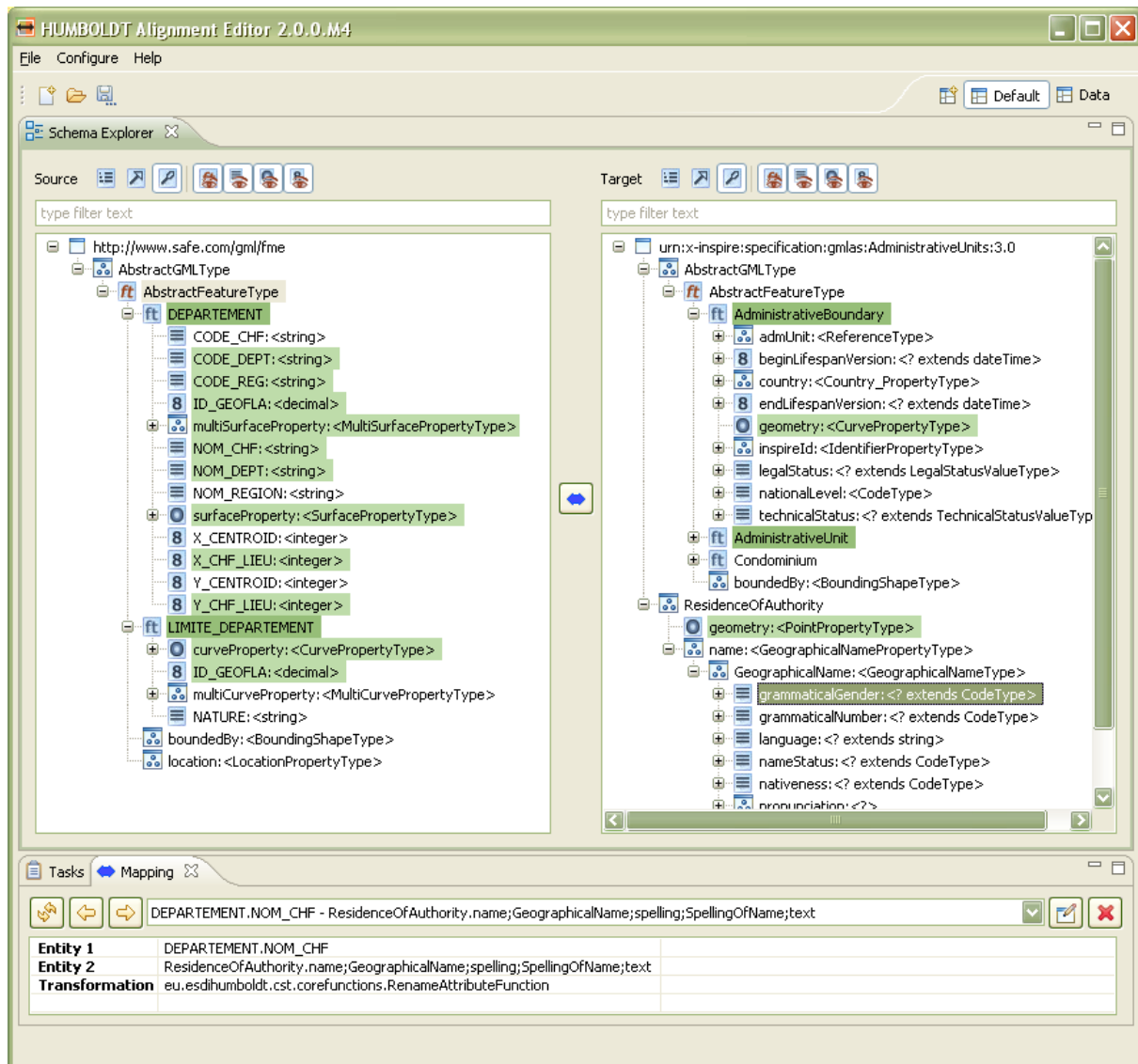
Figure 17: Interface d'appariement manuel de schémas fournie par HALE : appariement du schéma conceptuel de données GEOFLA© avec le schéma INSPIRE « Administrative Units »
