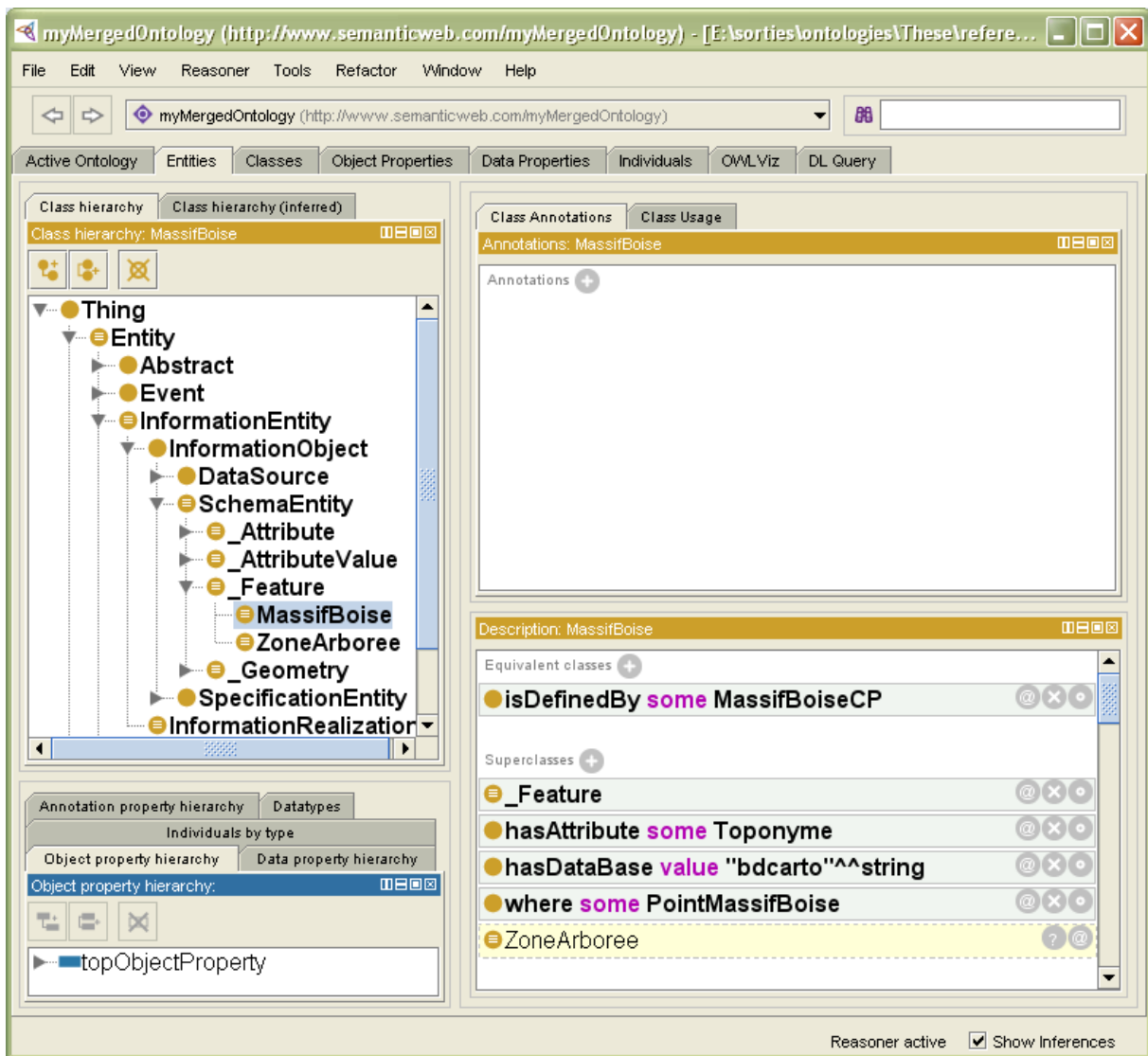
Figure 54: Utilisation d'un système de raisonnement pour ontologies pour l'appariement des classes Massif Boisé et ZoneArborée (Visualisation sous Protégé)
