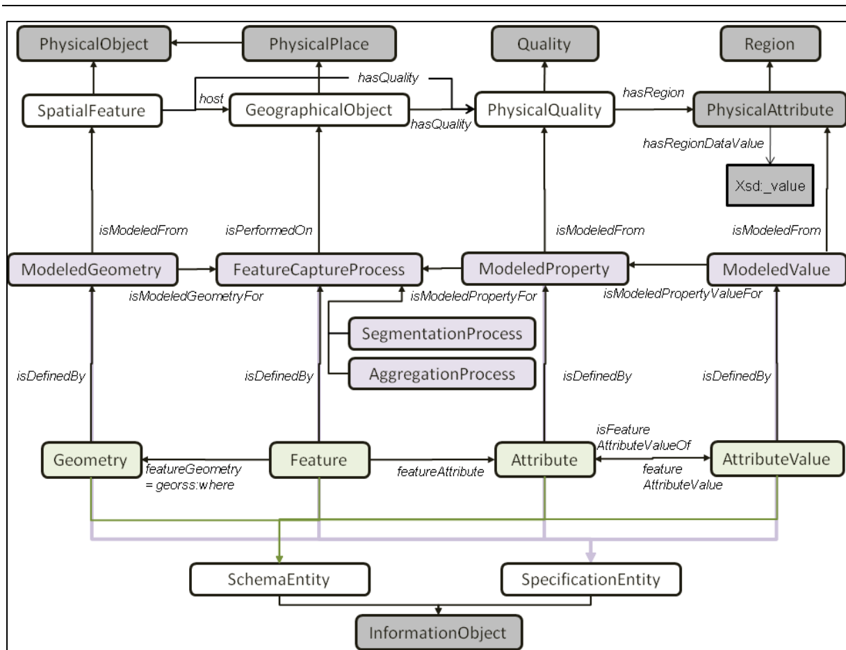
Figure 50: Modèle global pour la représentation des spécifications
