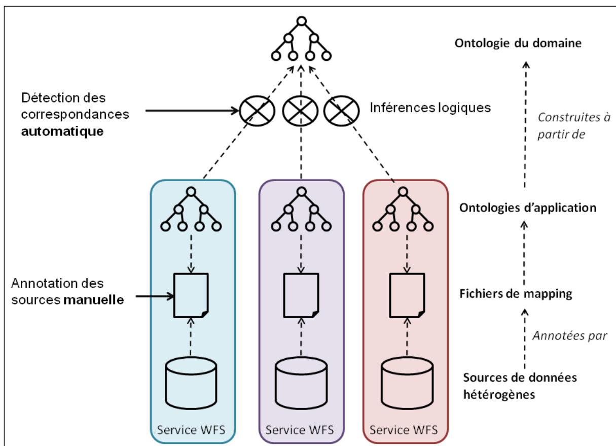
Figure 11: Approche proposée par (Lutz et al., 2006) pour la découverte des données: identification des étapes automatiques et manuelles
