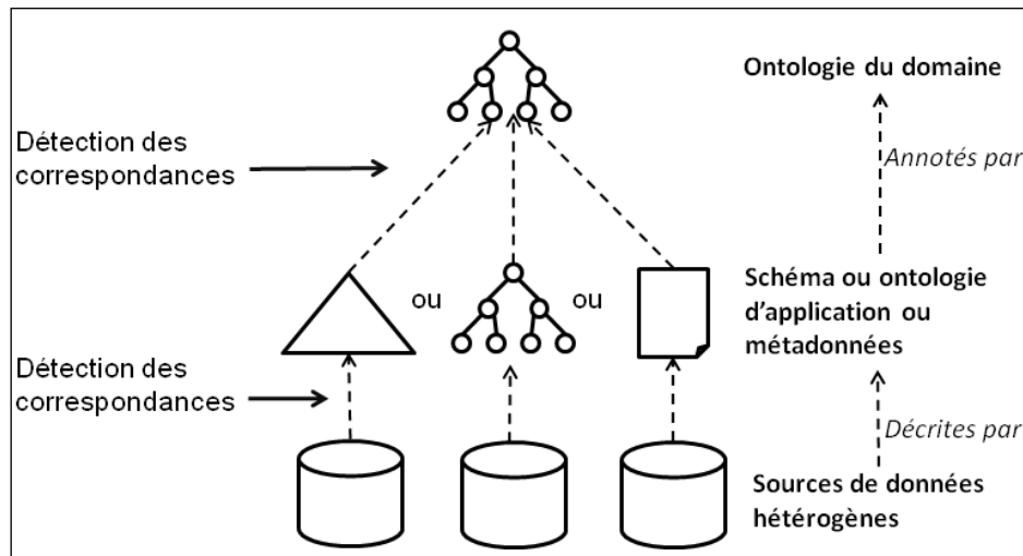
Figure 16: Architecture globale des applications décrites dans ce chapitre
