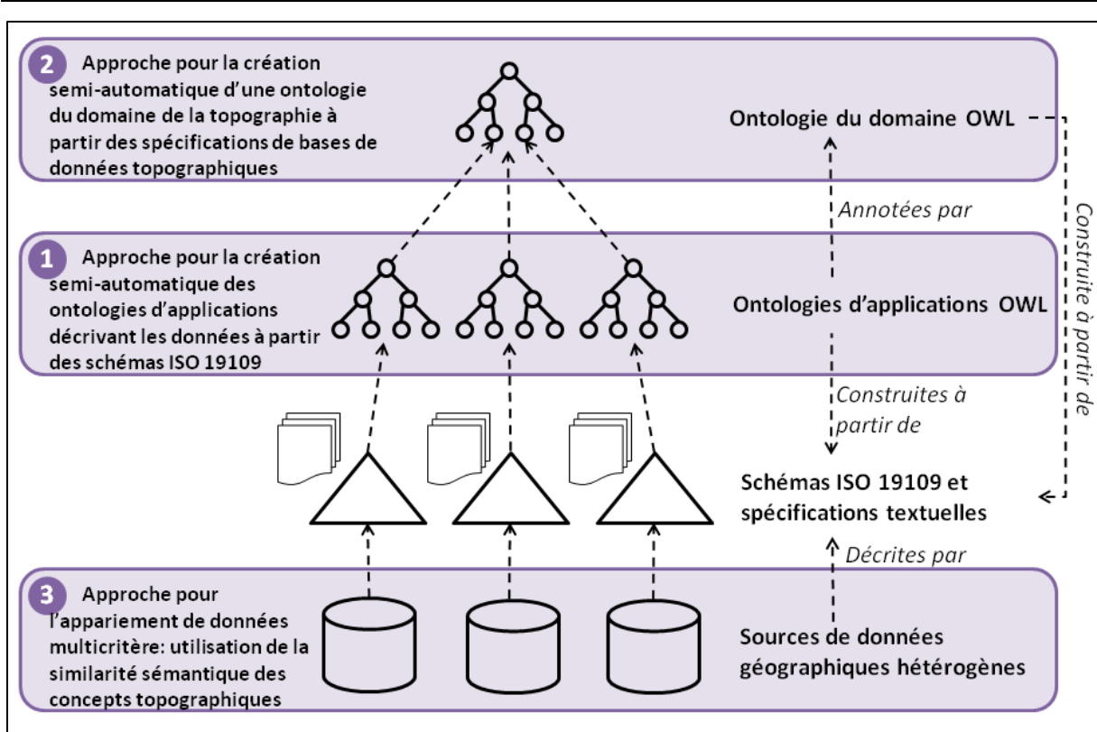
Figure 65: Principales contributions pour l'approche d'appariement fondée sur les valeurs d'attributs et une ontologie de support
