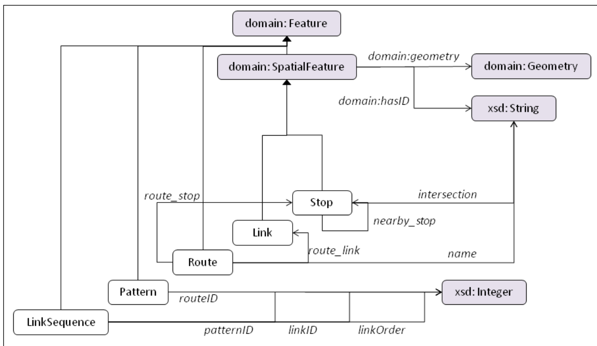
Figure 9: Ontologies utilisées par (Zhao et al, 2008)
