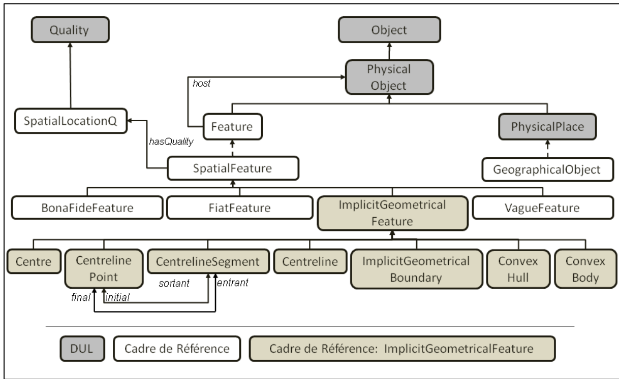
Figure 48: Cadre de référence sémantique pour la représentation des éléments géométriques implicites caractérisant la forme des entités géographiques
