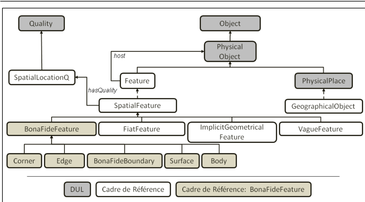
Figure 46: Cadre de référence sémantique pour la représentation des éléments caractérisant la forme des entités géographiques de type Bona Fide
