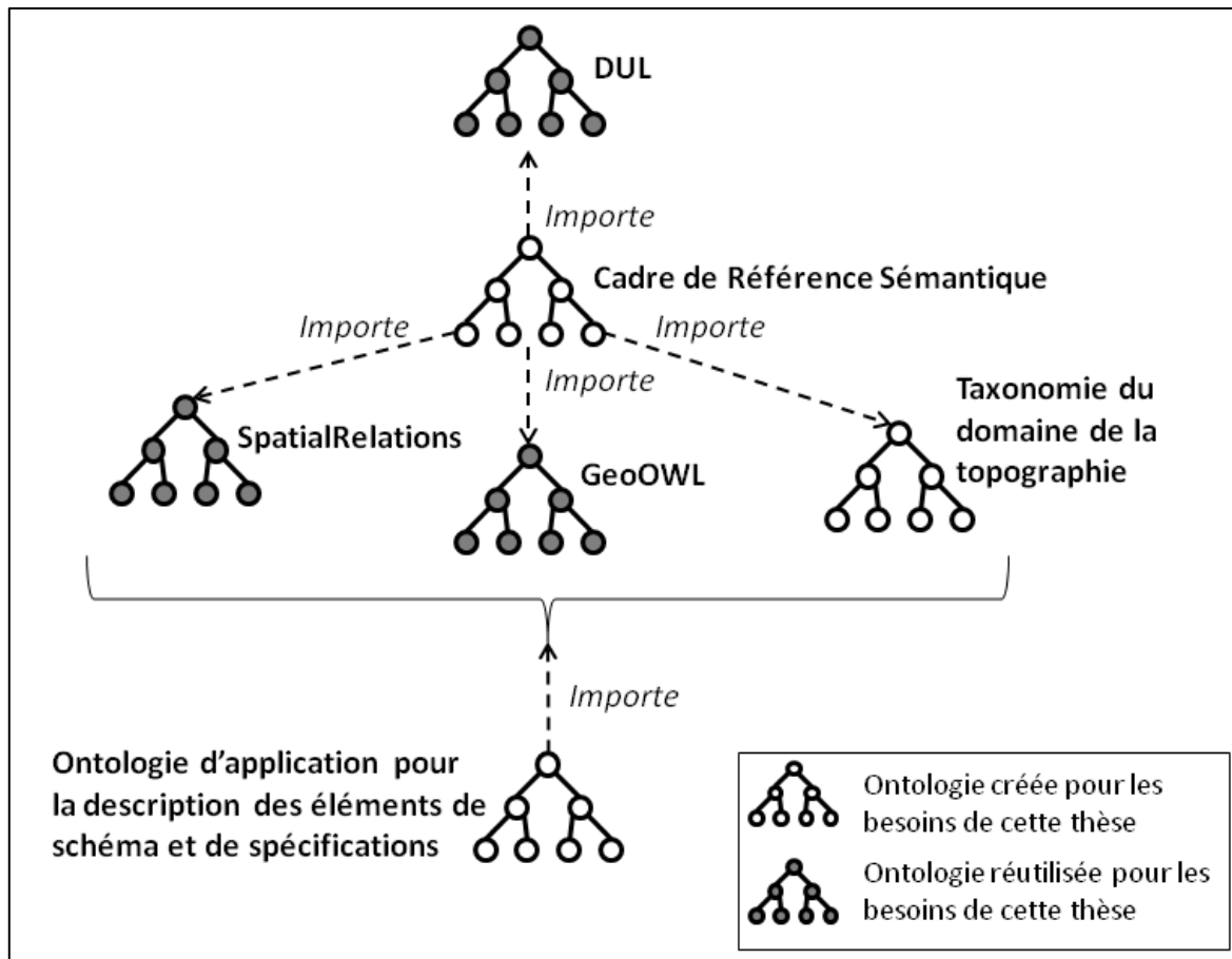
Figure 64: Articulation des différentes ontologies mises en œuvre dans l'approche fondée sur les spécifications (partie 4.3)
