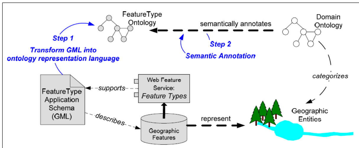
Figure 13: Modèle global pour l'annotation de bases de données géographiques extrait de (Klien, 2008)
