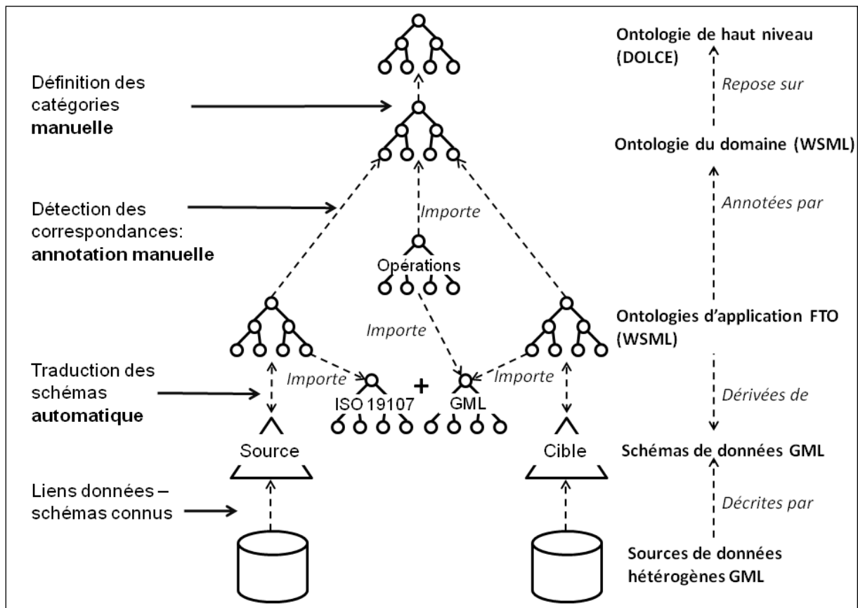
Figure 18: Approche proposée par Schade (2010): identification des étapes d'annotation automatiques et manuelles
