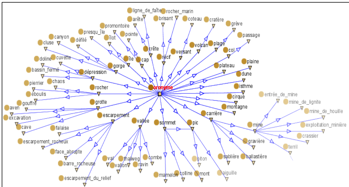
Figure 29: Taxonomie des éléments remarquables du relief obtenue par analyse automatique des spécifications de la BDTOPO© Pays 1.2 (visualisation sous Protégé)
