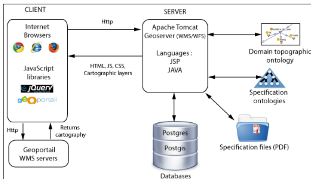
Figure 56: Implémentation de l'application de découverte de bases de données topographiques hétérogènes
