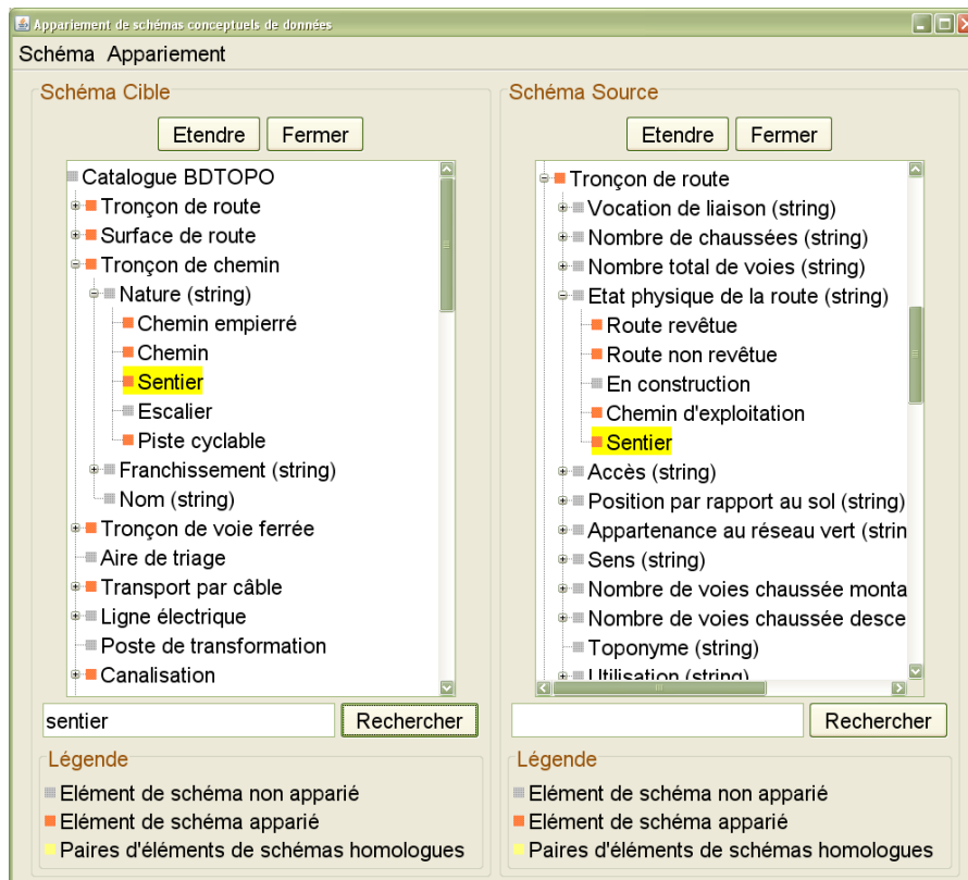
Figure 33: Apports de l'utilisation des « concepts cachés » dans le processus d'appariement: appariement des valeurs d'attributs Sentier
