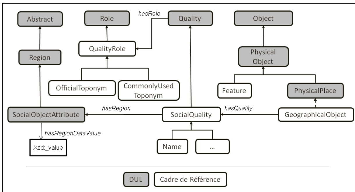
Figure 43: Cadre de référence sémantique pour la représentation des propriétés sociales des catégories d'entités topographiques
