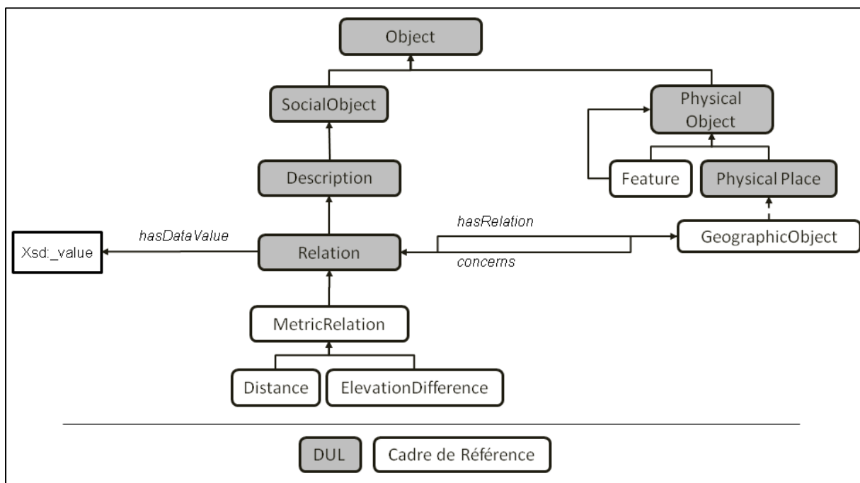
Figure 44: Cadre de référence sémantique pour la représentation des relations spatiales entre entités topographiques
