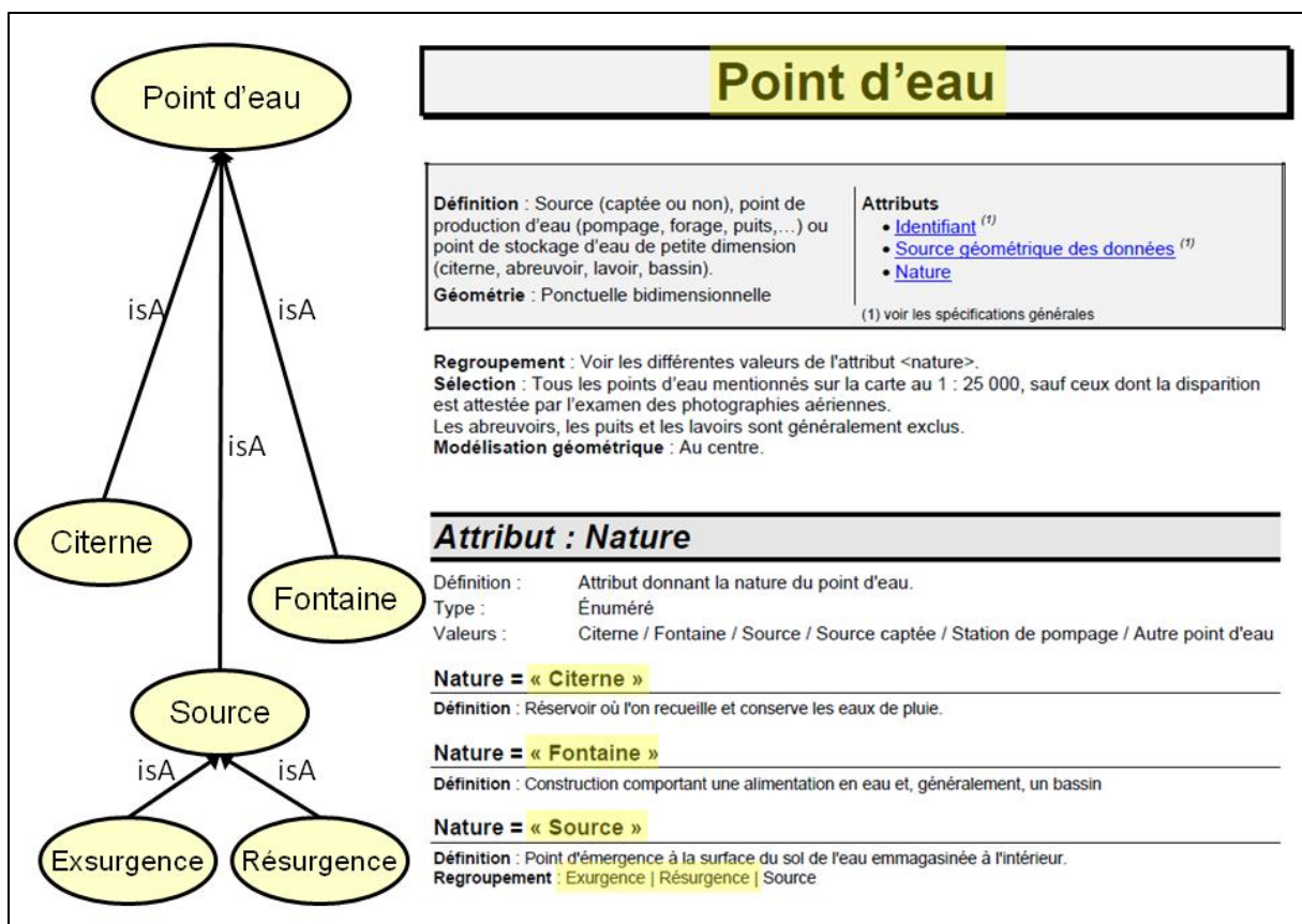
Figure 26: Approche proposée pour la définition et la structuration des connaissances au sein de l'ontologie du domaine de la topographie
