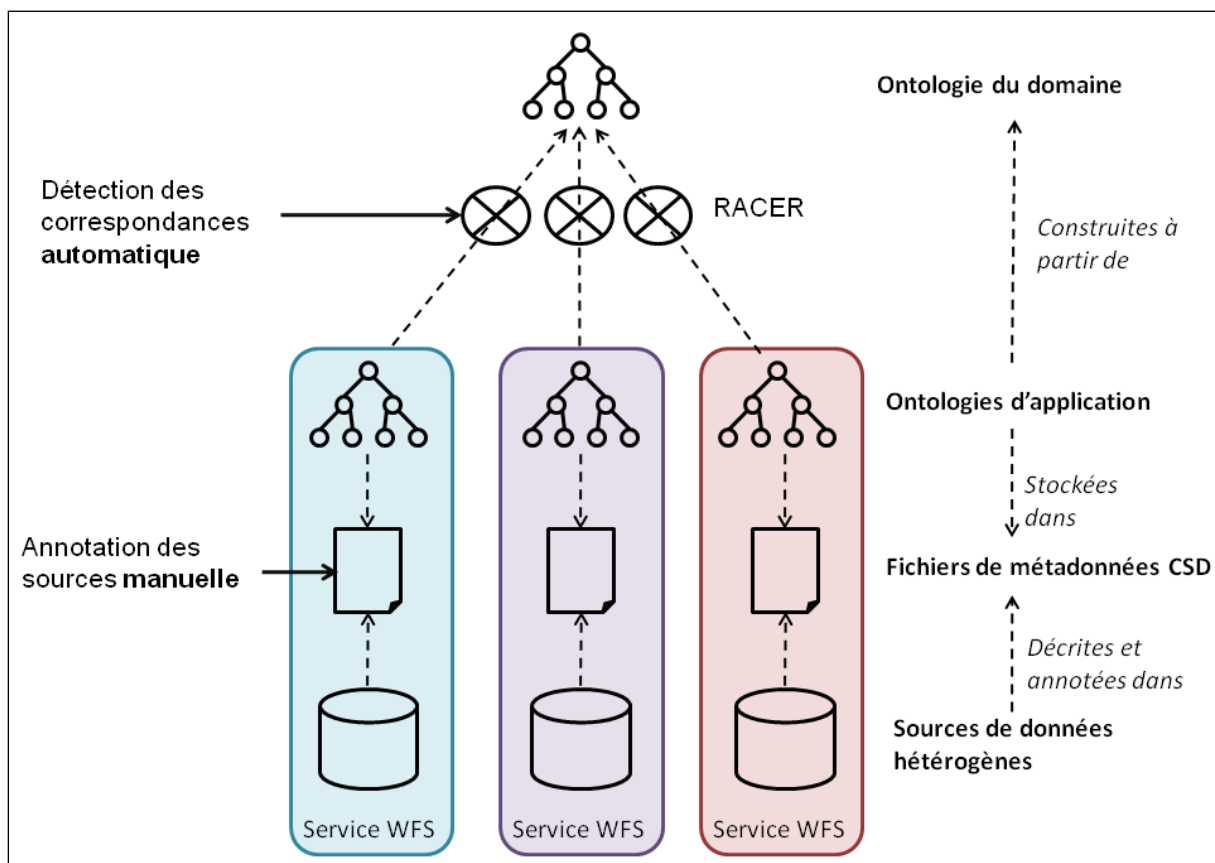
Figure 4: Approche proposée par (Paul et Ghosh, 2006) pour la découverte et l'accès aux données: identification des étapes d'annotation automatiques et manuelles
