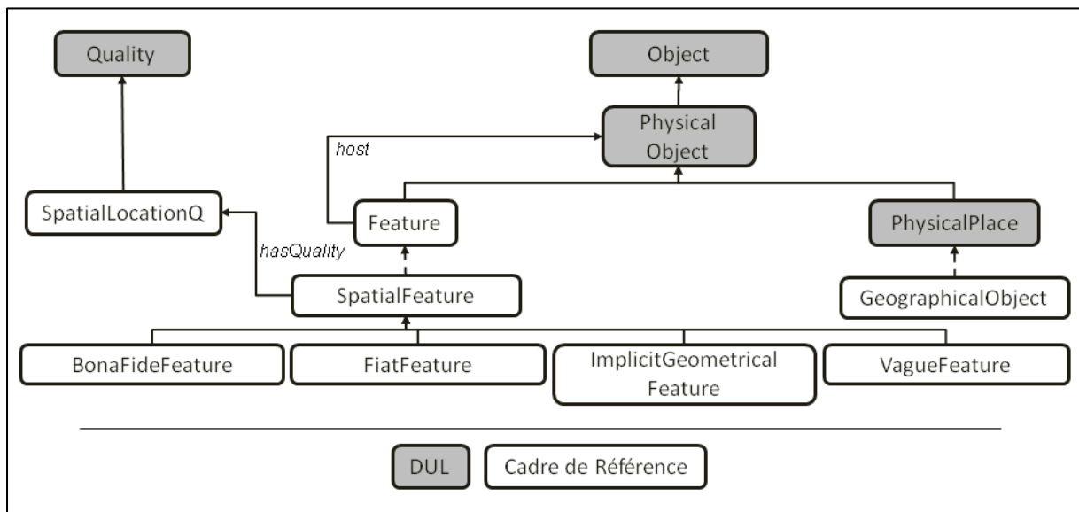
Figure 45: Cadre de référence sémantique pour la représentation des éléments caractérisant la forme des entités géographiques
