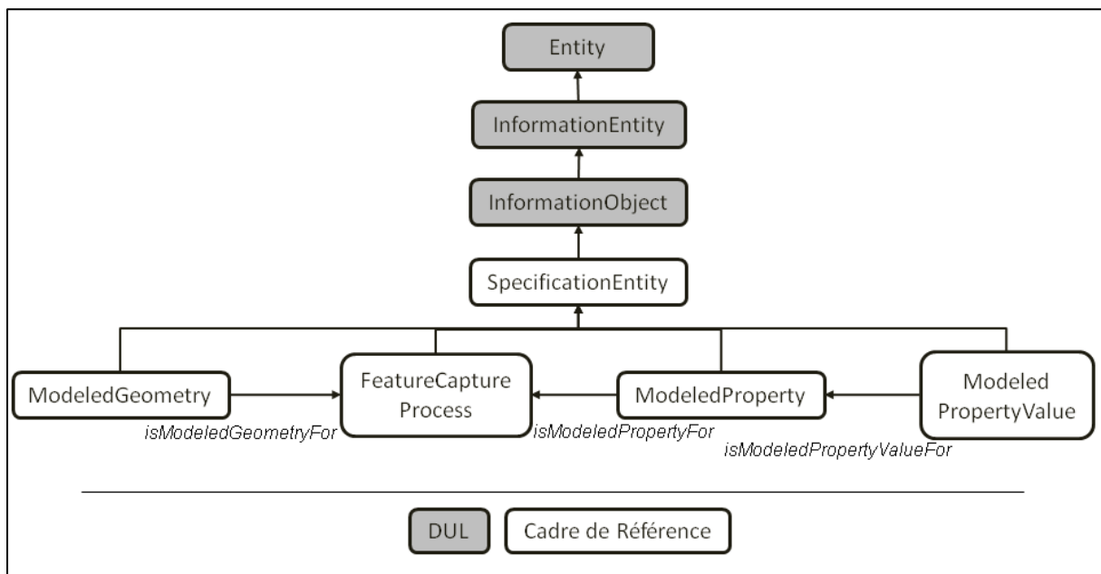
Figure 40: Partie du cadre de référence sémantique destinée à la représentation des éléments de spécifications de bases de données topographiques – Classes principales
