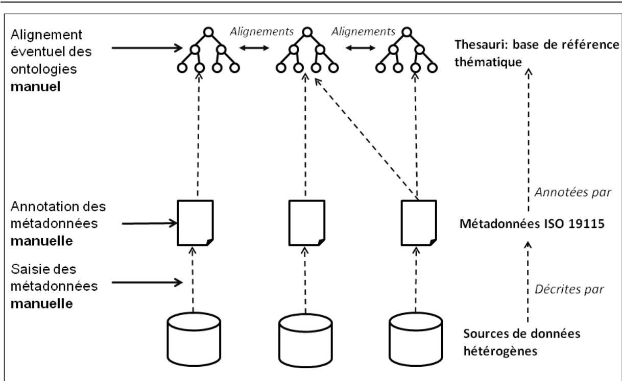
Figure 6: Approche proposée par (Desconnets et al., 2007) pour la découverte des données: identification des étapes d'annotation automatiques et manuelles
