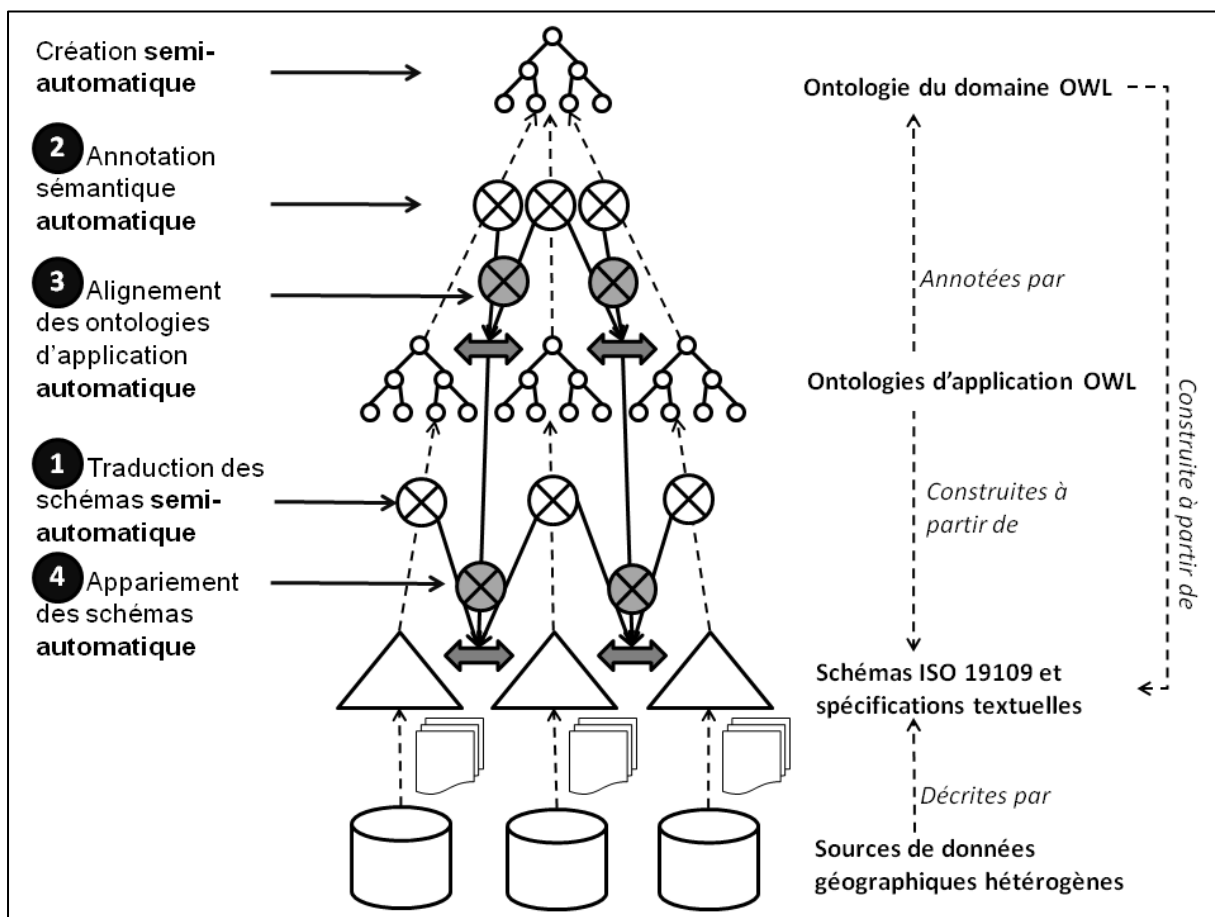
Figure 24: Processus global d'appariement de schémas de bases de données géographiques fondé sur des valeurs d'attributs et une ontologie de support
