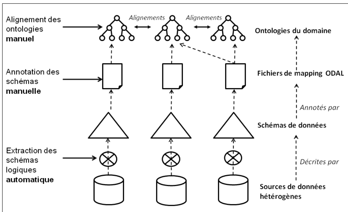
Figure 5: Approche proposée par (Nambiar et al., 2006) pour la découverte et l'accès aux données: identification des étapes d'annotation automatiques et manuelles
