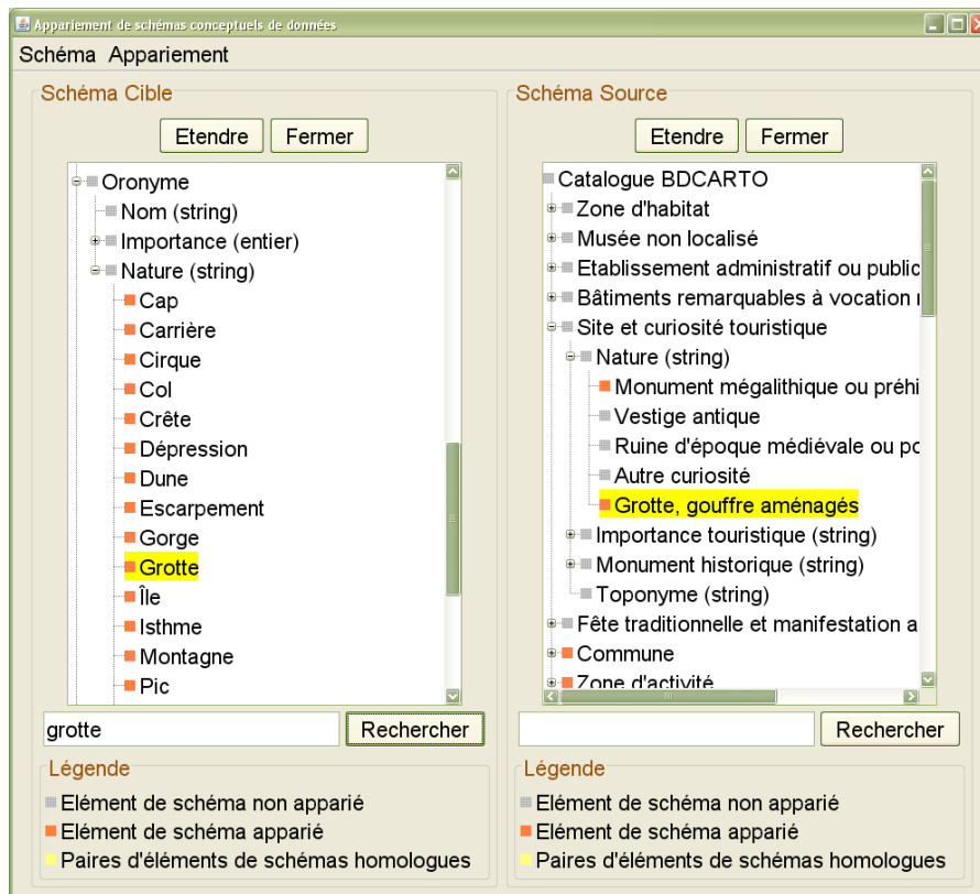
Figure 34: Apports de l'utilisation des « concepts cachés » dans le processus d'appariement: appariement des valeurs d'attributs Grotte
