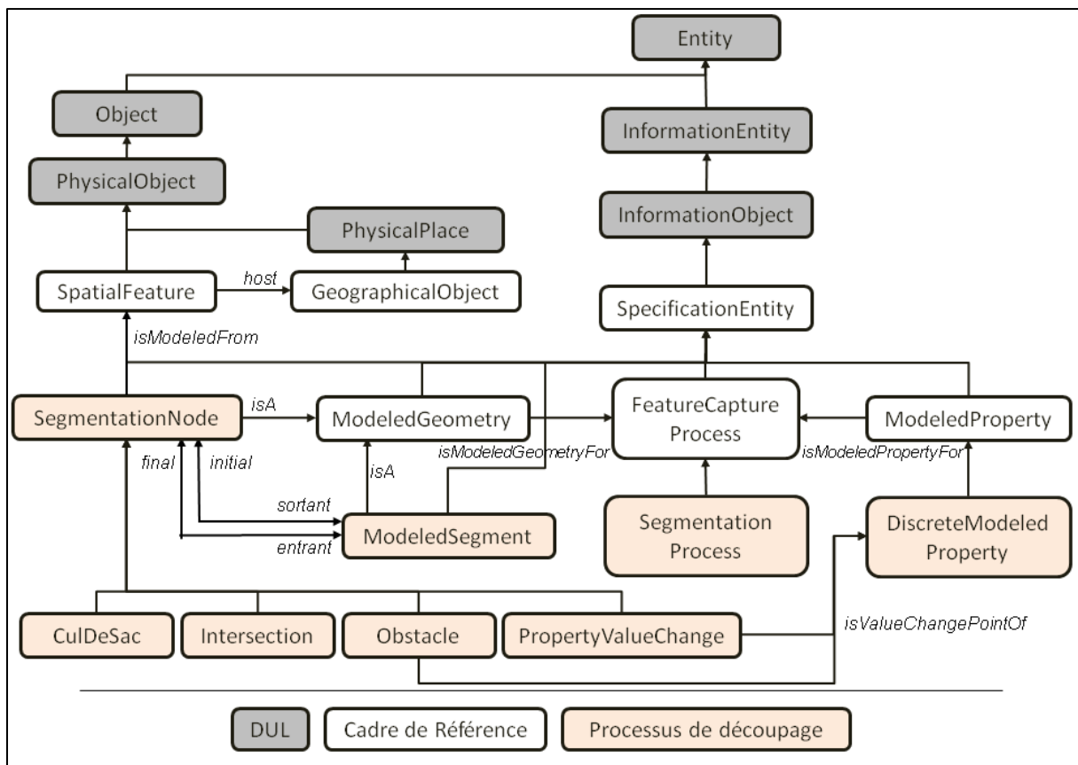
Figure 51: Cadre de référence sémantique pour la représentation du processus de découpage des entités topographiques de type réseau
