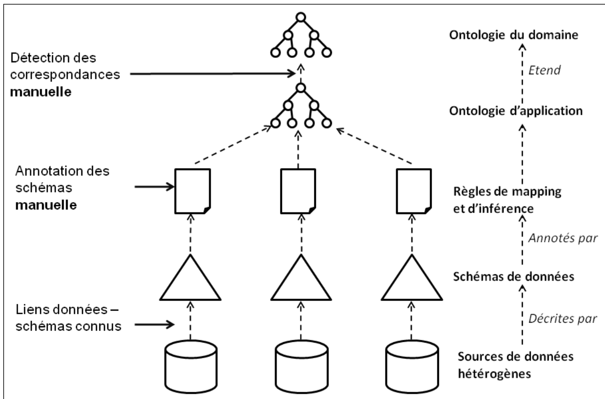
Figure 10: Approche proposée par (Zhao et al., 2008) pour la découverte des données: identification des étapes automatiques et manuelles
