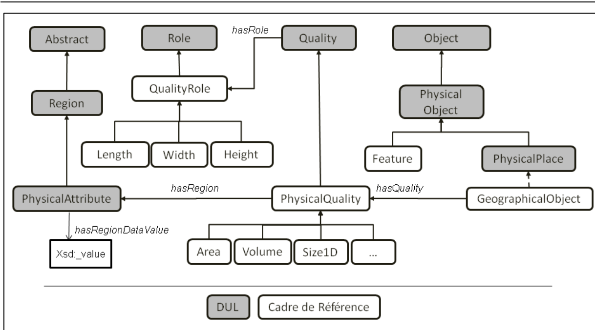
Figure 42: Cadre de référence sémantique pour la représentation des propriétés physiques des catégories d'entités topographiques
