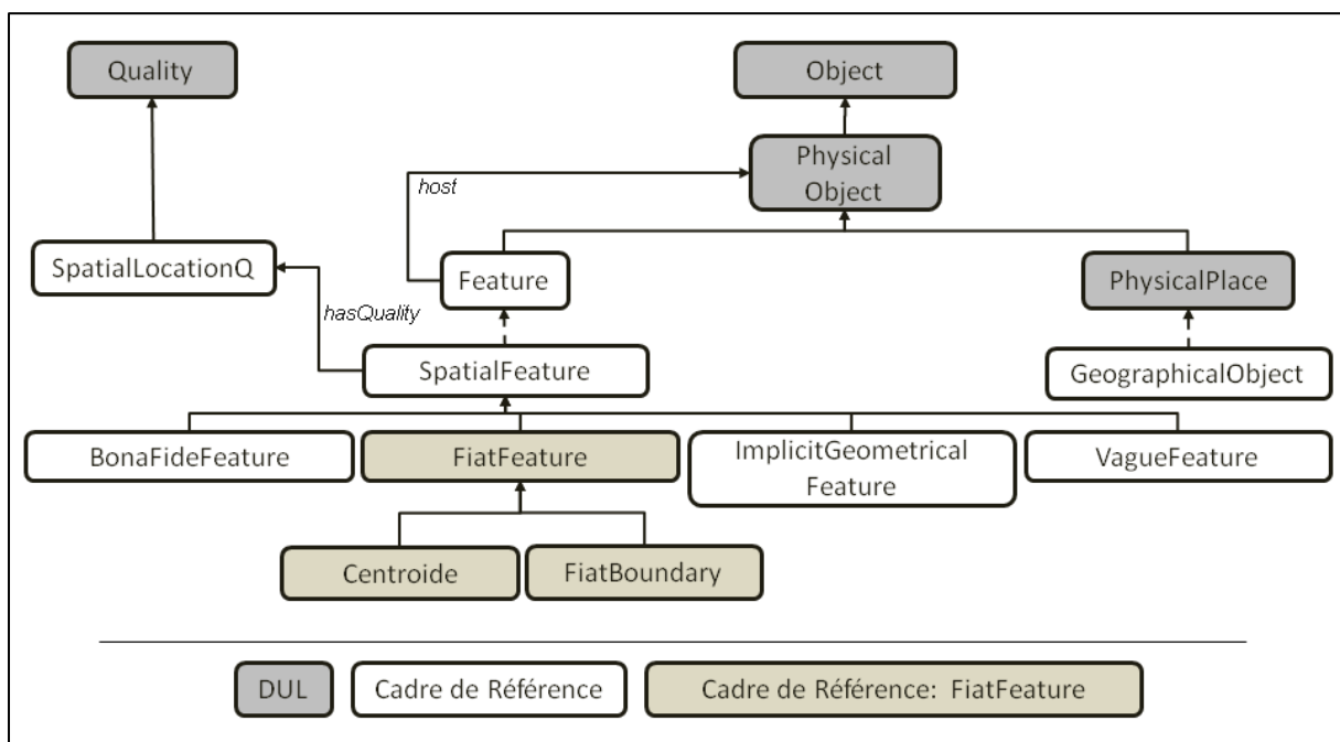
Figure 47: Cadre de référence sémantique pour la représentation des éléments caractérisant la forme des entités géographiques de type Fiat
