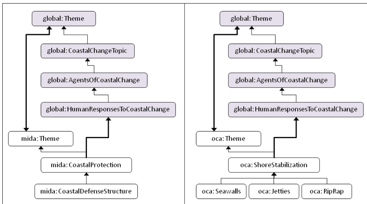
Figure 7: Extraits de deux ontologies de mappings d'après (Lassoued et al., 2008). A gauche celle reliant l'ontologie Marine Irish Digital Atlas à l'ontologie globale, à droite celle reliant l'ontologie Oregon Coastal Atlas à l'ontologie globale.
