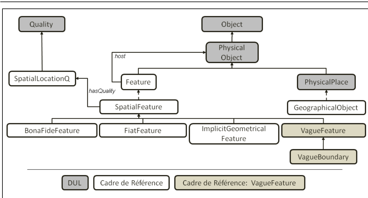
Figure 49: Cadre de référence sémantique pour la représentation des éléments caractérisant la forme des entités géographiques ne pouvant être déterminés avec précision
