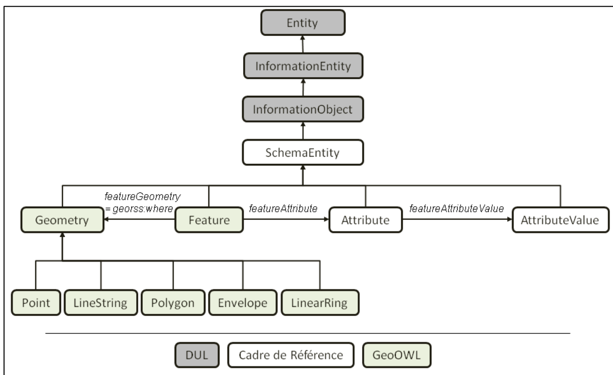
Figure 39: Partie du cadre de référence sémantique destinée à la représentation des éléments de schémas de bases de données topographiques
