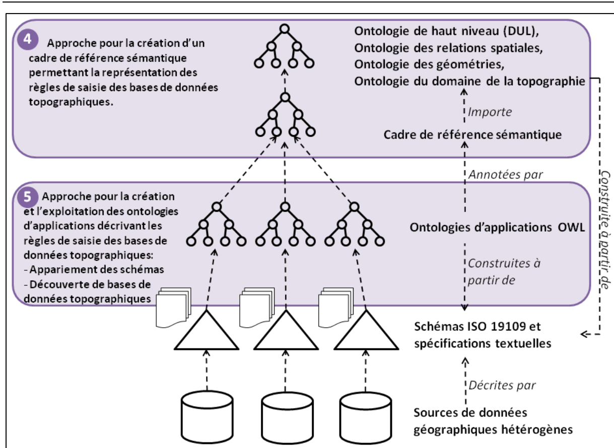
Figure 66: Principales contributions pour l'approche d'appariement fondée sur les spécifications des bases de données topographiques
