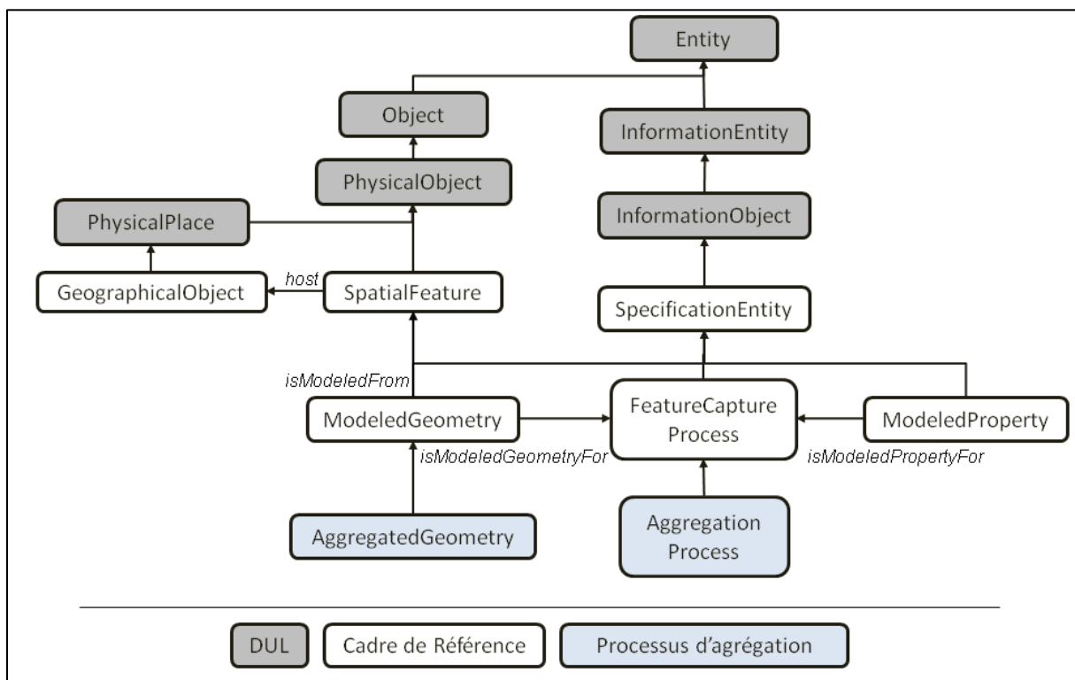
Figure 52: Cadre de référence sémantique pour la représentation du processus d'agrégation des entités topographiques
