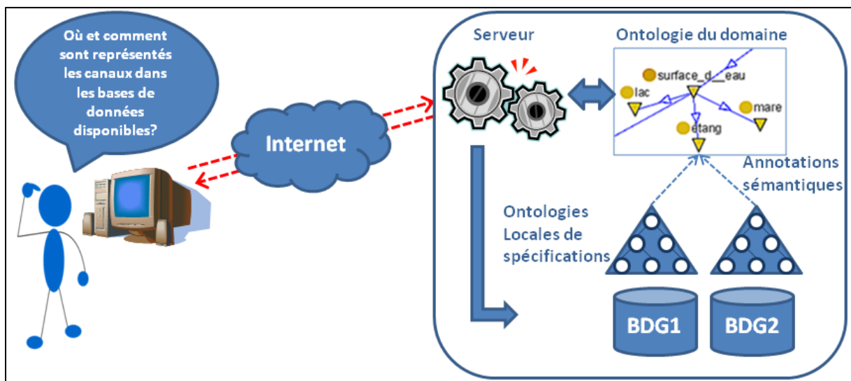
Figure 55: Architecture globale du système pour la découverte de bases de données topographiques hétérogènes
