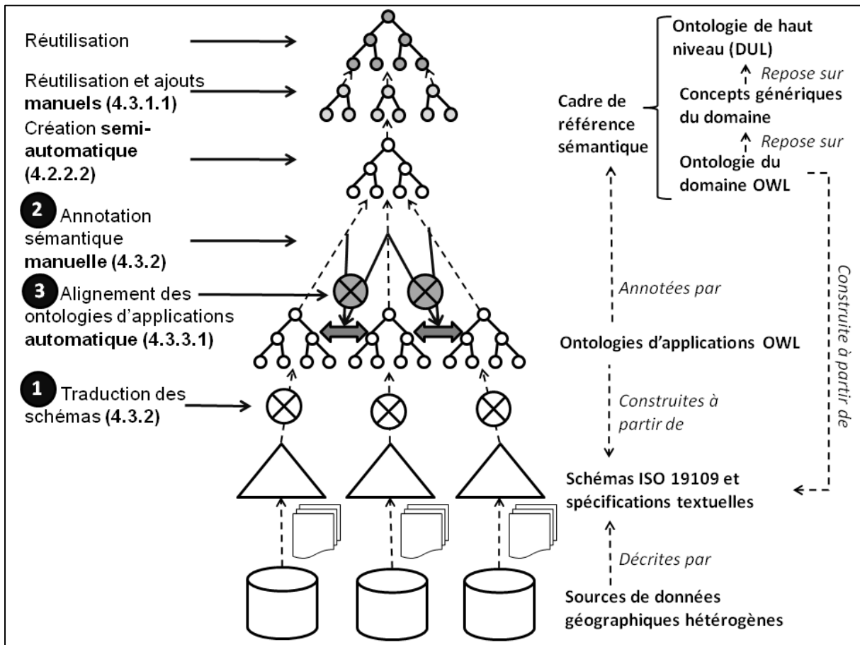
Figure 38: Architecture globale pour l'intégration virtuelle de bases de données géographiques fondées sur les spécifications de ces bases ; processus global d'appariement des schémas
