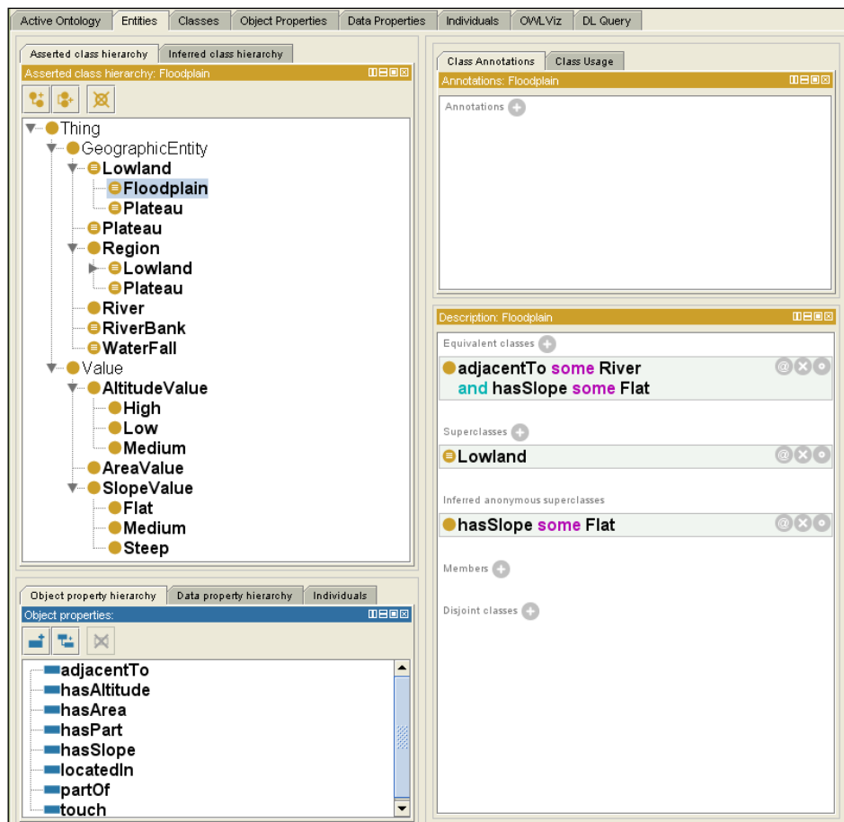
Figure 14: Ontologie du domaine OWL proposée par (Klien, 2008), visualisation sous Protégé 21
