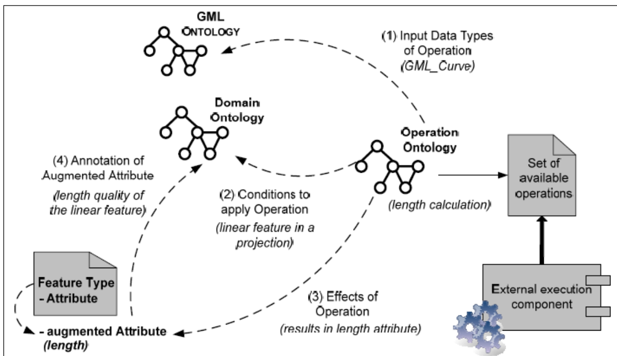
Figure 19: Description des opérations de transformation de données disponibles via l'ontologie des opérations extrait de (Schade, 2010)
