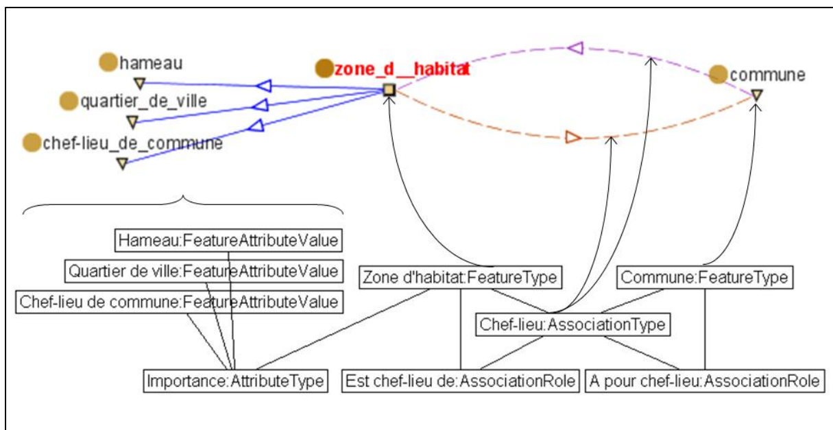
Figure 25: Traduction d'un extrait du schéma de la BDTOPO Pays 1.2 représenté selon le schéma ISO 19109 (en bas de l'image), en ontologie au format OWL (en haut de l'image, visualisation sous Protégé)
