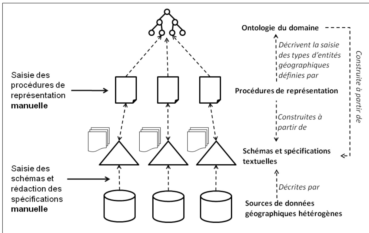
Figure 21: Approche proposée par Gesbert (2005): identification des étapes d'annotation automatiques et manuelles
