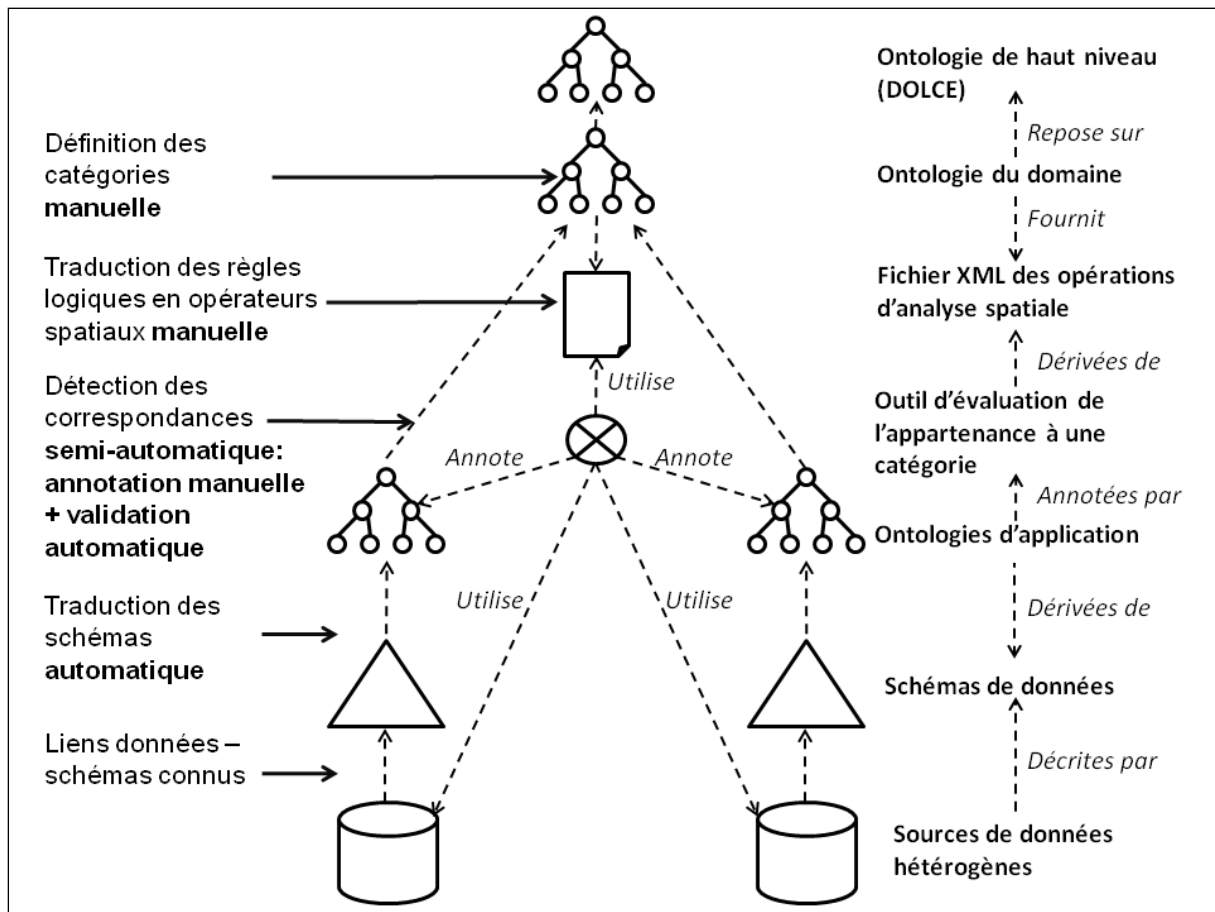
Figure 15: Approche proposée par (Klien, 2008) pour l'annotation semi-automatique de données géographiques: identification des étapes automatiques et manuelles
