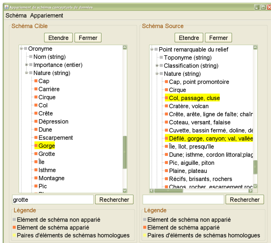
Figure 36: Apports de l'ontologie de support dans le processus d'appariement: appariement valeurs d'attributs Gorge et Col, passage, cluse
