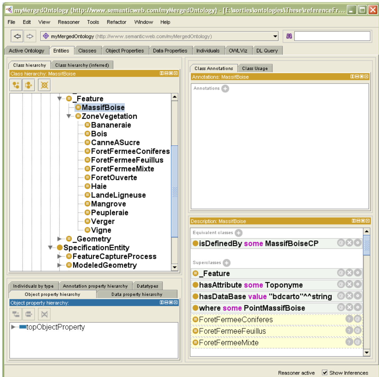
Figure 53: Utilisation d'un système de raisonnement pour ontologies pour l'appariement des classes Massif Boisé et Zone_Végétation (Visualisation sous Protégé)
