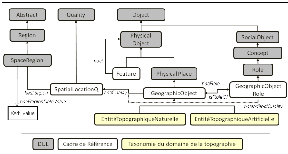
Figure 41: Cadre de référence sémantique pour la représentation des catégories d'entités topographiques, de leurs rôles et de leurs propriétés
