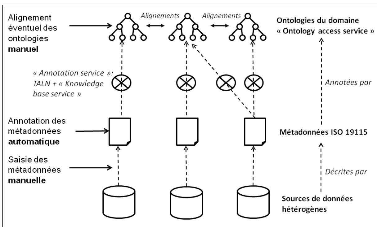
Figure 12: Approche proposée par (Bügel et al., 2007) pour la découverte des données: identification des étapes automatiques et manuelles
