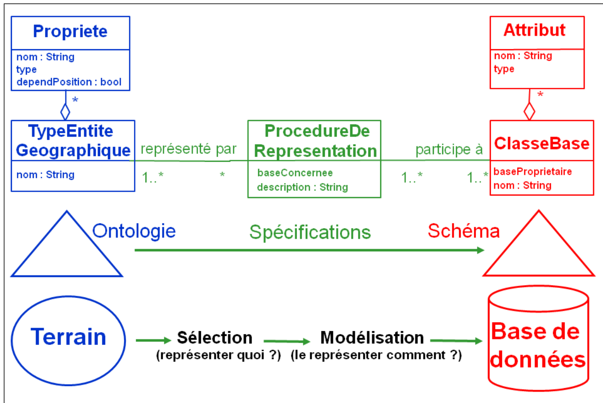
Figure 22: Modèle global pour la représentation des spécifications de bases de données géographiques, extrait de (Gesbert, 2005)
