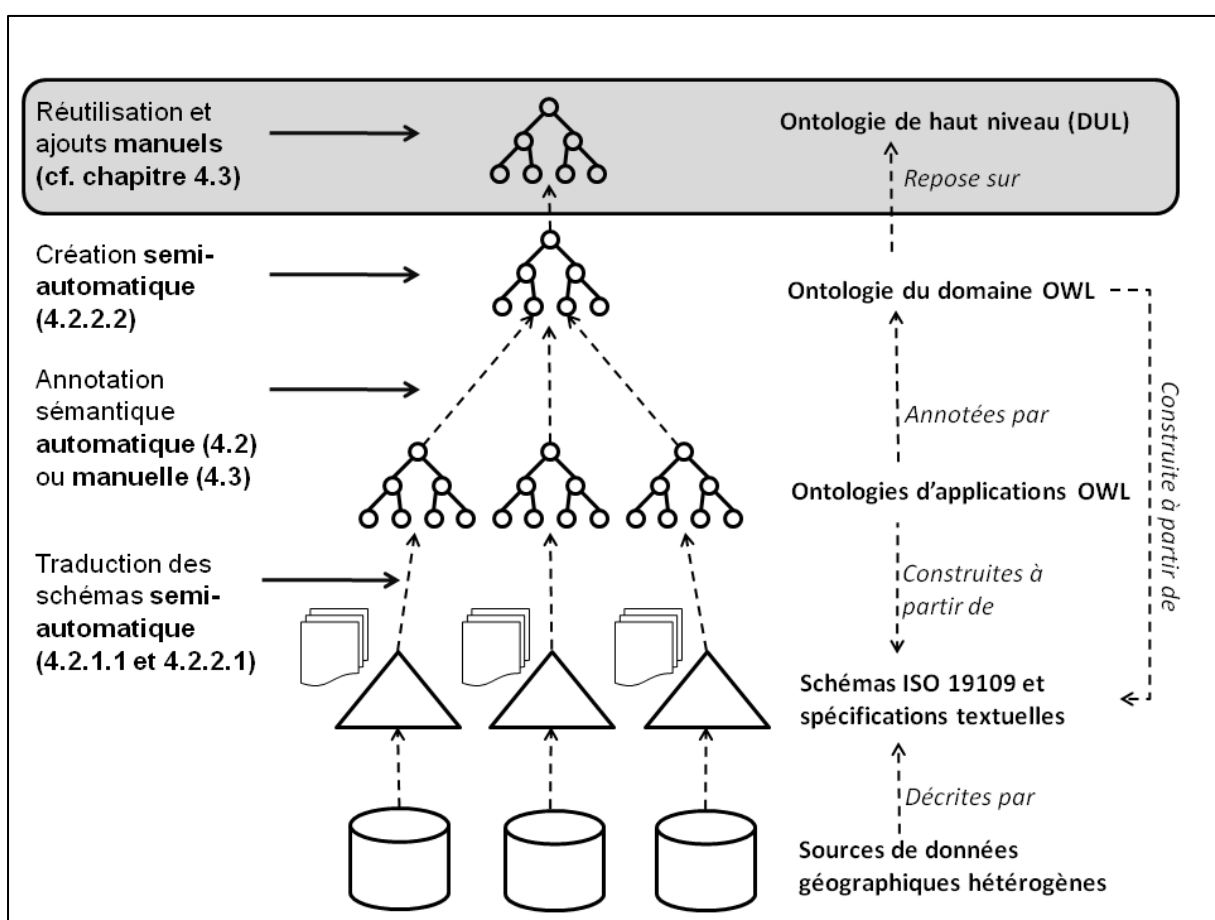
Figure 23: Architecture globale du modèle proposé: identification des étapes d'annotation automatiques et manuelles
