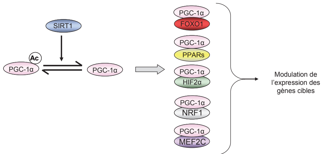
Figure 23 : Modulation de l'activité transcriptionnelle des facteurs de transcription par PGC-1α.
