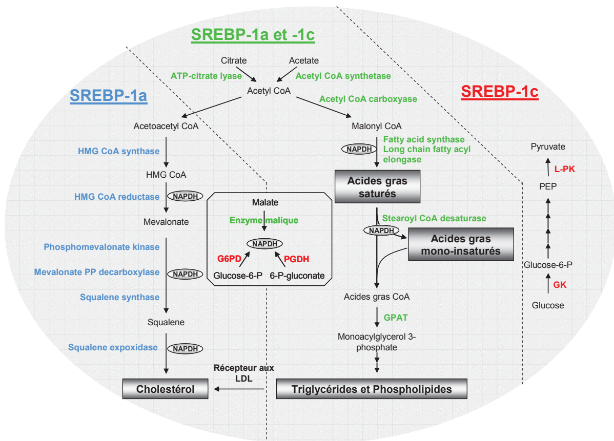
Figure 13 : Gènes et voies métaboliques régulés par SREBP-1a et SREBP-1c
