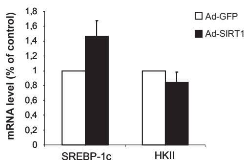
Figure 34 : SIRT1 régule l'expression des ARNm d'HKII et de SREBP-1c
