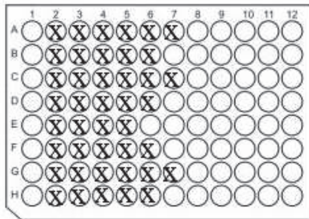
Figure 32 : exemple de titration adénovirale après 10 jours d'infection.
