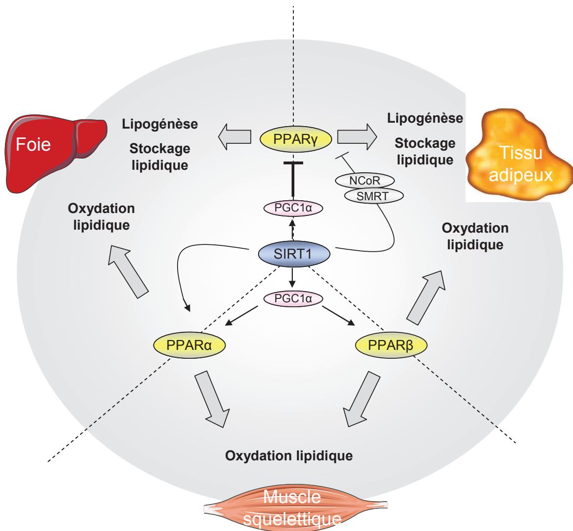
Figure 25 : SIRT1 régule l'activité transcriptionnelle des PPARs et module le métabolisme lipidique.
