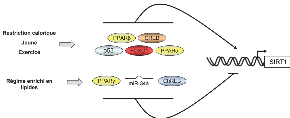
Figure 19 : Régulation de l'expression SIRT1
