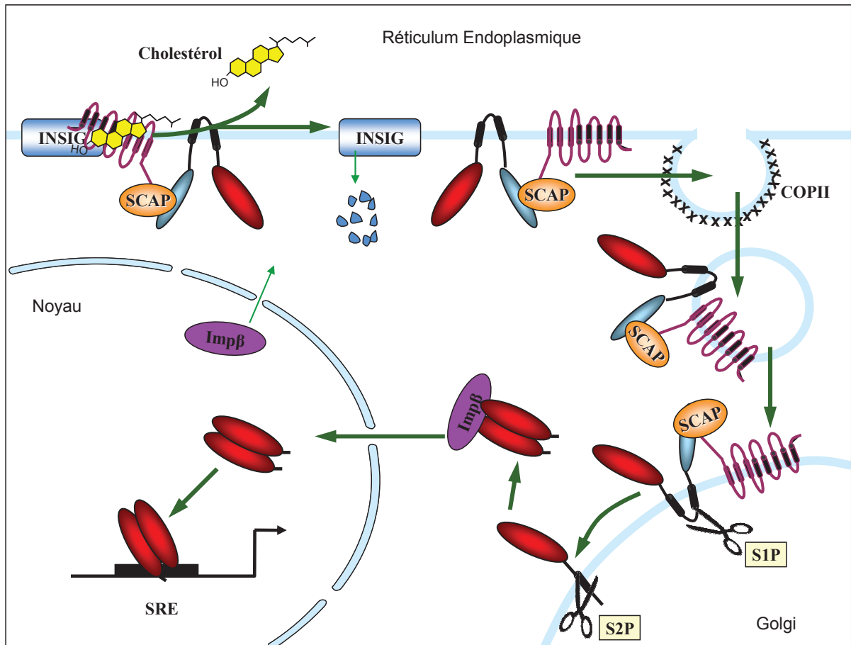
Figure 12 : Processus de maturation de SREBP-1 et régulation par les stérols
