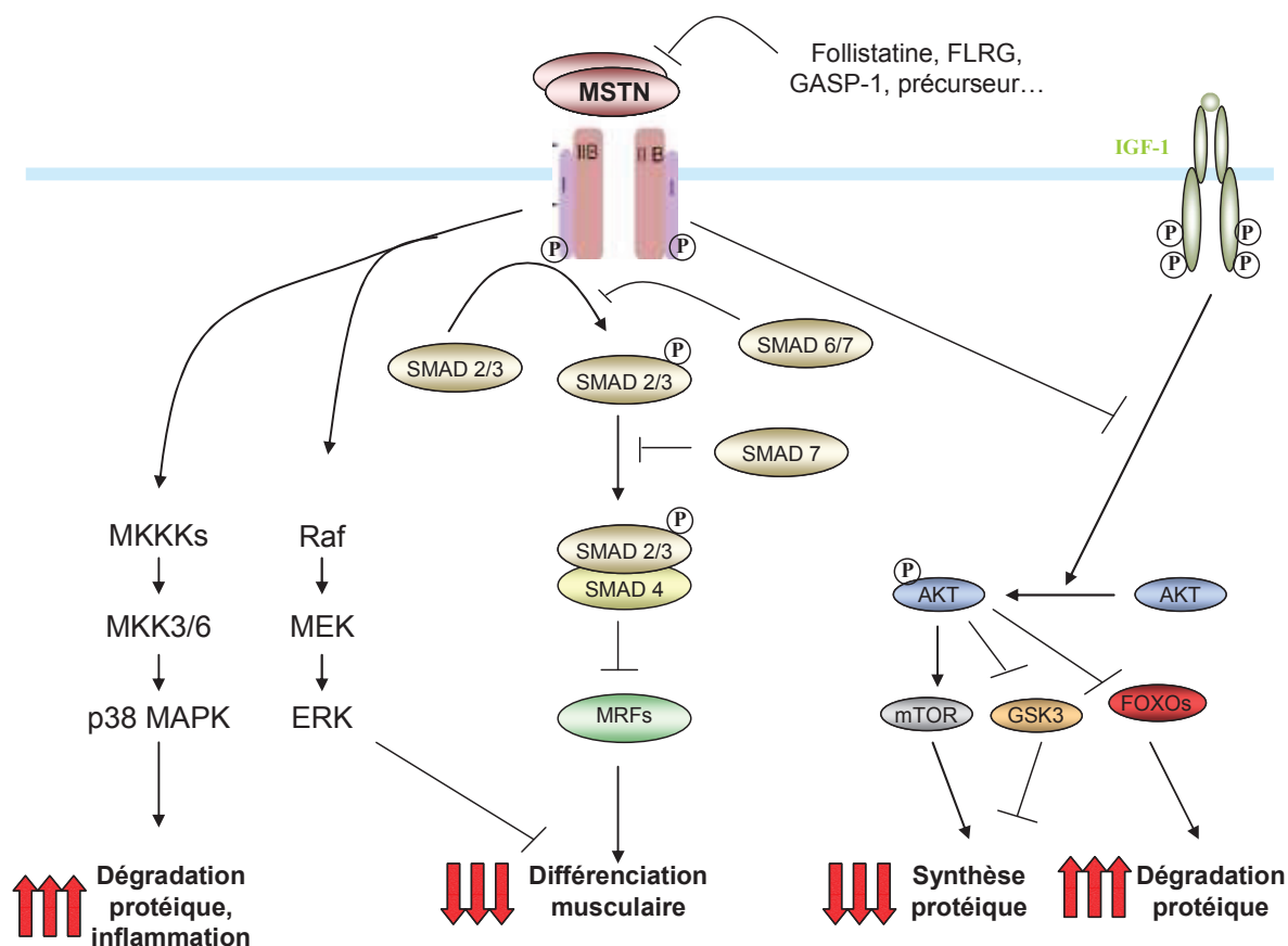
Figure 10 : Les différentes voies d'action de la myostatine.
