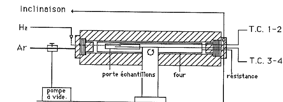
Schéma général de l'A.C.I.
