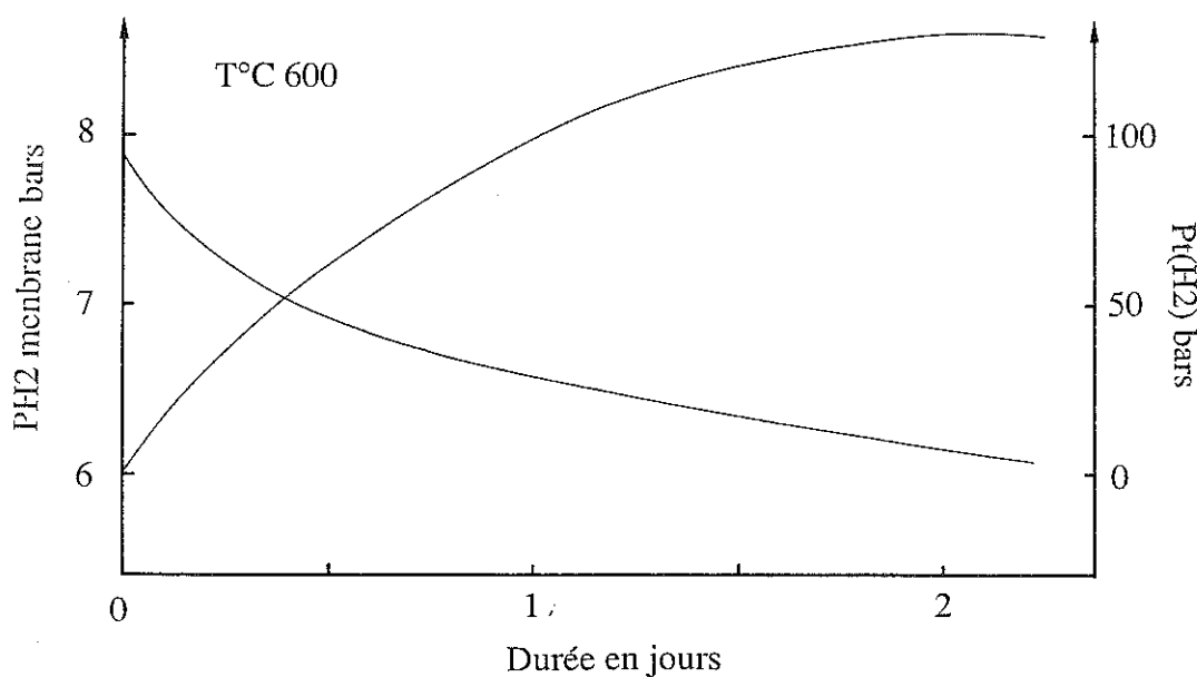
Fig. 74: Exemple d'équilibration membrane-autoclave (transfert \text{H}_2 de l'autoclave vers la membrane). P_t = P_{\text{H}_2} . Une fois l'équilibre atteint (droite en tireté), l'autoclave a été regonflée à 160 bars en P_t , avec de l'Ar, pour s'assurer que le phénomène observé correspondait bien à de la diffusion.
