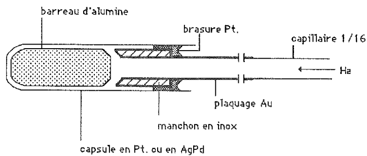
Détail de la membrane à hydrogène
