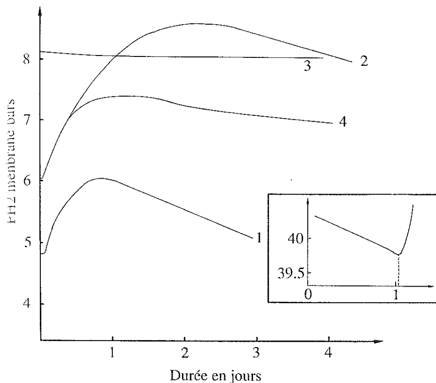
Fig. 73: Courbes de diffusion obtenues sur une autoclave à joint froid de faible volume (4 cc). Pour les courbes (1), (2) et (4), les trois parties décrites dans le texte se distinguent nettement. En médaillon est représenté un exemple de fuite (bombe vers membrane). Toutes les expériences ont été réalisées à T = 600^{\circ}\text{C} . Les conditions expérimentales sont;
