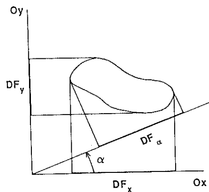
Fig.46. Principe de la m  thode des diam  tres de F  ret. DF x et DF y sont les diam  tres de F  ret respectivement parall  les    O x et    O y . DF α est le diam  tre de F  ret mesur   dans le direction α. (d'apr  s Lapique, 1987).
