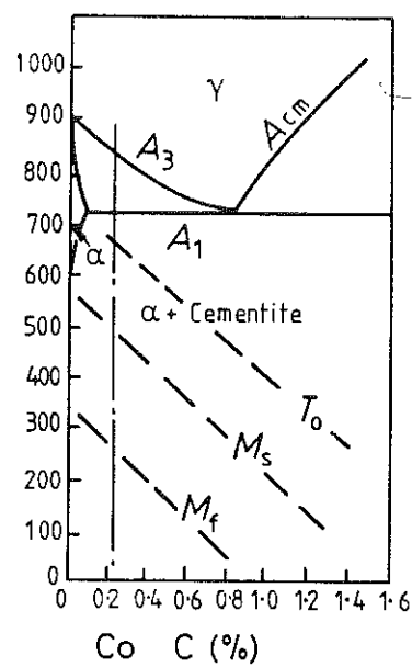
Fig. 75: Diagramme de phase Fe-C-Co ( in Porter et Easterling, 1981). L'effet de l'adjonction du Co dans l'alliage Fe-C (pour une teneur donnée en C) sur les températures Ms et Mf est indiqué
