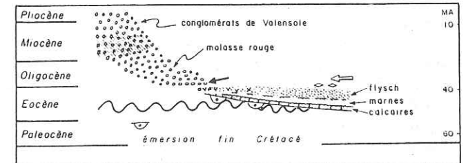
Fig. 47 - Schéma de la disposition relative des dépôts paléogènes et néogènes de la zone externe méridionale (Boillot et al. , 1984).
