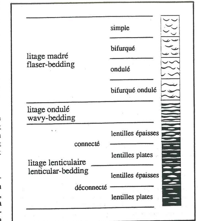
Fig. 33 - Les litages de rides madré, ondulé et lenticulaire (Flaser-, wavy- et lenticular-bedding) (Reineck et Wunderlich, 1968)
