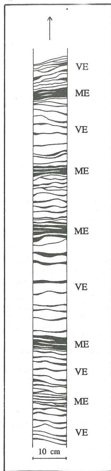
Fig. 121 - Carotte de 10 cm de diamètre simulée dans les alternances gréso-silteuses à wavy-bedding enregistrant des cycles de morte-eau/vive-eau (exemple de Saint-Symphorien, d'après diapositive). Les dilatations et les amincissements des lits successifs sont facilement identifiables
