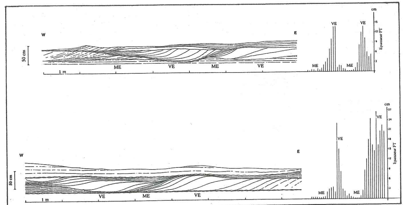
Fig. 95 - Les mégarides à cycles semi-lunaires de l'affleurement d'Auribeau ME, morte-eau ; VE, vive-eau ; FT, faisceaux tidaux
