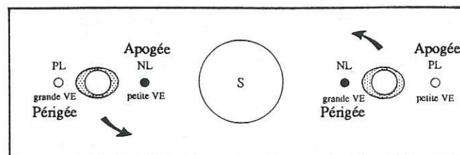
Fig. 5 - Explication du cycle lunaire (grande vive-eau/petite vive-eau) NL, nouvelle lune ; PL, pleine lune ; VE, vive-eau
