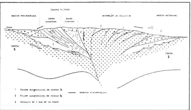
Fig. 49 - Localisation des bassins d'avant-pays périphérique et rétro-arc dans une chaîne de montagne issue d'une collision (Souquet, 1981)
