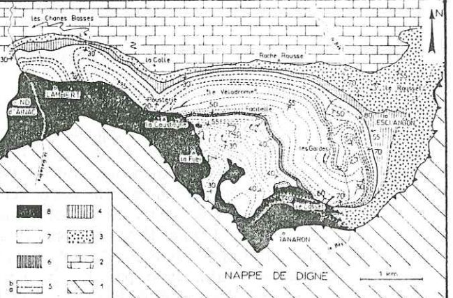
Fig. 51 - Carte simplifiée de la bordure nord du bassin de Digne entre Esclangon et Lambert (Gigot et al. , 1974). (1), Nappe de Digne; (2), substratum mésozoïque de la demi-fenêtre de Barles; (3), Molasse rouge oligocène; (4), Molasse intermédiaire; (5), Molasse marine miocène (a, membre 1, et b, membre 2); (6 & 7), Molasse jaune mio-pliocène; (8), "bassin résiduel"
