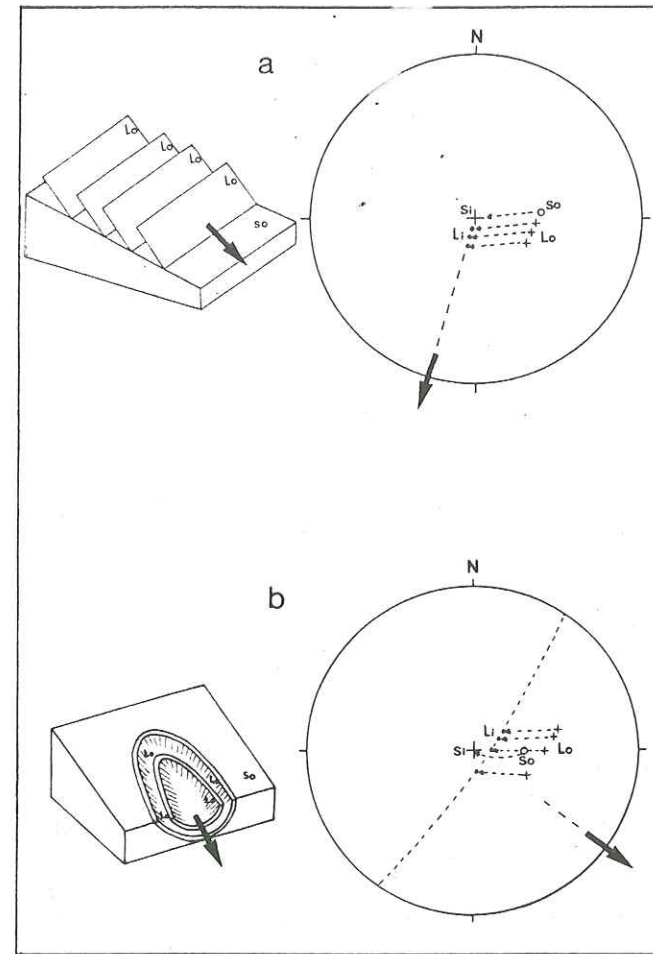
Fig. 72 - Méthode utilisée pour la reconstitution des sens de paléocourants dans la molasse marine du ravin de Saint-Symphorien. (a), dans le litage oblique plan ; (b), dans le litage oblique arqué (d'après Durand et Noblet, 1986). La flèche indique le sens de transport. S0, plan de stratification générale mesuré ; L0, plan de litage oblique mesuré ; Si, plan de stratification générale initial ; Li, plan de litage oblique initial. (canevas de Wulff, hémisphère supérieur)
