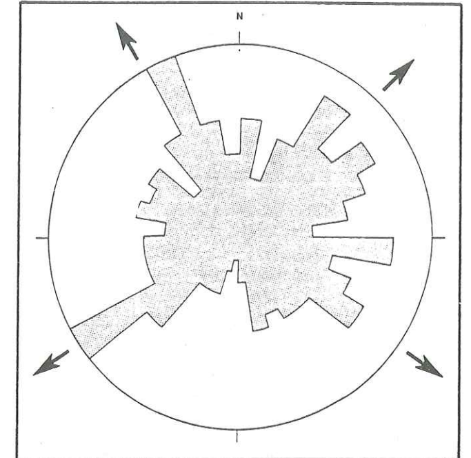
Fig. 73 - Rosace de l'ensemble des sens de paléocourants dans la molasse marine du ravin de Saint-Symphorien
