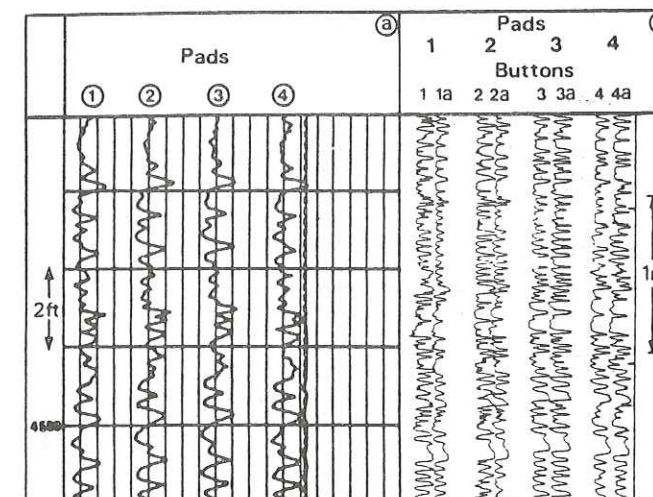
Fig. 122 - Exemple de courbes de résistivité fournies par le pendagemètre (H.D.T. et S.H.D.T.)
