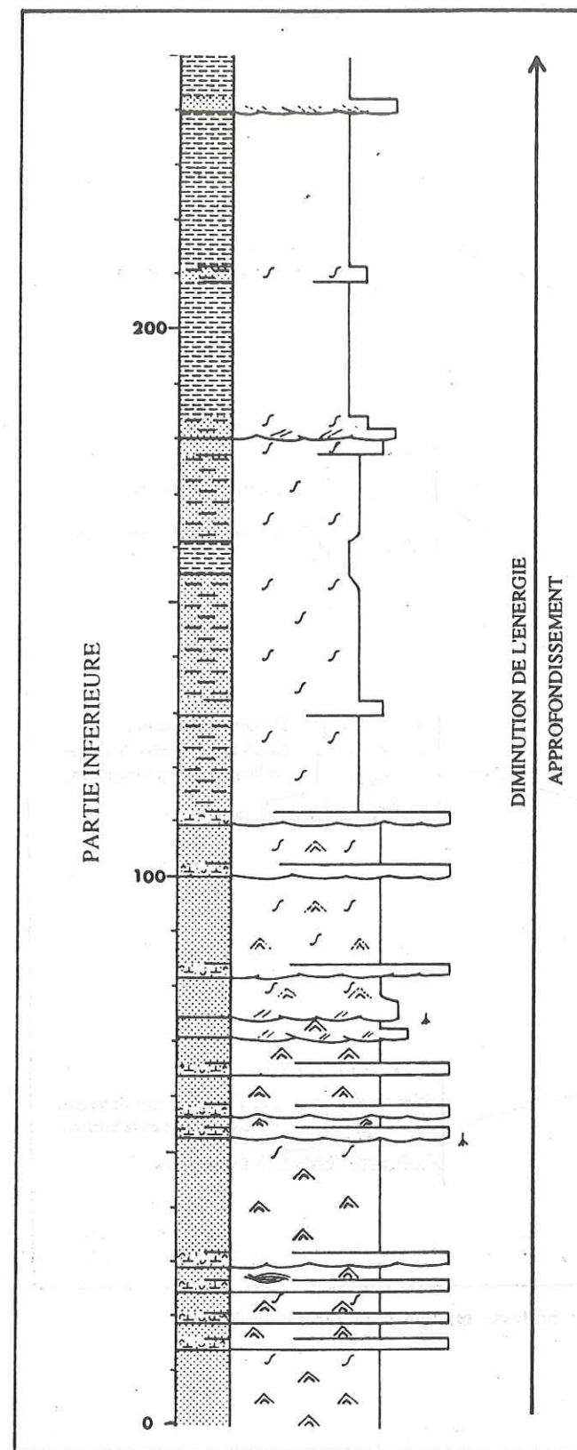
Fig. 68 - La partie inférieure de la molasse marine dans le ravin de Saint-Symphorien. L'évolution verticale des faciès (diminution du matériel bioclastique, apparition progressive de la bioturbation, affinement général du matériel détritique) reflète un approfondissement du milieu. Il s'agit d'une séquence transgressive (Voir légende Fig. 64bis)
