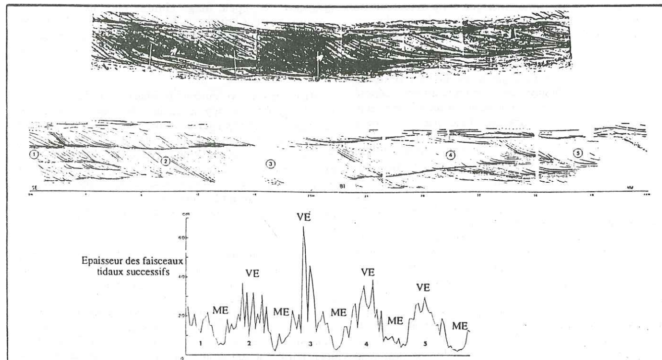
Fig. 13 - Exemple de cycles semi-lunaires identifiés dans une mégaride holocène de l'estuaire du Oosterschelde (d'après Yang et Nio, 1985)
