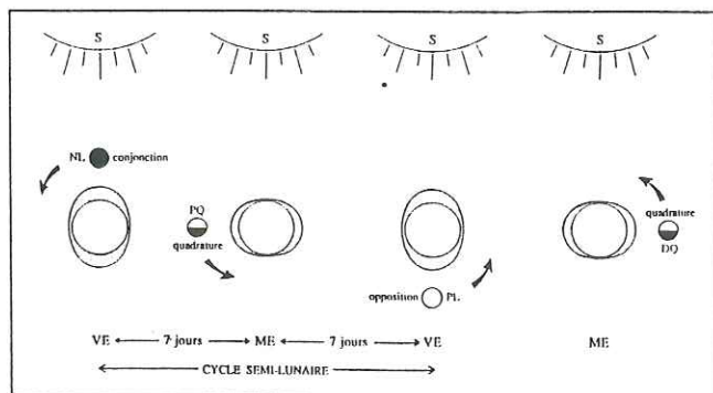
Fig. 4 - Explication du cycle semi-lunaire (morte-eau/vive-eau) NL, nouvelle lune ; PL, pleine lune ; VE, vive-eau ; ME : morte-eau
