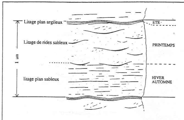
Fig. 43 - Schématisation du cycle d'origine annuelle et son interprétation.
