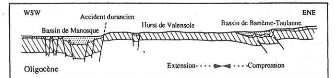
Fig. 48 - Structuration du domaine subalpin méridional pendant l'Oligocène (d'après Gigot et al. , 1975)
