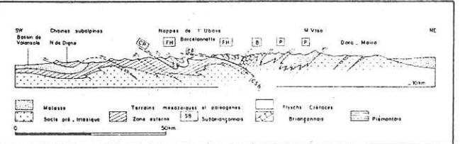
Fig. 50 - Coupe simplifiée des Alpes occidentales selon la transversale Barcelonnette-Digne (Boillot et al. , 1984) montrant notamment la position du bassin d'avant-pays molassique de Digne-Valensole. CP, chevauchement pennique; FH, nappes de flyschs à Helminthoïdes; SB, Subbriançonnais; B, Briançonnais; P, Piémontais; CSB, "cicatrice" subbriançonnaise
