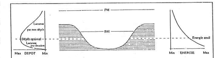
Fig. 107 - Interprétation hypothétique de la grande période composant l'enregistrement de Saint-Symphorien. PM, pleine mer ; BM, basse mer
