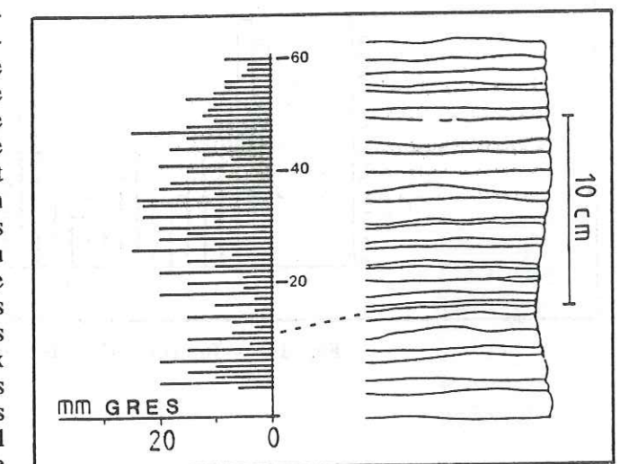
Fig. 108 - Exemple d'ESCLANGON. Evolution verticale de l'épaisseur des lits gréseux successifs
