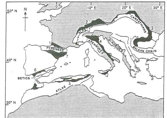
Fig. 46 - Localisation des bassins d'avant-pays dans l'Europe alpine et les régions voisines (Allen et al. , 1986). (1), bassin aquitain; (2), bassin molassique Nord alpin; (3), bassin des Carpathes; (4), bassins des Apennins et du Pô; (5), bassins atlasiques (Tello-Rifain); (6), bassin Nord bétique; (7), bassin Sud Pyrénéen et bassin de l'Ebre
