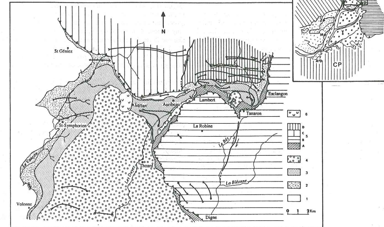
Fig. 45 - Carte structurale de la bordure septentrionale du bassin de Digne (d'après Haccard et al. , 1989a). (Cartouche : ND, nappe de Digne; SA, Secondaire autochtone; CP, Chaînons de Provence; D, Digne; S, Sisteron; F, Forcalquier; M, Manosque; V, valensole; AD, accident durancien). (1), Secondaire autochtone; (2), Molasse rouge oligocène; (3), Molasse marine miocène; (4), Conglomérats de Valensole mio-pliocènes, (5), complexe de l'Arc chevauchant de Digne: A, olistostrome de la Nappe de Digne ou "bassin résiduel"; B, Nappe de Digne; C, Unité de Mélan-Clamensanne; D, Unité d'Esclangon-Grande Cloche; (6), glissement de Mélan; —, anticlinaux; —, synclinaux; —, contact chevauchant.
