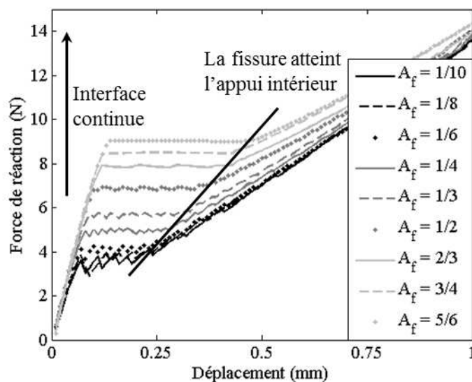
Figure IV-31 : Flexion 4-points : Courbes de chargement ( force=f(déplacement) ) pour différentes valeurs d'aire de contact A_f ( w = 160 \mu m ).
