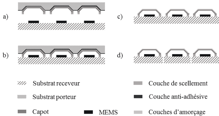
Figure I-3 : Principe de réalisation du report de capots par transfert de films : a) Aligment ; b) Scellement ; c) Libération ; d) Découpe.
