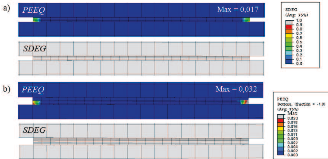
Figure IV-46 : T_{max} / \sigma_y = 2 : a) T_{max} = 30\text{ MPa} ; b) \sigma_y = 30\text{ MPa} .
