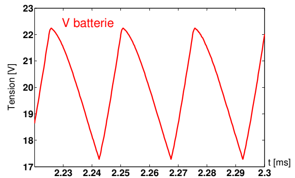
Figure 5.16 : tension aux bornes des batteries
