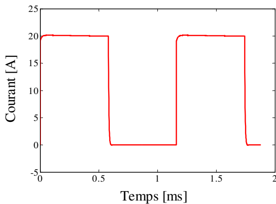
Figure 5.22 : courant de pile à 860 Hz (simulation)
