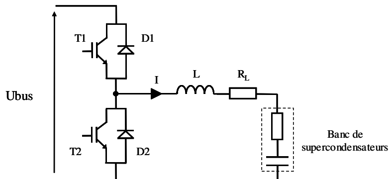
Figure 3.23: structure du hacheur élévateur en tension, réversible en courant
