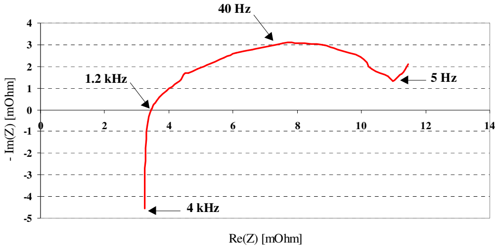
Figure 23 : diagramme d'impédance, courant de polarisation de 300 A
