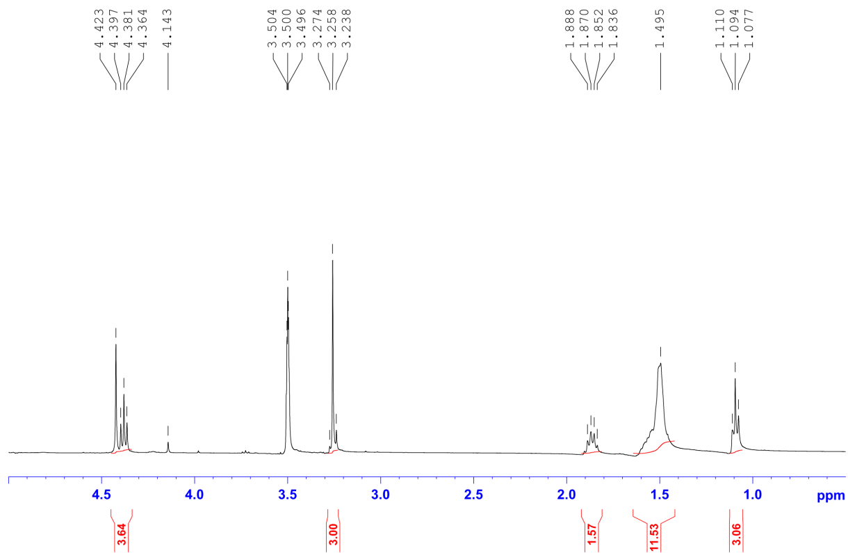
Trotier-Faurion et al., Suppl Figure 10 ( ^1\text{H} NMR)
