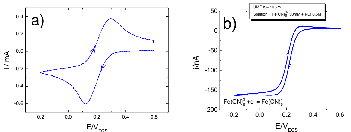
Figure 37 : (a) Voltammétrie cyclique du substrat de Pt avec une vitesse de balayage v = 100 mV/s, (b) Voltammétrie cyclique d'une microélectrode de 10 \mu\text{m} de rayon avec une vitesse de balayage de 10 mV/s ; solution \text{Fe}(\text{CN})_6^{3-} 50 mM + KCl 0,5 M.
