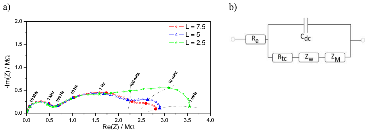
Figure 27 : a) Diagrammes d'impédance obtenus sur une UME de 10 μm de rayon au potentiel d'équilibre en fonction de la distance sonde-substrat dans une solution de 10 mM K_3Fe(CN)_6 + 10 mM K_4Fe(CN)_6 + 0,5 M KCl ; b) Circuit équivalent total de la diffusion en couche mince d'une microélectrode.
