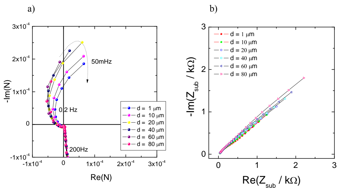
Figure 56 : a) Fonction de transfert complexe N(\omega) expérimentale et b) l'impédance expérimentale du substrat Z_{\text{sub}}(\omega) , E_{\text{sub}} = -0,25 V_{ECS} , la sonde de 20 \mu\text{m} de rayon et le substrat de Platine de 0,5 cm de diamètre dans une solution \text{HClO}_4 0,1 M + \text{KBr} 5 mM.
