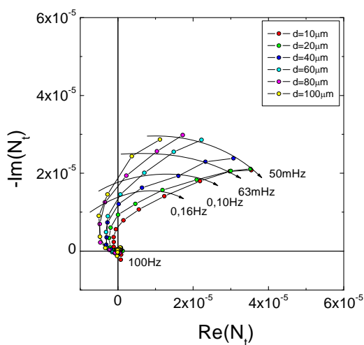
Figure 47 : Coefficient de transport complexe expérimental N_i(\omega) (substrat d'or) en fonction de la distance sonde-substrat avec une UME de 20 \mu m de rayon dans une solution H_2SO_4 0,5 M, fréquences : de 100Hz à 0,05Hz; le potentiel de la sonde est maintenu constant à 0,2 V_{ECS} , le substrat est polarisé à -0,258 V_{ECS} .
