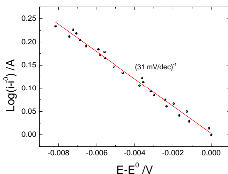
Figure 46 : Diagramme de Tafel pour la réaction HER sur le substrat d'or dans solution H_2SO_4 0,5M.
