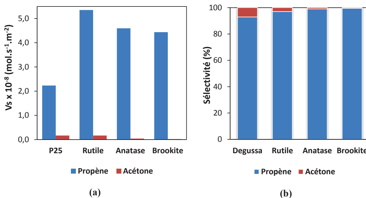
Figure 33. Vitesse de réaction (a) et sélectivités en produits (b) obtenues sur différentes phases cristallines de TiO 2 et sur la référence P25 à 523 K.
