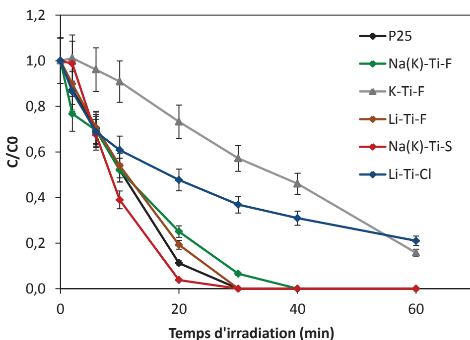
Figure 9. Photo-oxydation catalytique de l'acide formique pour TiO 2 préparé dans des nitrates fondus et pour la référence P25 (filtre « 0-52 », λ = 365 nm, I = 6,2 mW.cm -2 ).
