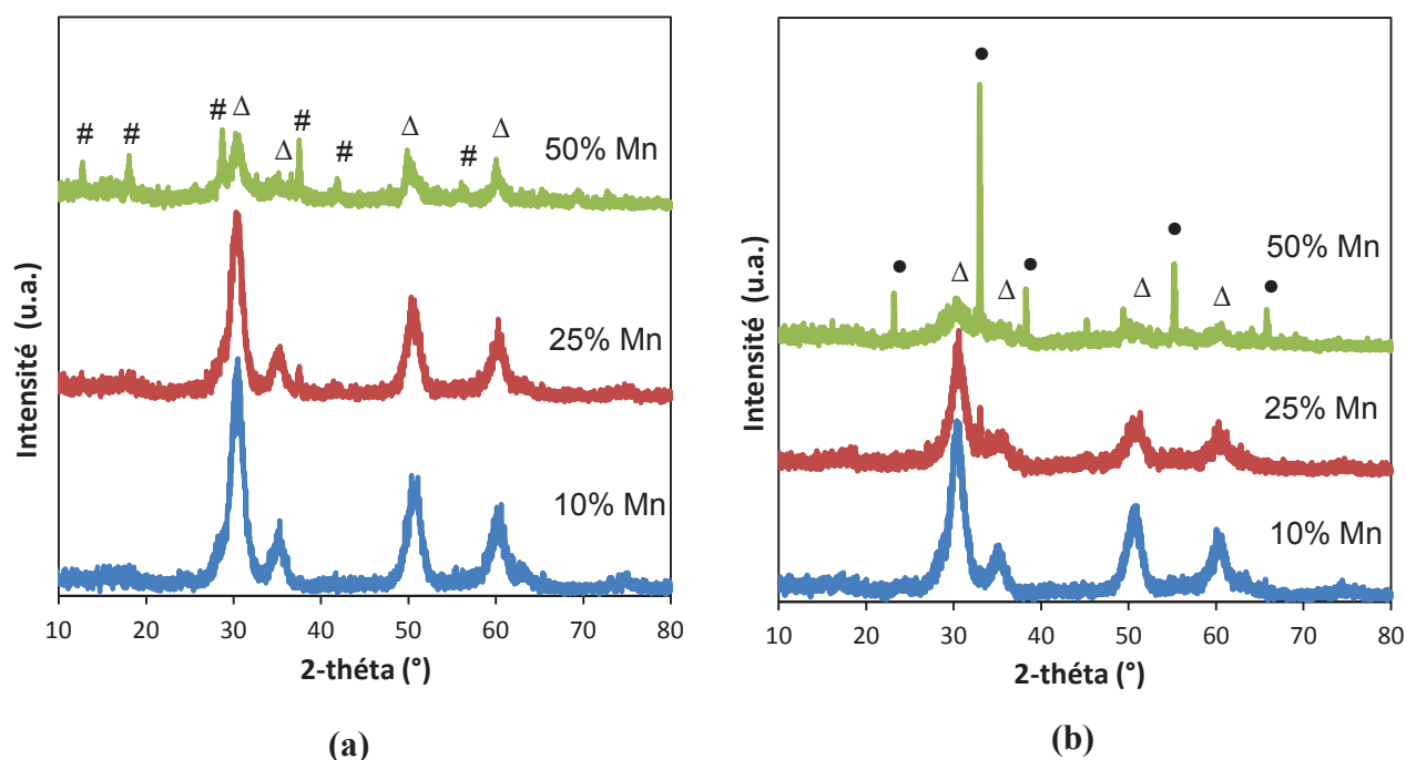
Figure 1. Clichés DRX des oxydes Mn-Zr obtenus en fonction de la teneur en Mn en utilisant comme précurseur (a) KMnO_4 et (b) MnCl_2 . Légende : # - K_xMn_8O_{16} cryptomélane; Δ - ZrO_2 (tétraonale); • - Mn_2O_3 .
