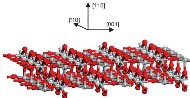
c) - Structure de la surface (110), rutile
