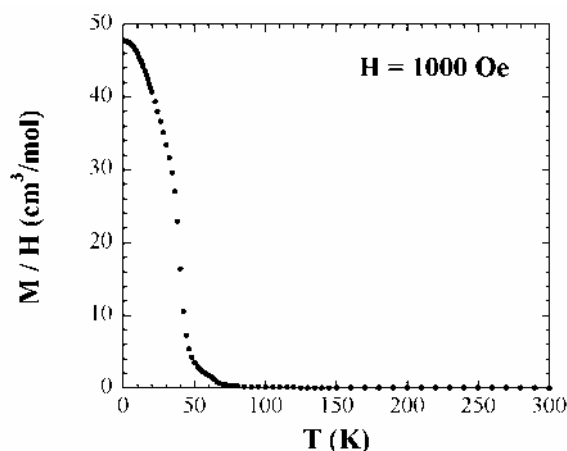
Figure 32 : Evolution de l'aimantation normalisée au champ magnétique de 2 en fonction de la température.
