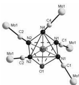
Figure 7 : Environnement et géométrie du Mn1 dans 6 .
