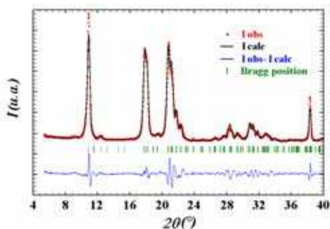
Figure 17 : Diffractogramme obtenu par diffraction des rayons X d'un échantillon brut. La ligne continue est le paramétrage des données expérimentales par la phase orthorhombique du KC_{60} en ajustant ses paramètres de maille à : a = 14,31 \text{ \AA} , b = 9,96 \text{ \AA} , et c = 9,11 \text{ \AA} .
