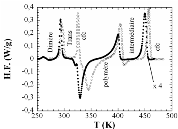
Figure 27 : Comparaison des thermogrammes obtenus après soustraction de la ligne de base d’un échantillon brut ayant subi une trempe dans le but de former la phase de dimères. Les symboles (O) représentent l’échantillon que nous avons mesuré. Les symboles (●) représentent l’échantillon de la référence [49].
