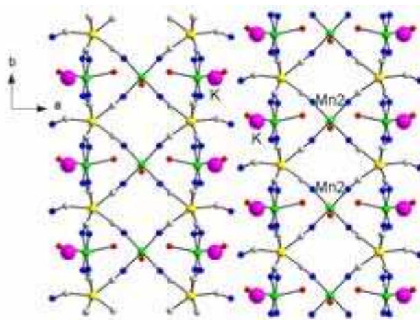
Figure 12 : Structure étendue de 2 dans le plan ab . Les molécules d'eau de cristallisation ont été enlevées pour des raisons de clarté.
