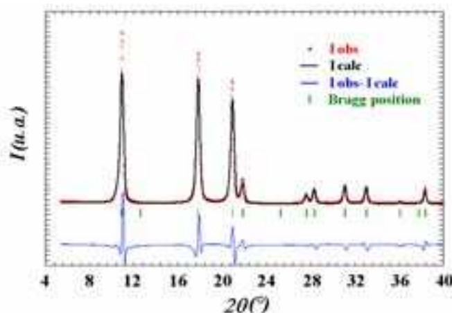
Figure 13 : Diffractogramme obtenu par diffraction des rayons X d'un échantillon brut exposé à l'air à 473 K. La ligne continue est le paramétrage des données expérimentales par la phase cubique du C_{60} en ajustant son paramètre de maille à 14,13 Å.
