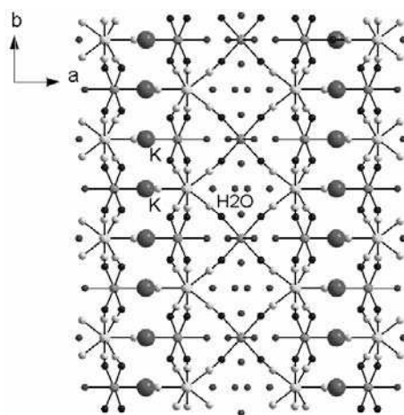
Figure 11 : Structure étendue de 6 dans le plan ab . Les cations K^+ sont entre les plans, tandis que les molécules d'eau sont entre les biplans.
