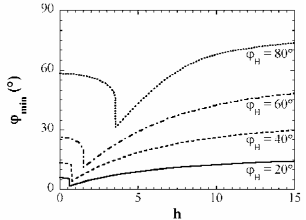
Figure 66 : Evolution de \varphi_{\min} en fonction de h pour différentes valeurs de \varphi_H (avec \eta = 1,7 et k = 0,5 ).
