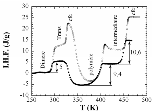
Figure 28 : Comparaison des courbes intégrales obtenues à partir des thermogrammes de la figure 27. Les symboles (O) représentent l’échantillon que nous avons mesuré. Les symboles (●) représentent l’échantillon mesuré de la référence [49].
