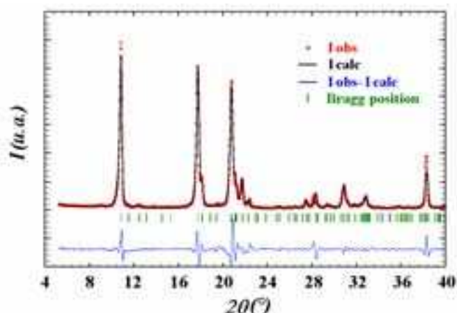
Figure 51 : Diffractogramme obtenu par diffraction des rayons X d'un échantillon brut. La ligne continue est le paramétrage des données expérimentales par la phase orthorhombique du KC_{60} en ajustant ses paramètres de maille à : a = 14,31\text{ \AA} , b = 9,94\text{ \AA} , et c = 9,12\text{ \AA} .
