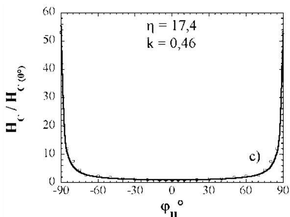
Figure 70 : Evolution du champ magnétique critique en fonction de \phi_H pour a) 1, b) 2, c) 3 à 2 K. Les lignes continues représentent le champ critique théorique pour a) 1, \eta = 1,7 et k = 0,5 , b) 2, \eta = 1,4 et k = 0,19 et c) 3, \eta = 17,4 et k = 0,46 .
