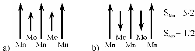
Figure 18 : Représentation schématique des différents alignements des spins dans la maille magnétique de 2 . a) alignement ferromagnétique des spins ( M_S = 17 \mu_B ) et b) alignement antiferromagnétique des spins ( M_S = 13 \mu_B ).
