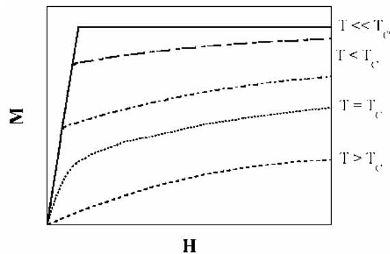
Figure 17 : Evolution schématique de l'aimantation en fonction du champ magnétique à différentes températures.
