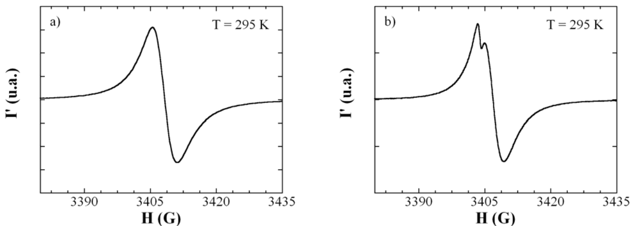
Figure 9 : Spectres RPE mesurés à température ambiante a) d'un échantillon brut et b) d'un échantillon brut mis en contact avec l'air à température ambiante.
