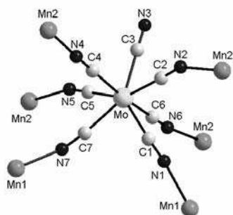
Figure 13 : Environnement du site Mo dans 2 .
