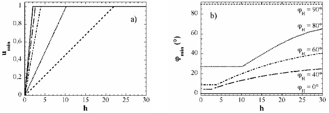
Figure 12 : Evolution de a) u_{\min} et b) \varphi_{\min} en fonction de la variable réduite h pour différentes valeurs de \varphi_H et a = 10 .
