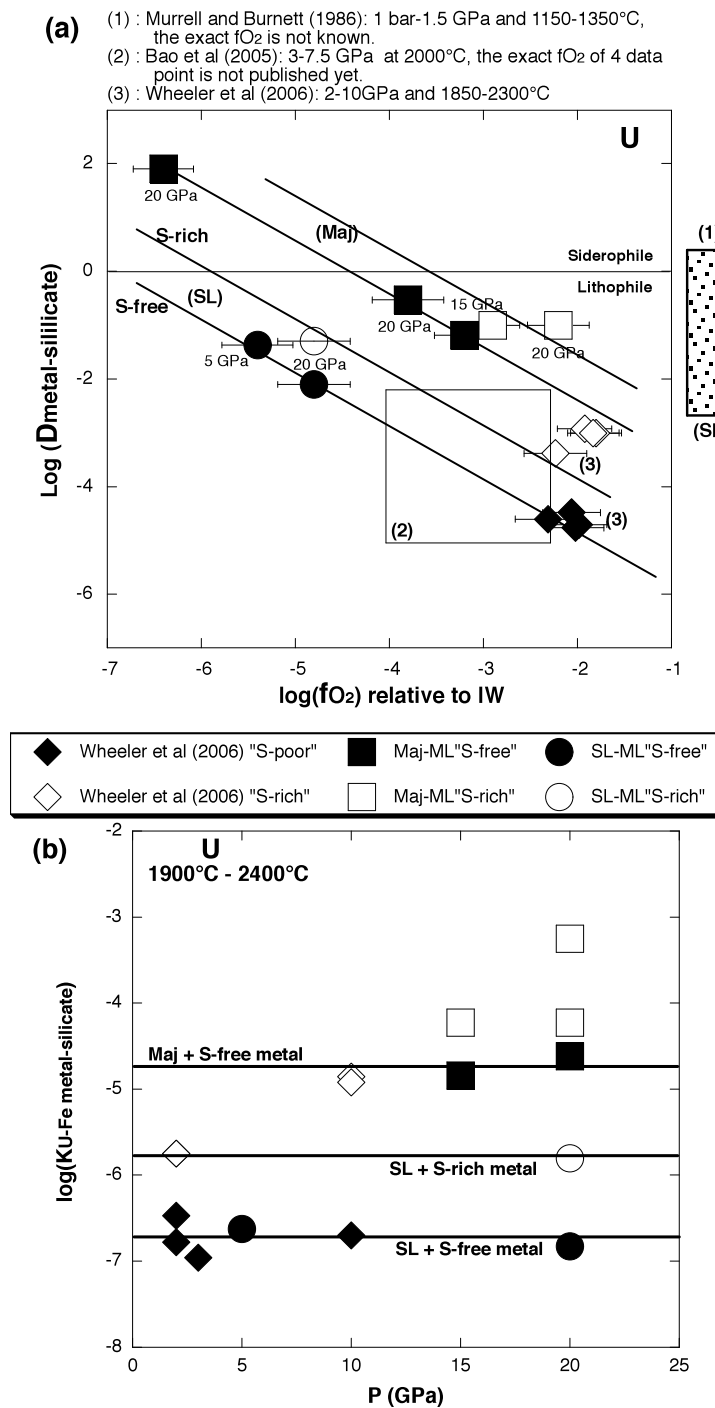
Figure 2.6 : Evolution du coefficient de distribution D^U entre métal et silicates en fonction de la fO_2 (a), puis du coefficient de partage K_d^U normalisé par rapport au fer en fonction de la pression (b). K_d de dépend pas de la fO_2 .
