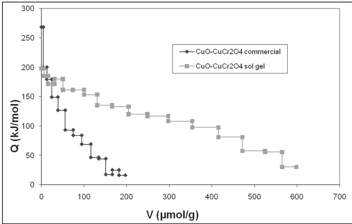
Figure 26 : chaleur différentielle d'adsorption en fonction de la quantité de \text{NH}_3 adsorbée
