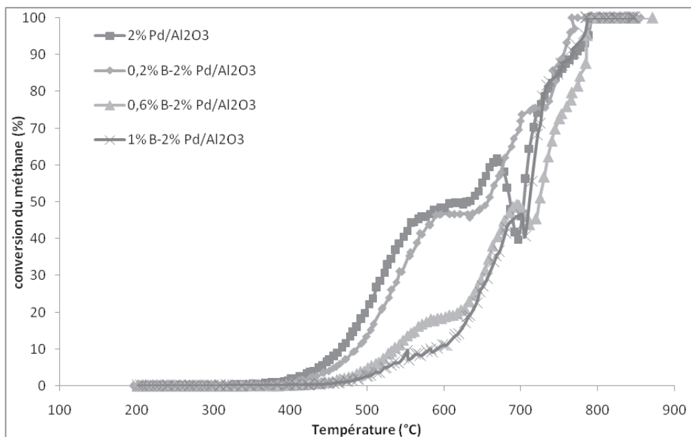
Figure 8 : activité catalytique en combustion du méthane lors de la descente en température des catalyseurs x\% B-2% Pd/ Al_2O_3 ( 0,2 \leq x \leq 1 )
