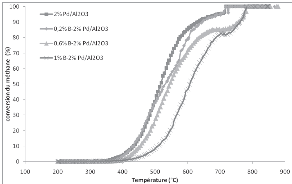
Figure 7 : activité catalytique en combustion du méthane lors de la première montée en température des catalyseurs x\% B-2% Pd/ Al_2O_3 ( 0,2 \leq x \leq 1 )
