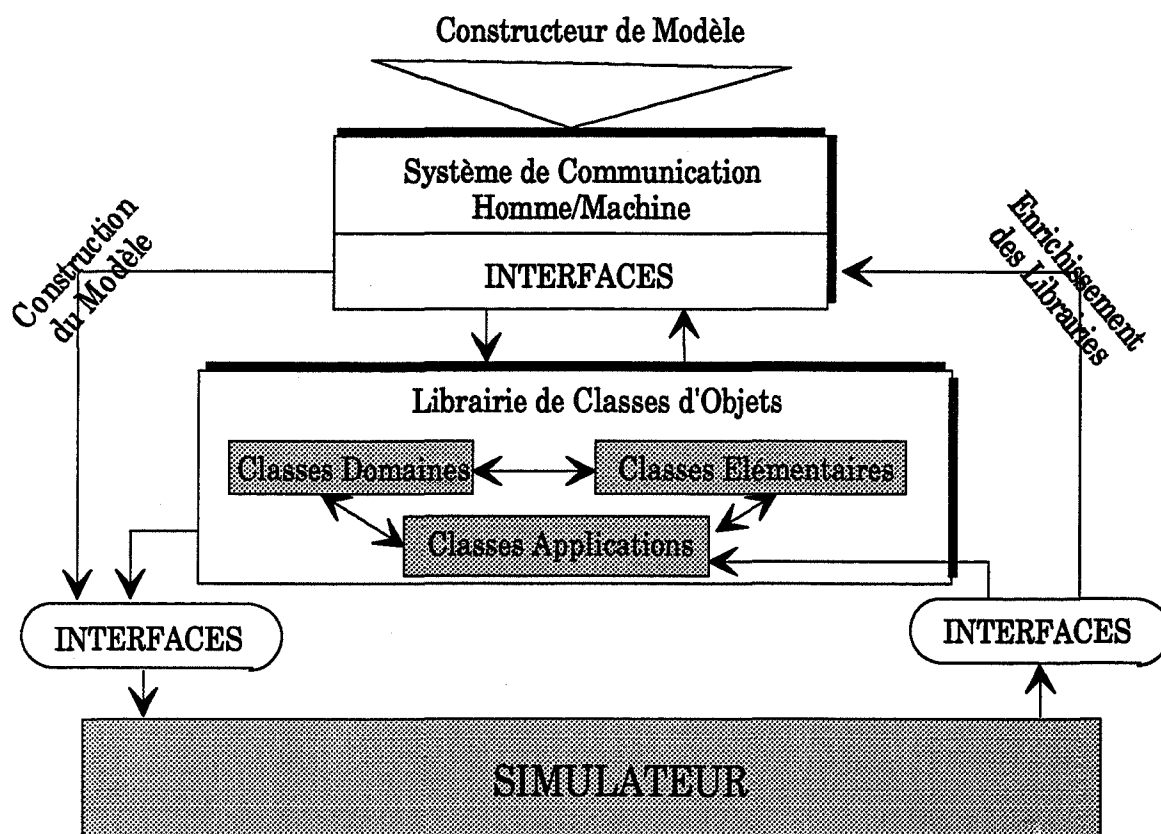
Figure 4-6 Architecture de Construction de Modèles de Simulation
