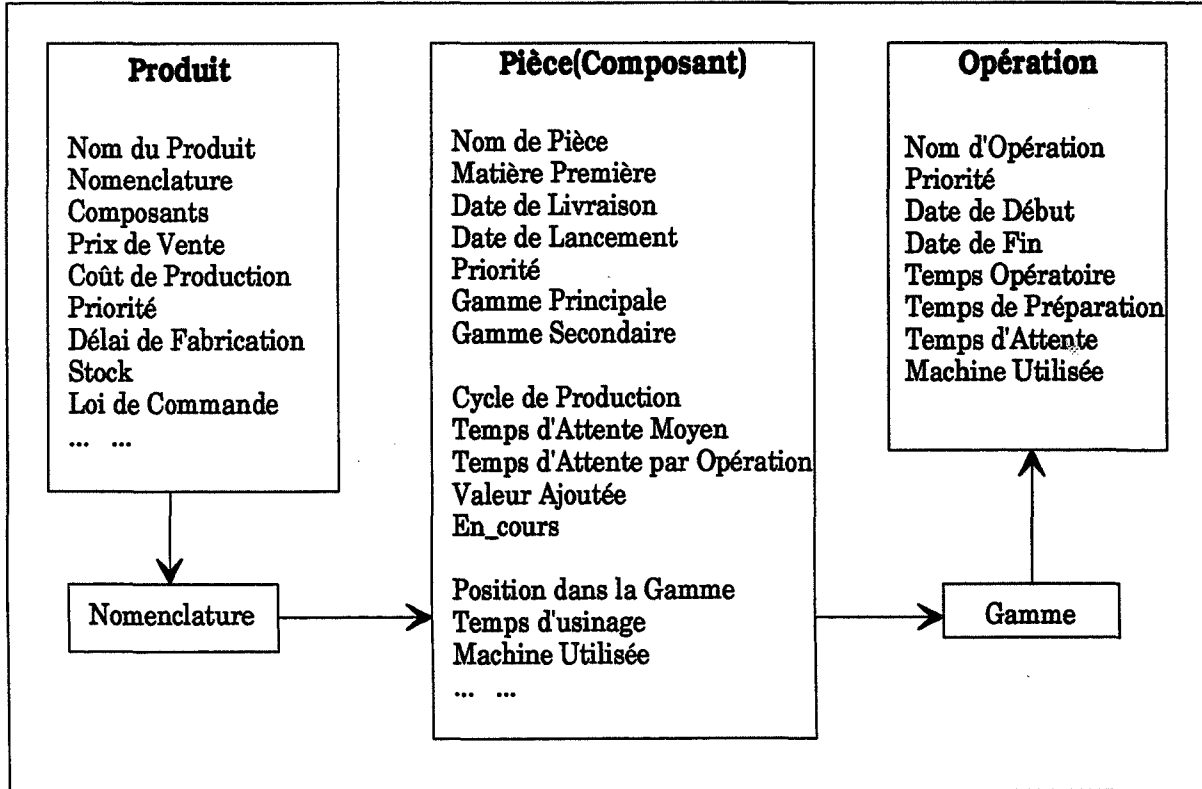
Figure 4-11 Liens entre Produit, Pièce et Opération
