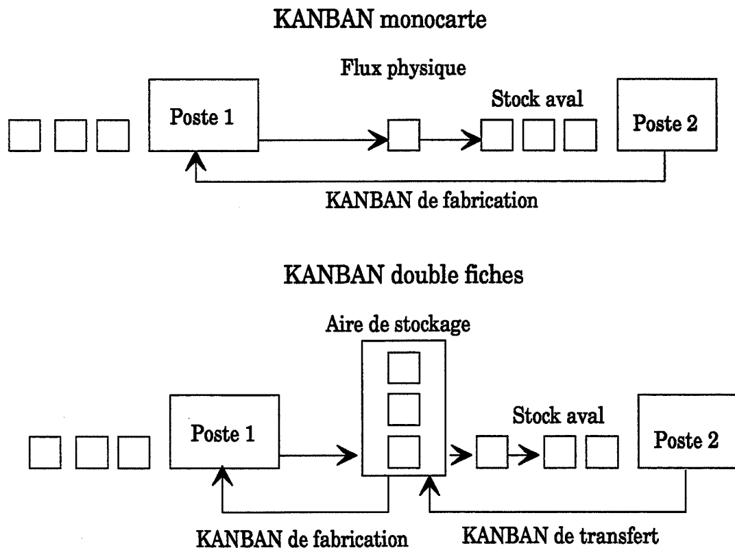
Figure 1-5 Méthode Kanban
