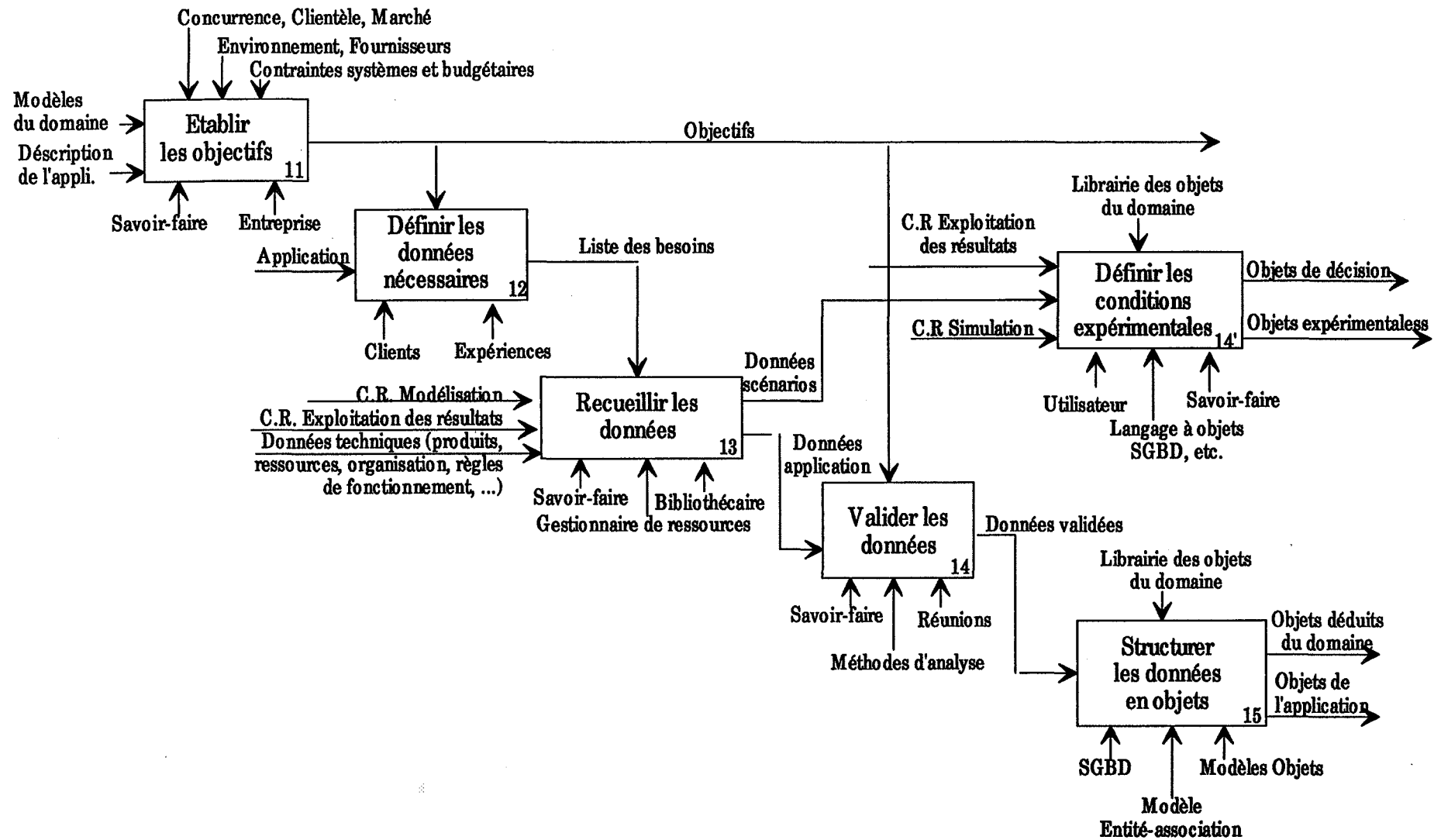
Figure 3-27 Diagramme A1: Analyser l'Application (les Systèmes de Production)
