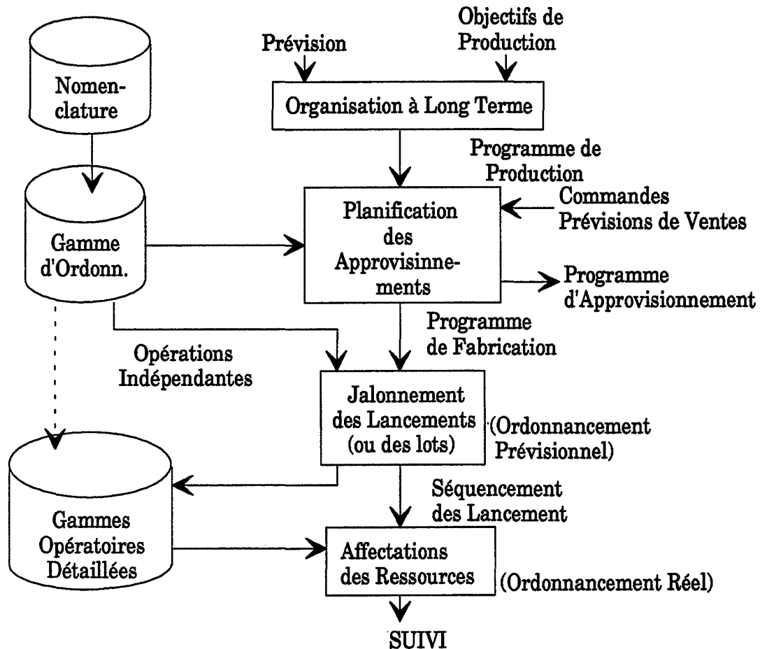
Figure 4-14 Schéma du Système de Commande de la Production
