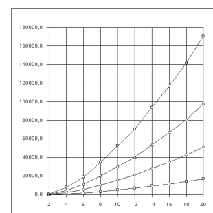
Rationnels
