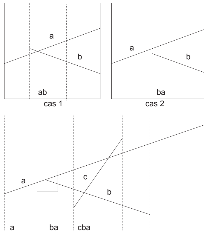
figure 4 Incohérences topologiques
