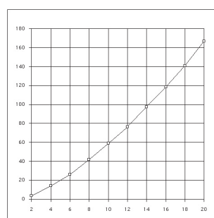
Paresseux
