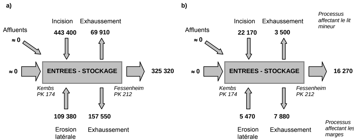
Figure 2.54 : Bilan des sédiments grossiers mobilisés entre le barrage de Kembs et le bouchon de Fessenheim entre 1990 et 2010 : a) Volumes totaux (en m³). b) Volumes annuels moyens (en m³/an)
