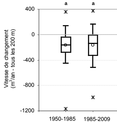
Figure 2.14 : Evolution de la vitesse de changement vertical dans la bande active entre 1950/56 et 2009 (en \text{m}^3/\text{an} , tous les 200 m jusqu'au PK 214 : n = 197 )
