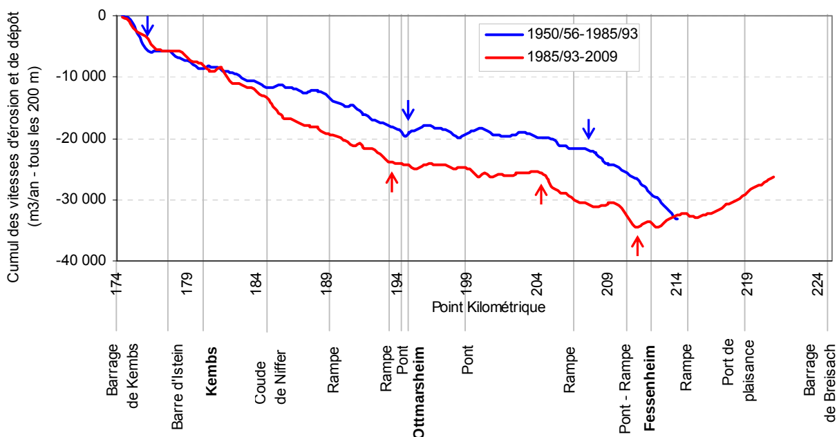
Figure 2.18 : Cumuls des vitesses d'érosion et de dépôt dans la bande active entre 1950/56 et 2009 (en \text{m}^3/\text{an}/\text{profils} en travers tous les 200 m : n = 197 ou 231). Les flèches indiquent les ruptures détectées avec le test de Hubert
