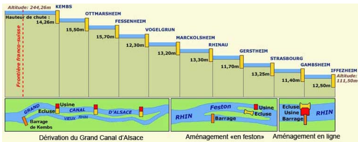
Figure 1.2 : Aménagement hydro-électrique du Rhin supérieur entre Kembs et Iffezheim : huit usines sont implantées en dérivation et deux usines sont implantées en ligne (d'après www.encyclopedia.bsditions.fr )
