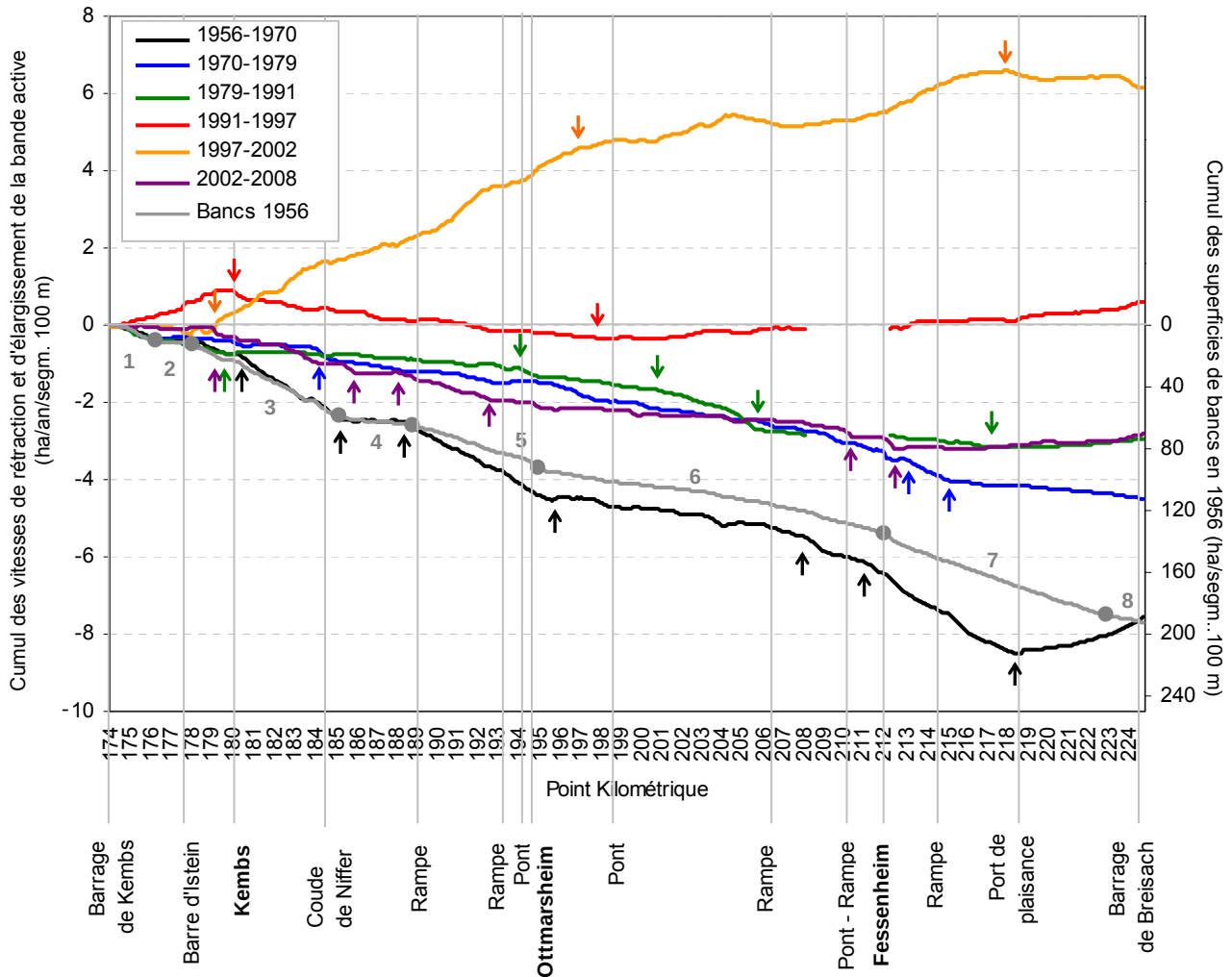
Figure 2.36 : Cumuls des vitesses de rétraction (valeurs négatives) et d'élargissement (valeurs positives) de la bande active entre 1956 et 2008 (en ha/an) et cumuls des surfaces de bancs en 1956 (en ha) (segments élémentaires de 100 m : n = 510). Les flèches indiquent les ruptures détectées avec le test de Hubert. Les points gris indiquent la position des ruptures détectées sur les surfaces de bancs et les chiffres gris indiquent le numéro des tronçons fluviaux homogènes
