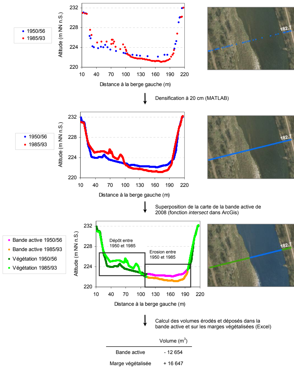
Figure 2.7 : Description de la procédure de calcul des volumes de sédiments érodés et déposés dans la bande active et sur les marges végétalisées à partir des profils en travers. Exemple du PK 182,7 entre 1950/56 et 1985/93. Illustration sur l'ortho-photographie d'avril 2008
