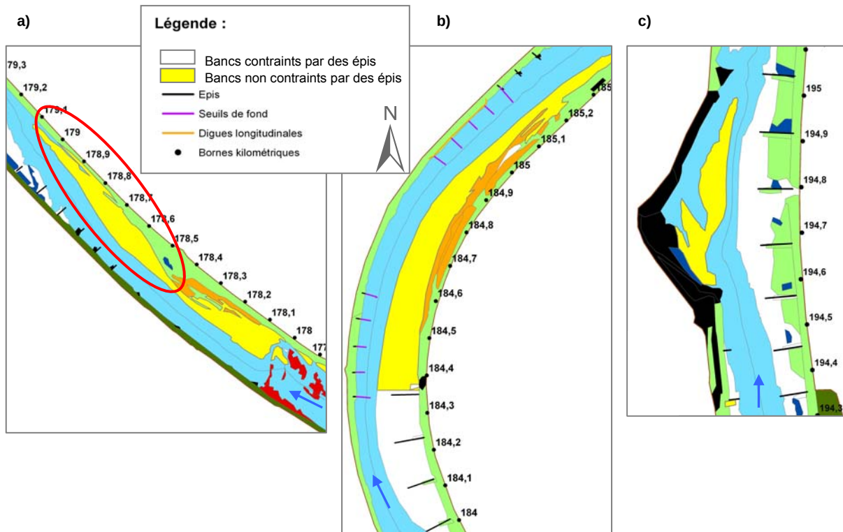
Figure 2.32 : Illustration de bancs non contraints par des épis sur la carte des unités physionomiques du Vieux Rhin en 1956 : aval de la barre d'Istein (a), coude de Niffer (b), bouchon d'Ottmarsheim (c). Le cercle rouge localise un banc « mixte », vraisemblablement induit à la fois par la barre d'Istein et par la convexité créée par les épis en rive gauche
