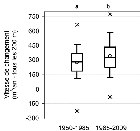
Figure 2.15 : Evolution de la vitesse de changement vertical sur les marges végétalisées entre 1950/56 et 2009 (en \text{m}^3/\text{an} , tous les 200 m jusqu'au PK 214 : n = 197 )
