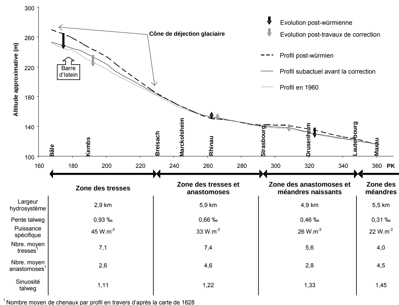
Figure 1.21 : Gradient longitudinal du Rhin supérieur entre Bâle et Maxau et caractérisation synthétique des secteurs du Rhin sauvage (1828) (d'après Carbiener, 1970 ; Carbiener et Dillmann, 1992 ; Schmitt, 2010)
