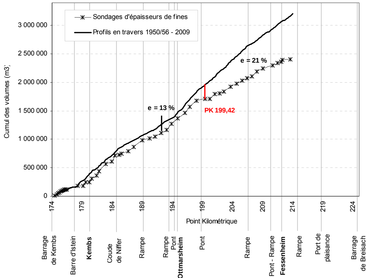
Figure 2.19 : Cumuls des volumes de sédiments déposés sur les marges depuis 1950 à partir de l'analyse des profils en travers et des sondages d'épaisseurs (en m 3 /profil en travers tous les 200 m : n = 197)
