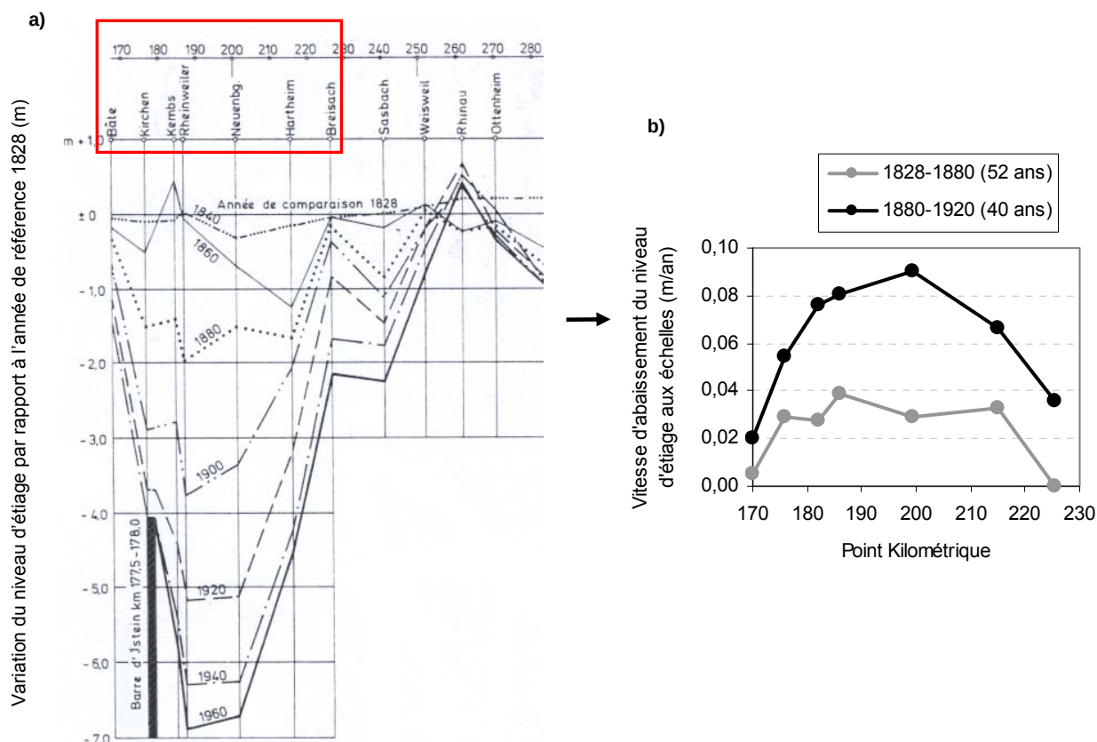
Figure 2.55 : a) Variations du niveau d'étiage ( 540 \text{ m}^3/\text{s} à Bâle) aux échelles limnimétriques entre les PK 170 et 280 depuis 1828. L'encadré rouge localise le tronçon d'étude (d'après CHR, 1977). b) Abaissement du niveau d'étiage par périodes entre 1828 et 1920
