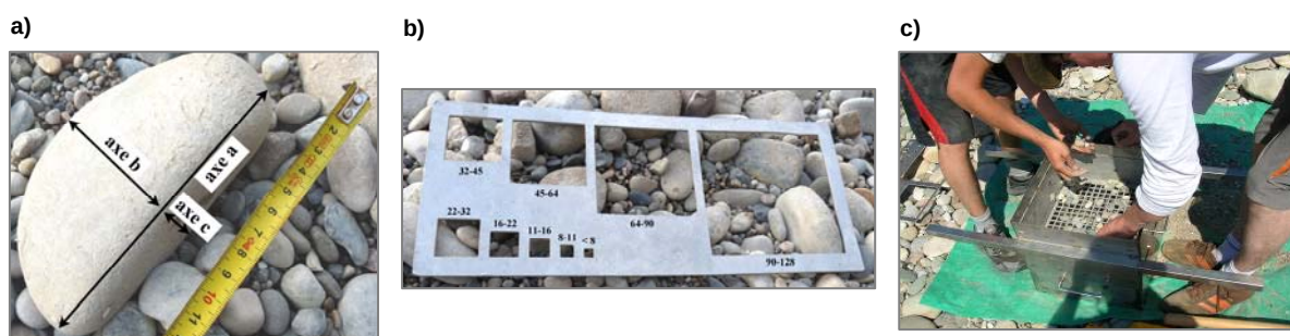
Figure 2.47: a) Représentation des trois axes caractéristiques d'une particule : a (grand), b (intermédiaire), c (petit). b) Gabarit à trous carrés. c) Tamis à maille carrée (clichés F. Arnaud, V. Ferrier, 2011)
