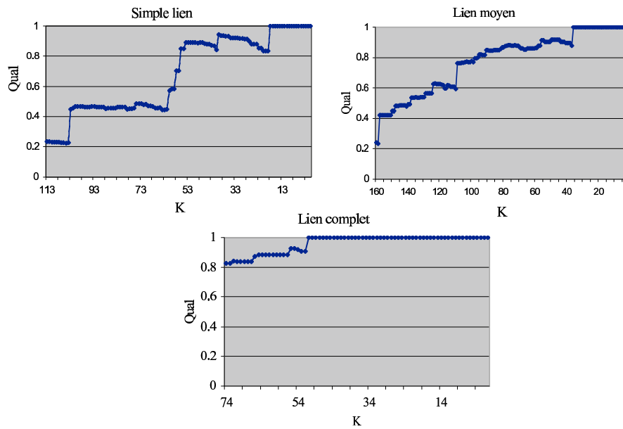
FIG. 5.3 – Représentation de la qualité pour les trois stratégies (méthode 1)
