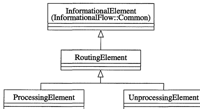
FIG. A.16 – Syntaxe abstraite de Simulation::InformationalFlow::Routing
