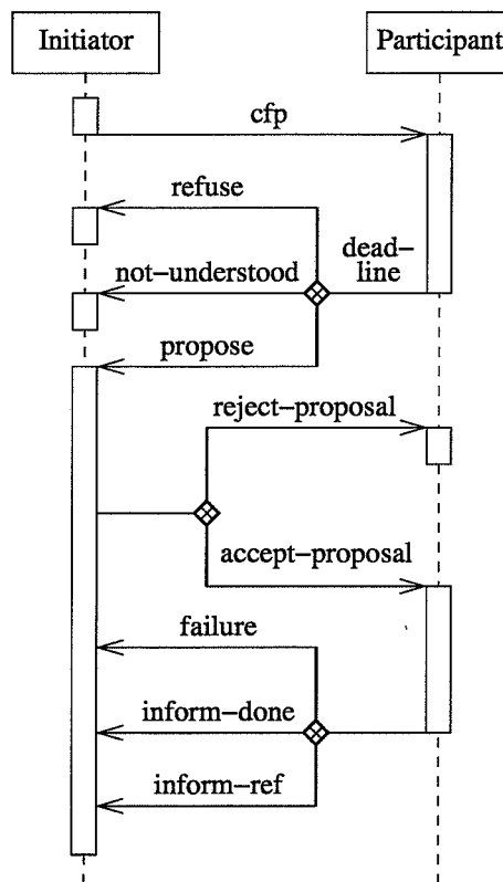
FIG. 6.1 – Protocole d'appel d'offre [ FIPA, 2001a ]
