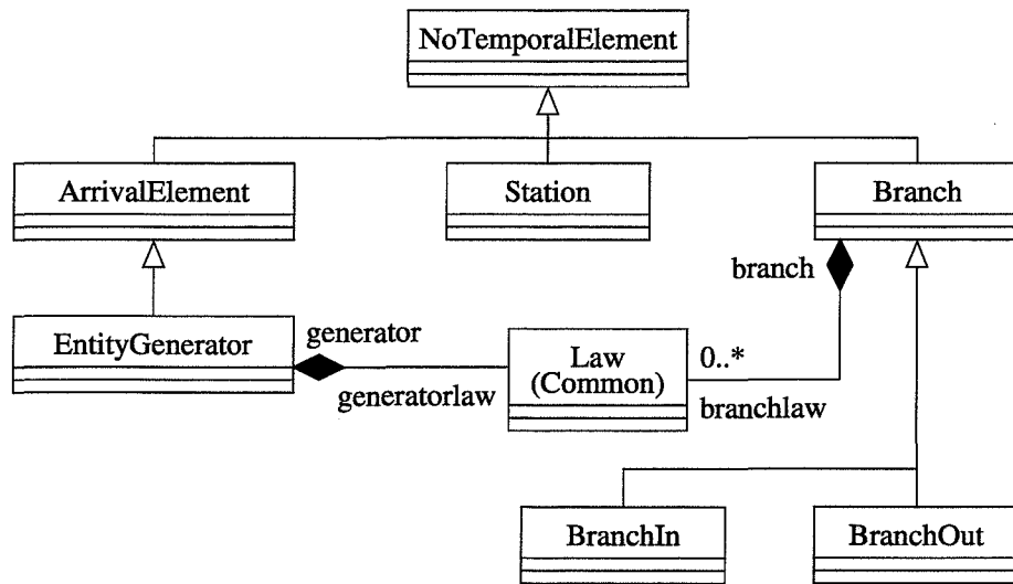
FIG. A.7 – Simulation::PhysicalFlow : Éléments avec traitement immédiat (2)
