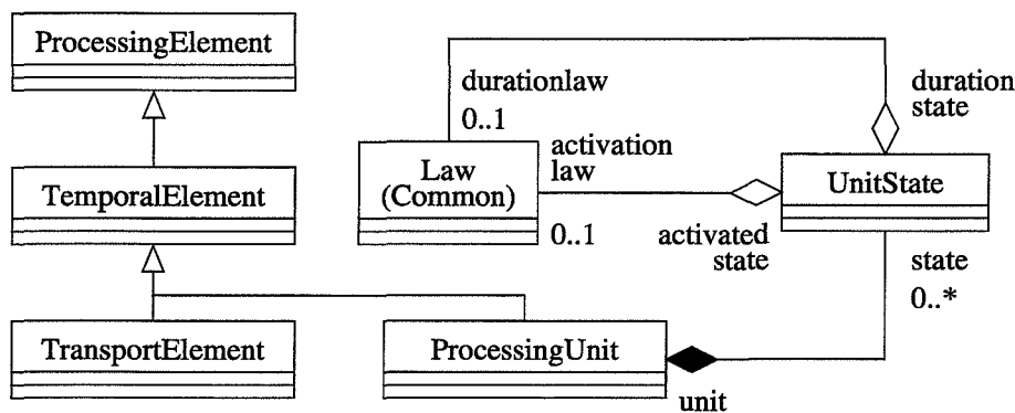
FIG. A.8 – Simulation::PhysicalFlow : Éléments avec traitement temporisé
