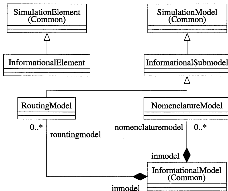
FIG. A.13 – Syntaxe abstraite de Simulation::InformationalFlow::Common
