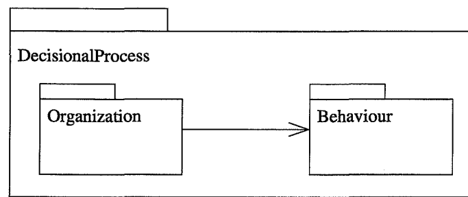
FIG. A.24 – Paquetage DecisionalProcess
