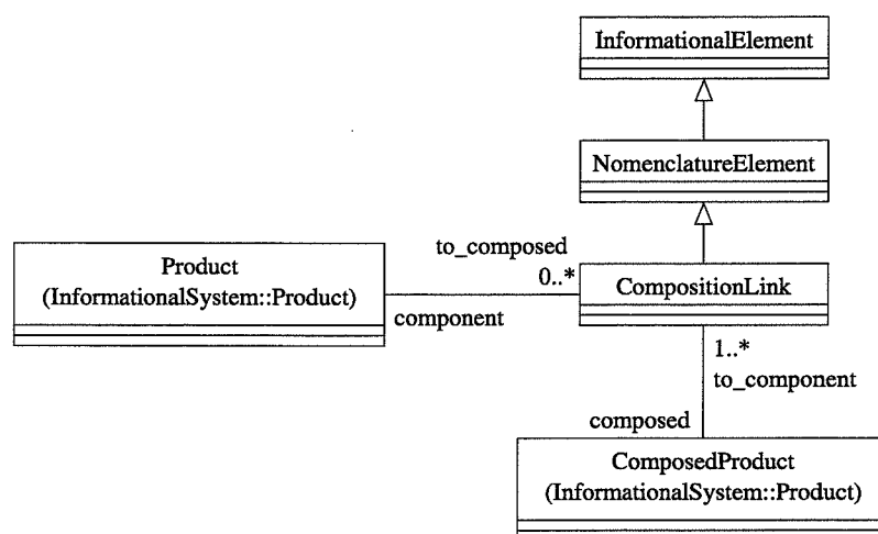
FIG. 9.8 – Extrait du métamodèle du sous-système informationnel
