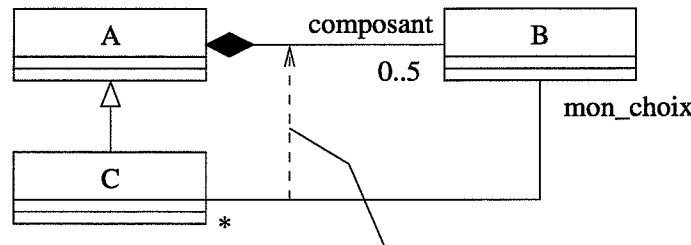
FIG. 9.9 – Extrait d'un métamodèle pour la vérification locale
