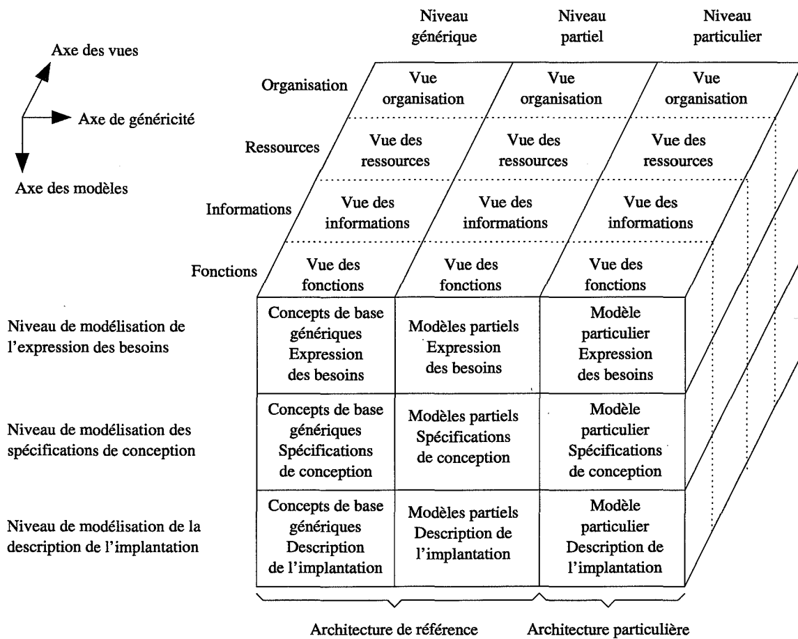
FIG. 4.4 – Le « cube » CIMOSA
