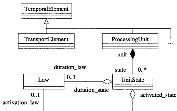
FIG. 9.7 – Extrait du métamodèle du sous-système opérationnel
