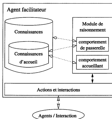
FIG. 10.2 – Architecture d'un agent facilitateur
