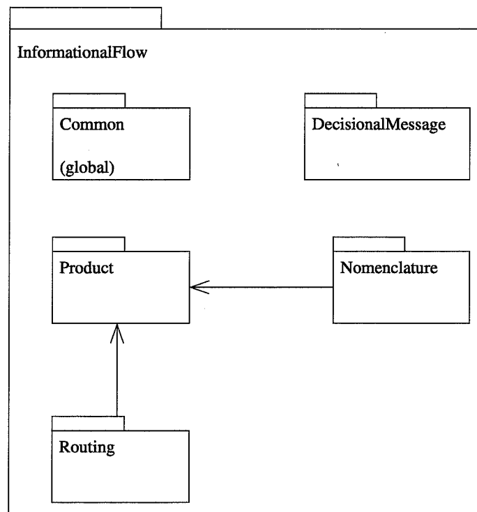
FIG. A.12 – Paquetage InformationalFlow
