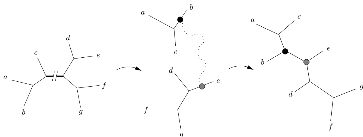
FIG. 3.11 – TBR . Après section (à gauche), un point de liaison est défini sur chaque sous-arbre (au centre). Ces deux points constituent les extrémités de la nouvelle branche joignant les deux sous-arbres (à droite).
