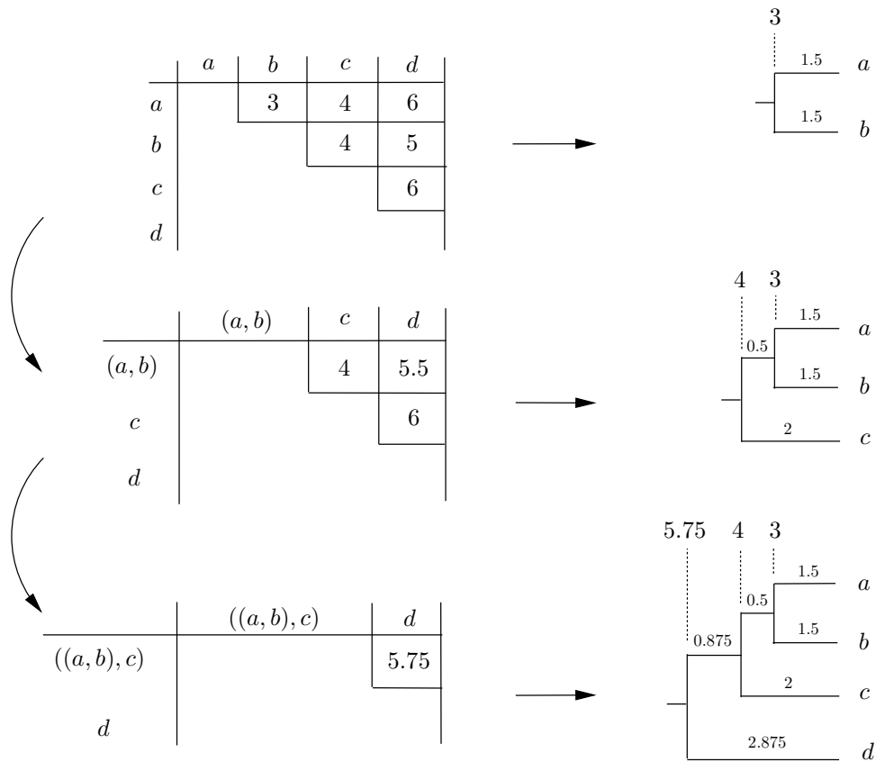
FIG. 1.3 – Construction d'un phénogramme par WPGMA. La matrice (à gauche) reporte les distances entre les noeuds agglomérés de l'arbre. Les positions de ces derniers sont indiquées par les valeurs situées au-dessus de l'arbre. Celles-ci correspondent aux distances minimales dans la matrice à chaque étape et désignent donc la suite de paires de noeuds agglomérés aboutissant au phénogramme complet.
