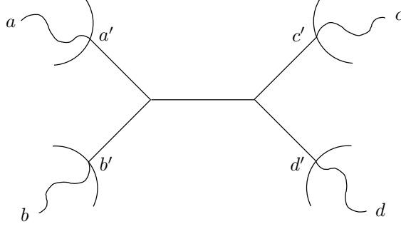
FIG. 4.3 – Arbre modèle. a , b , c et d désignent des noeuds externes, tandis que a' , b' , c' et d' correspondent à des noeuds internes, racines des sous-arbres A , B , C et D , présentant respectivement |A| , |B| , |C| et |D| UEs.
