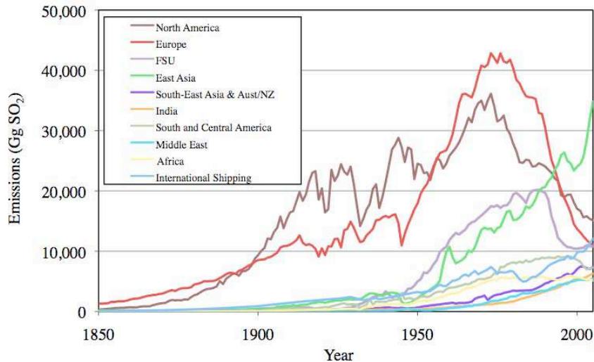
Figure 1.5 Tendances annuelles des émissions anthropiques de SO 2 par région (Amérique du Nord = USA + Canada; Asie de l'Est = Chine + Japon + Corée du sud) de 1850 à 2005 estimées à partir d'inventaires des émissions de SO 2 (Smith et al., 2011).
