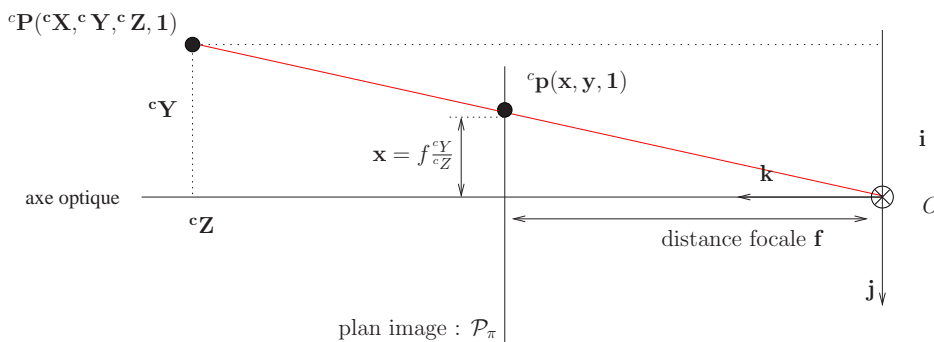
FIG. 2.3 – Projection centrale et notations
