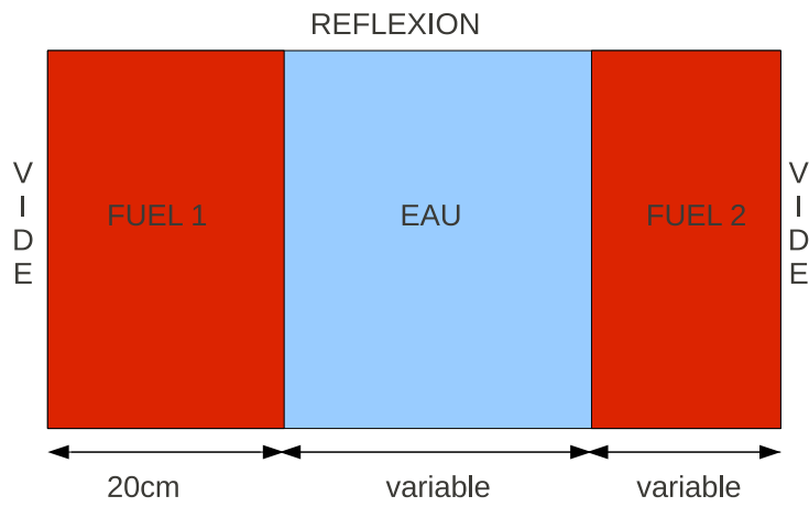
FIGURE 3.6 – Géométrie du cas test
