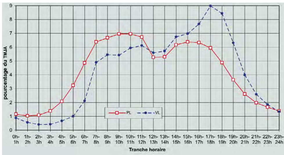
Figure 1.4 : profils moyens journaliers annuels de trafic Véhicules Légers (VL) et Poids Lourds (PL) sur Routes Nationales par tranche horaire. (source : Préviation du bruit routier – SETRA [7])
