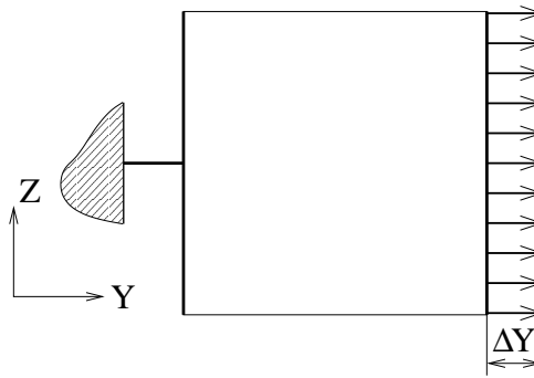
FIGURE 4.17 – Conditions limites appliquées à l’essai de traction
