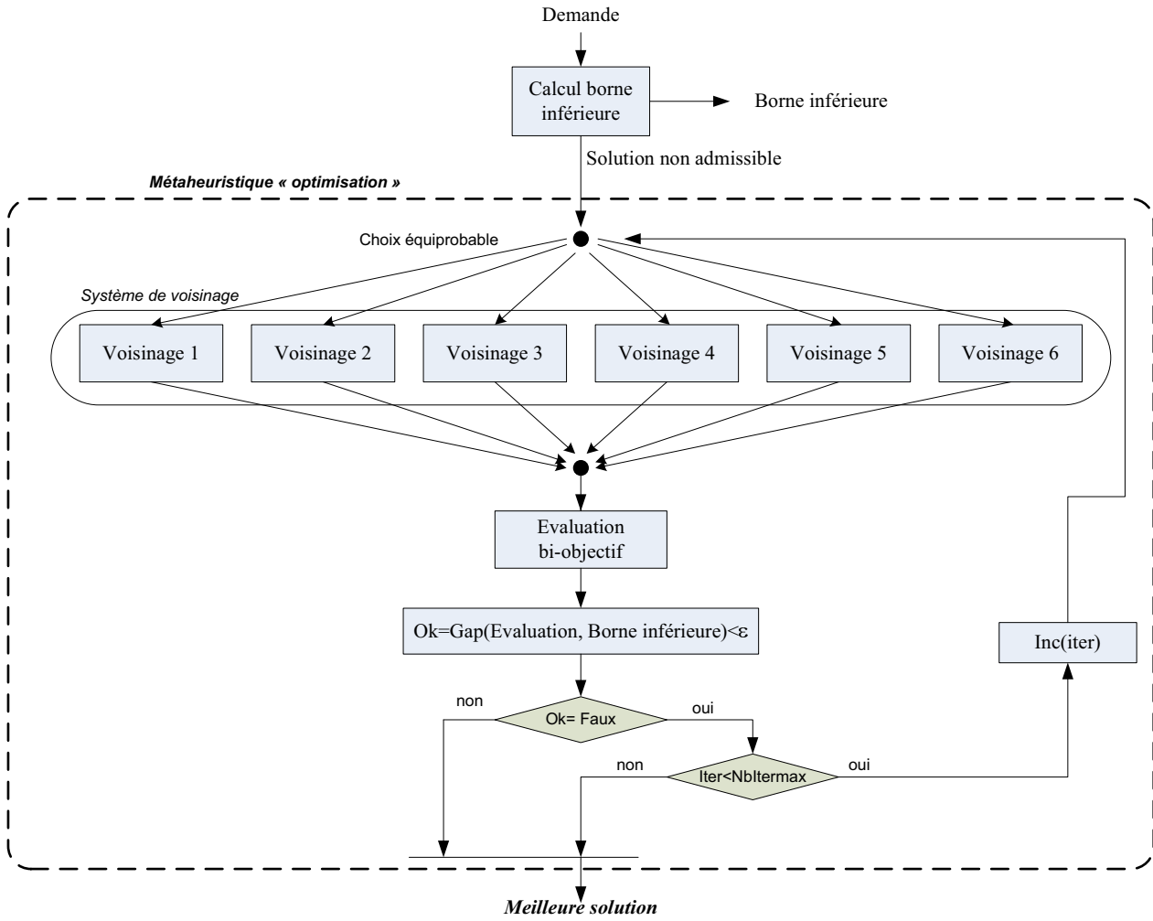
Figure 3.17 – Algorithme de principe de notre méthode d’optimisation avec fonction bi-objectif
