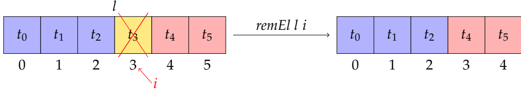
Figure 4.1 — Suppression de l'élément d'indice i (ici, decode\ i = 3 ) dans l
