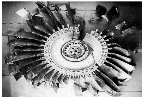
FIG. 4.6 – Roue aubagée reconstruite suite à une rupture de disque due aux phénomènes de fatigue
