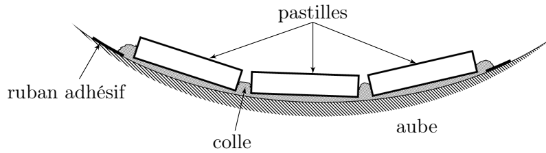
FIG. 5.34 – Schéma de la mosaïque collée sur l'intrados de l'aube de soufflante.
