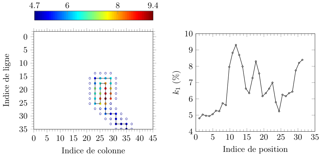
(a) Chemin suivi lors de la recherche de la position optimale. (b) Évolution du facteur de couplage modal en fonction de la position sur la surface de l'aube.
