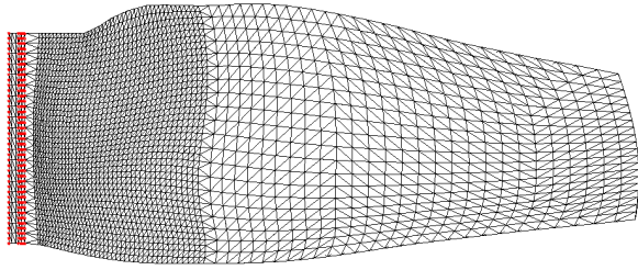
FIG. 5.24 – Maillage régulier de l'échasse de l'aube fan.
