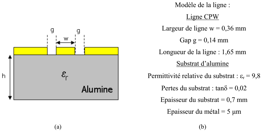
Figure II-12 – a) Modèle de ligne CPW simple sur substrat d'alumine et b) ses paramètres
