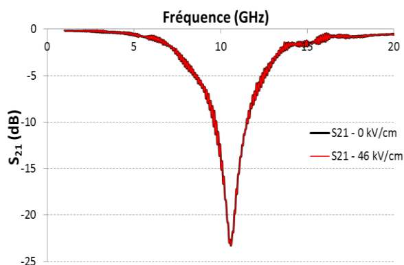
Figure IV-27 - Variation du paramètre S_{21} , en fonction de la fréquence avec et sans champ statique appliqué, d'un résonateur à stub réalisé sur un film \text{La}_2\text{Ti}_2\text{O}_7 (LTON-590)
