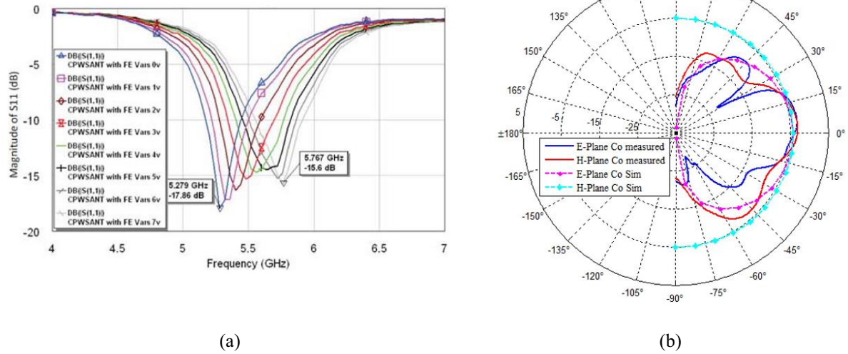
Figure I-23 – a) Coefficient de réflexion en fonction de la tension continue et b) rayonnement ( V=0V ) de l'antenne avec les capacités ferroélectriques
