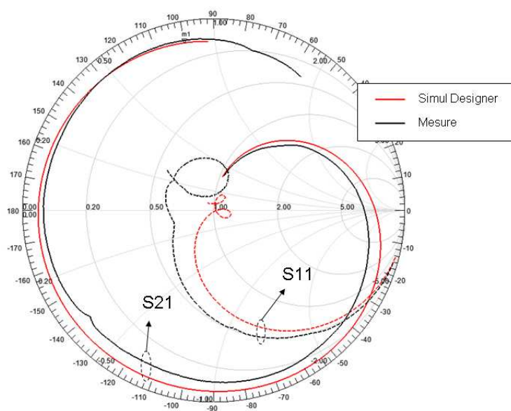
Figure A2-8 - Paramètres S
