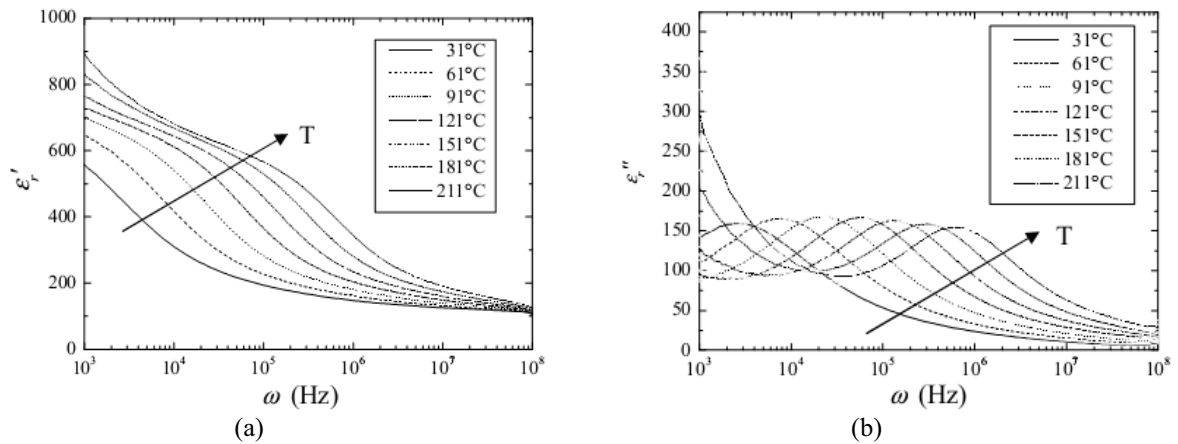
Figure I-37 – Evolution de la permittivité réelle et imaginaire du composé (Ba_{0,90}Sr_{0,10})TiO_3 en fonction de la fréquence à différentes températures de mesure [123]
