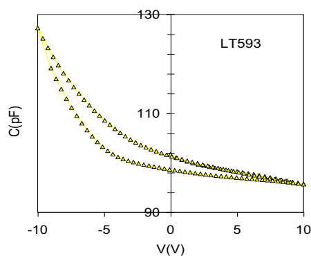
Figure IV-24 - Evolution de la capacité, à 100 kHz et en fonction de la tension statique appliquée, du film \text{La}_2\text{Ti}_2\text{O}_7 déposé sur \text{Nb:SrTiO}_3 (LTON-593)
