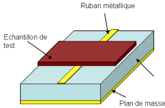
Figure II-5 - Ligne microruban chargée avec l'échantillon
