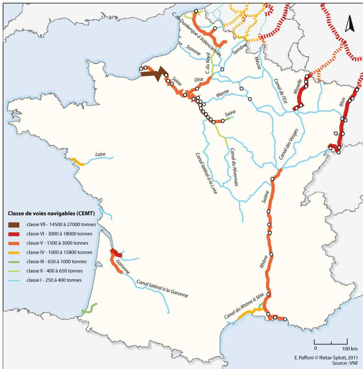
Figure I-2. Classes et gabarits des voies navigables en France en 2009
