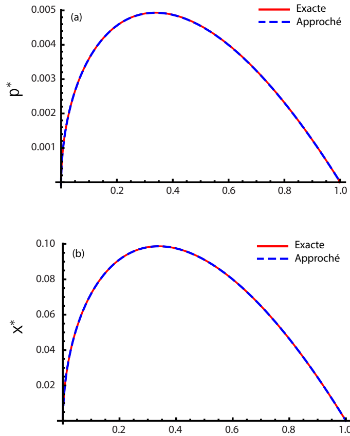
FIGURE B.1 – (a) Comparaison entre l'expression exacte de p^*(\gamma) (cf. équation (B.2) ; ligne rouge) et l'expression approchée (cf. équation (B.10) ; ligne pointillée bleue). (b) Même comparaison pour x^*(\gamma) . \zeta = 0.5 et \lambda = 0.95 .
