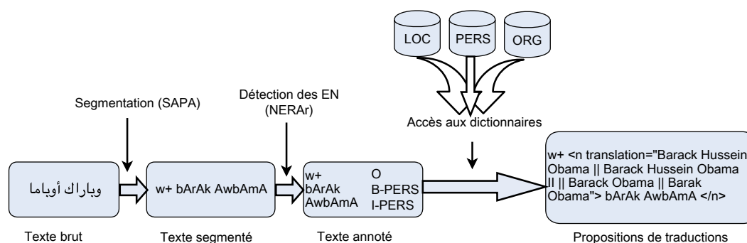
Figure 5.5: Méthode de prétraitement du texte en arabe en combinant segmentation du texte, détection des EN et proposition de traductions.
