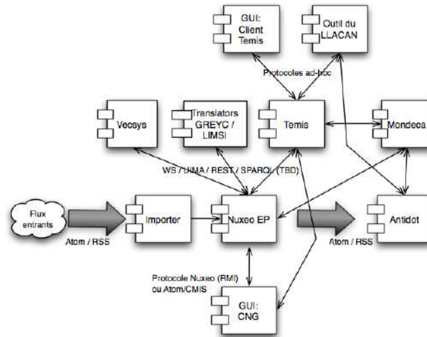
Figure 7.2: Architecture de la plateforme SAMAR telle que illustrée par Nuxeo 2 .
