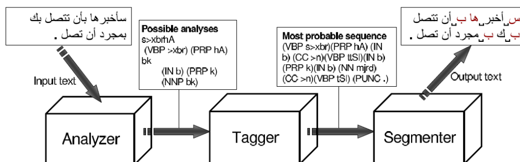
Figure 4.4: L'architecture du segmenteur MorphTagger (Mansour, 2010)
