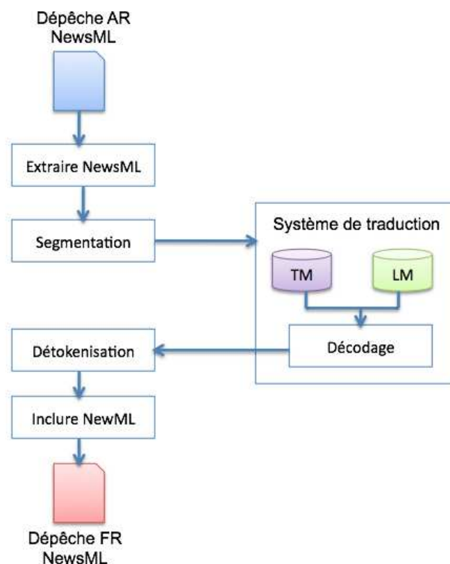
Figure 7.3: Chaîne de traitement d'une dépêche AFP pour la traduction de l'arabe vers le français.
