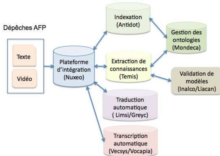
Figure 1: Schéma fonctionnel du projet SAMAR et interaction entre les partenaires.
