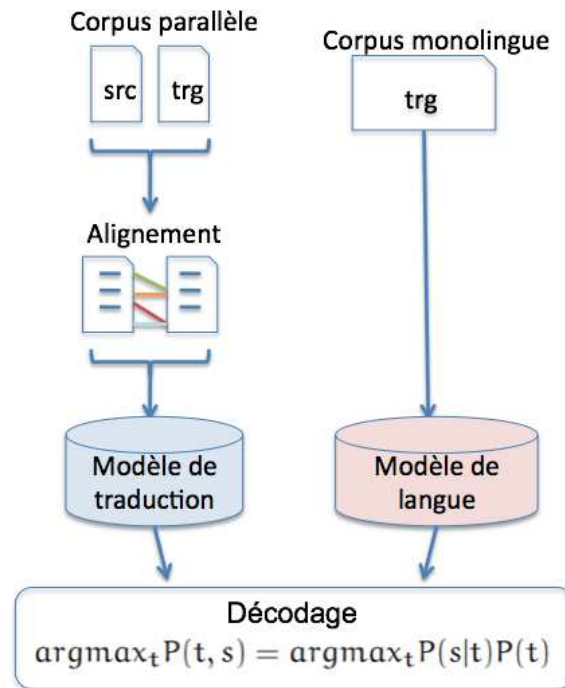
Figure 1.4: Système de traduction automatique.
