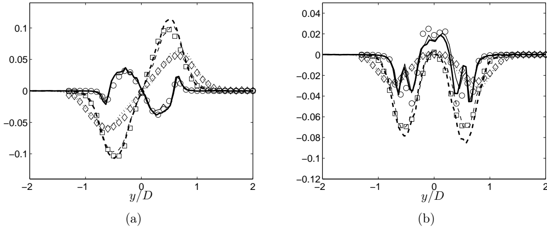
FIGURE 4.3 – Comparaison des moments croisés d’ordre 3 à un nombre de Reynolds de 3600. PIV-2C (trait fin), TR-PIV2C (trait épais), et ADL3C (symboles) en x = 2.2D (—, \circ ); x = 3D (- - -, \square ); x = 3.8D ( \cdots , \diamond ). (a) \overline{vq^2}/U_0^3 , (b) \overline{uq^2}/U_0^3 .
