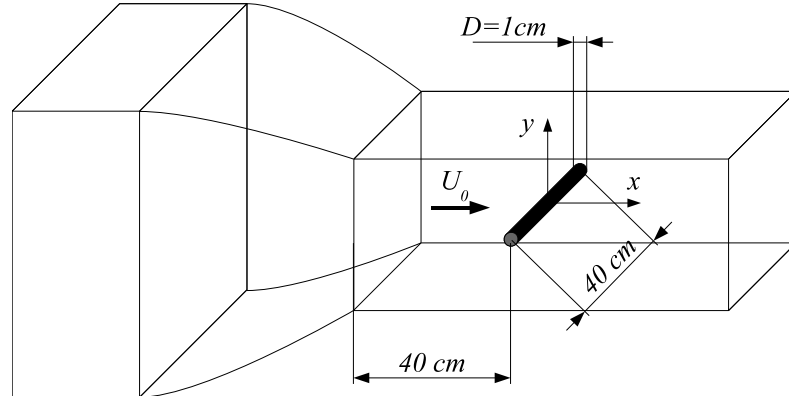
FIGURE 2.4 – Mise en place du cylindre dans la soufflerie
