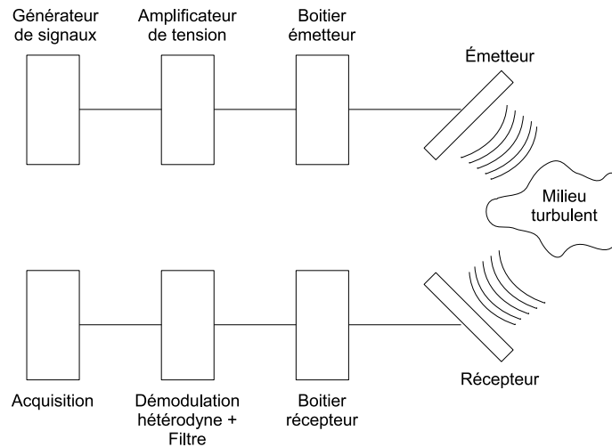
FIGURE 2.15 – Chaîne de mesure de diffusion acoustique
