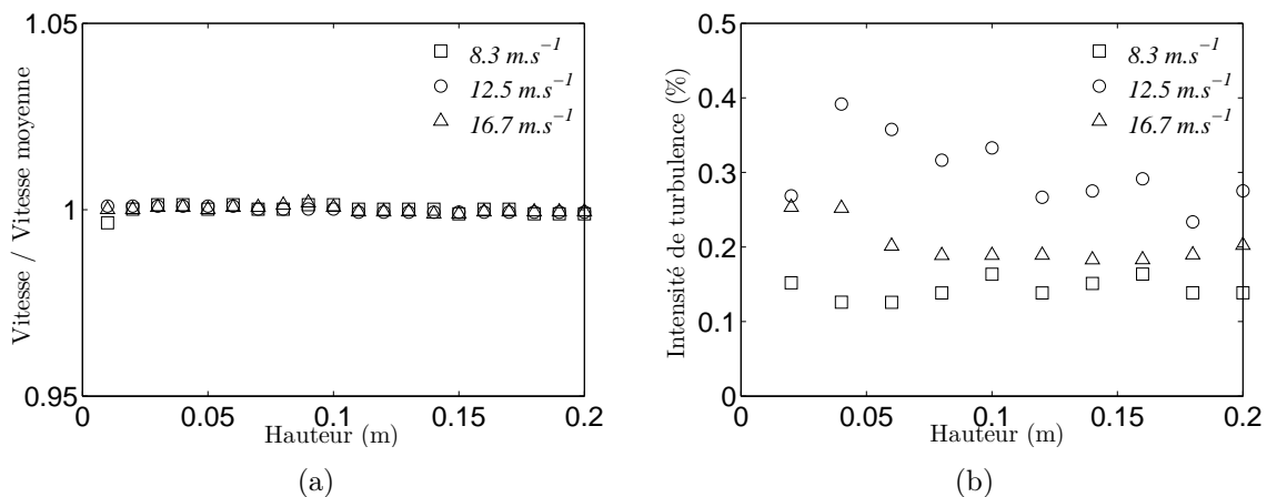
FIGURE 2.3 – Profil vertical de vitesse moyenne longitudinale (a) et d'intensité de turbulence (b)
