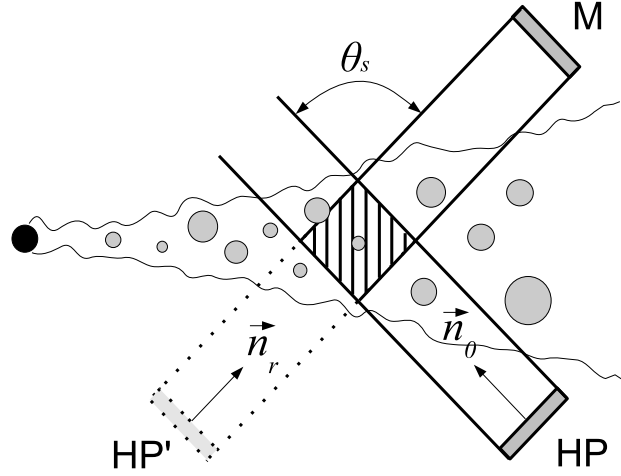
FIGURE 2.14 – Mise en place du haut-parleur et du microphone au sein de l'écoulement turbulent
