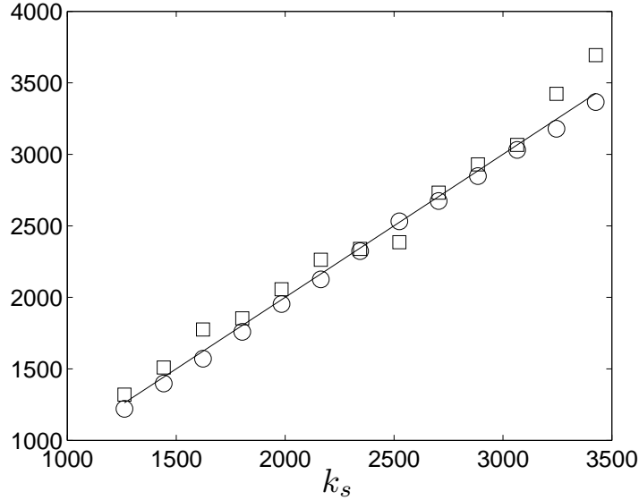
FIGURE 3.4 – Comparaison des moments d'ordre 1 et 2 calculés par le biais de la diffusion acoustique et par anémométrie au fil chaud. — : k_s = k_s , \circ : 2\pi\mu_f/\bar{U} , \square : 2\pi\sigma_f/(\bar{u}^2)^{1/2} . x = 50D , y = 0D , Re_D = 4800
