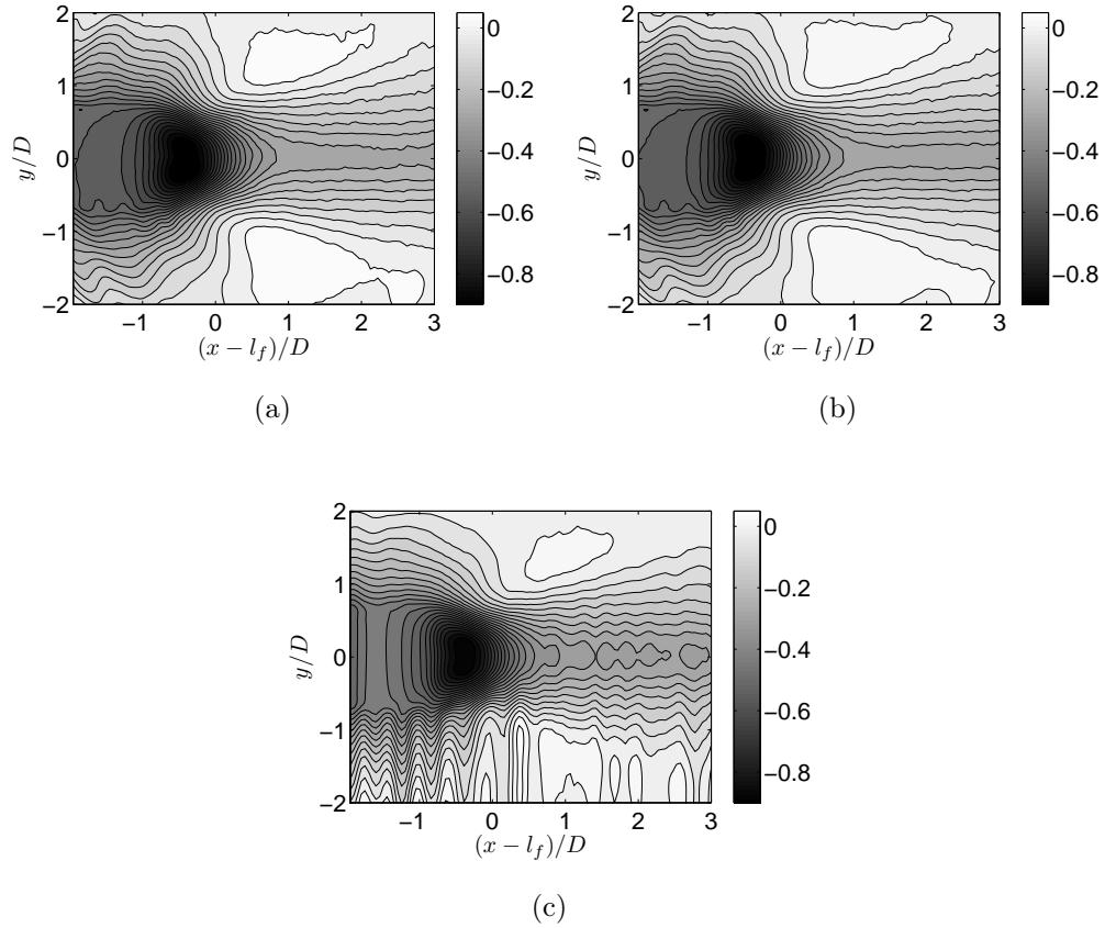
FIGURE 4.13 – (a) Moyenne temporelle des fluctuations ordonnées de la pression, (b) par le biais de (4.30), (c) Coefficient de pression moyen calculé à partir du bilan de quantité de mouvement.
