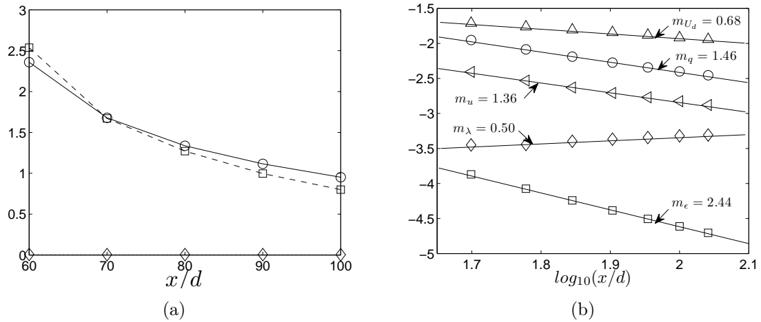
FIGURE 5.1 – (a) Termes du bilan énergétique en un point (5.1) sur la ligne centrale. \square -\frac{1}{2}\overline{U}\frac{\partial \overline{q^2}}{\partial x} , \circ \overline{\epsilon} , \diamond (\overline{u^2} - \overline{v^2})\frac{\partial \overline{U}}{\partial x} . (b) Exposant de décroissance sur la ligne centrale; \circ \log_{10}(\overline{q^2}/U_0^2) , \triangleleft \log_{10}(\overline{u^2}/U_0^2) , \square \log_{10}(\overline{\epsilon}D/U_0^3) , \diamond \log_{10}(10^{-1}\lambda/D) , \triangle \log_{10}(U_d^2/U_0^2) , les droites pleines correspondent à une approximation linéaire.
