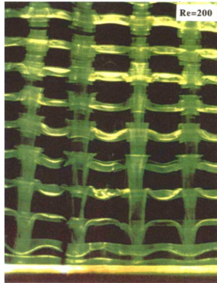
FIGURE 3 – Visualisation de la dégénérescence en trois dimensions de l’allée de Bénard-von Kármán. Le nombre de Reynolds est de 200. Il s’agit d’une vue de dessus, le cylindre est placé horizontalement et l’écoulement parcourt l’image de bas en haut. D’après Williamson [141]
