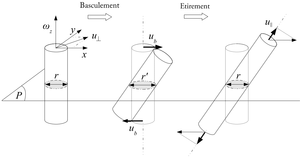
FIGURE 3.7 – Schématisation de l'effet du basculement-étirement sur un rouleau de vorticit .
