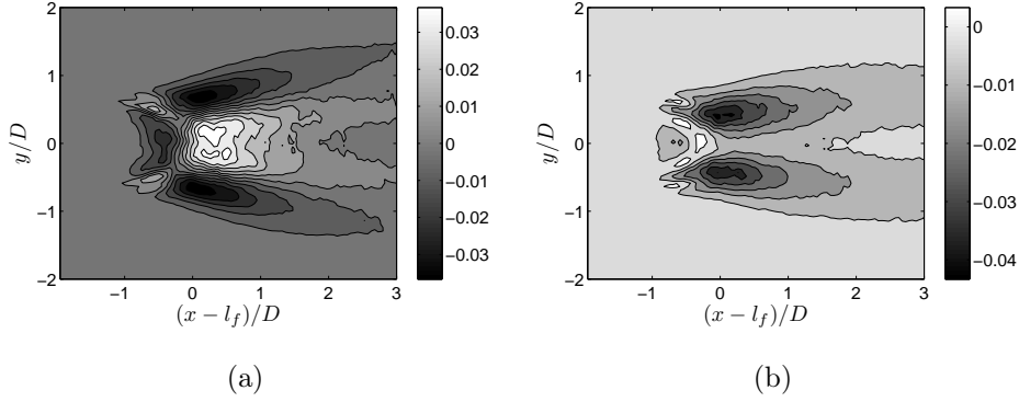
FIGURE 4.19 – (a) Diffusion des fluctuations aléatoires par le champ cohérent \frac{1}{2} \frac{\partial \overline{u_j \langle q'^2 \rangle}}{\partial x_j} , (b) Production de fluctuations aléatoires par le champ cohérent \overline{\langle u'_i u'_j \rangle} \frac{\partial \overline{u_i}}{\partial x_j}
