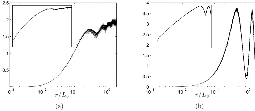
FIGURE 3.9 – Comparaison des hypothèses de Taylor globale (—) et locale (.....) à x = 7D , y = 0D et Re_D = 3600 (ADL3C). (a) composante u et (b) composante v . Insert : représentation log-log.
