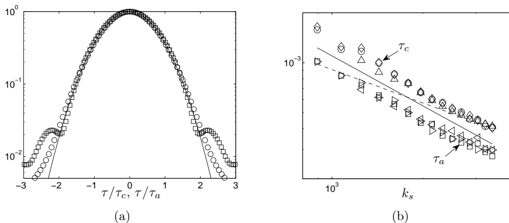
FIGURE 3.6 – (a) Corrélacion du nombre complexe et de son amplitude en fonction de la séparation spatiale. \circ : \rho_{\omega\omega} ; \square : \rho_{|\omega||\omega|} ; — Gaussienne. (b) Évolution des temps caractéristiques \tau_c/\sqrt{u^2} et \tau_a/\sqrt{u^2} en fonction du nombre d'onde pour différents nombres de Reynolds Re_D = 3000, 4800, 6000 . — : prédiction de Tennekes k_s^{-1} ; ..... : prédiction de Kolmogorov k_s^{-2/3} .
