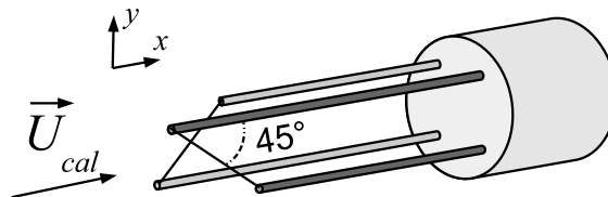
FIGURE 2.8 – Représentation schématique d'une sonde double en X
