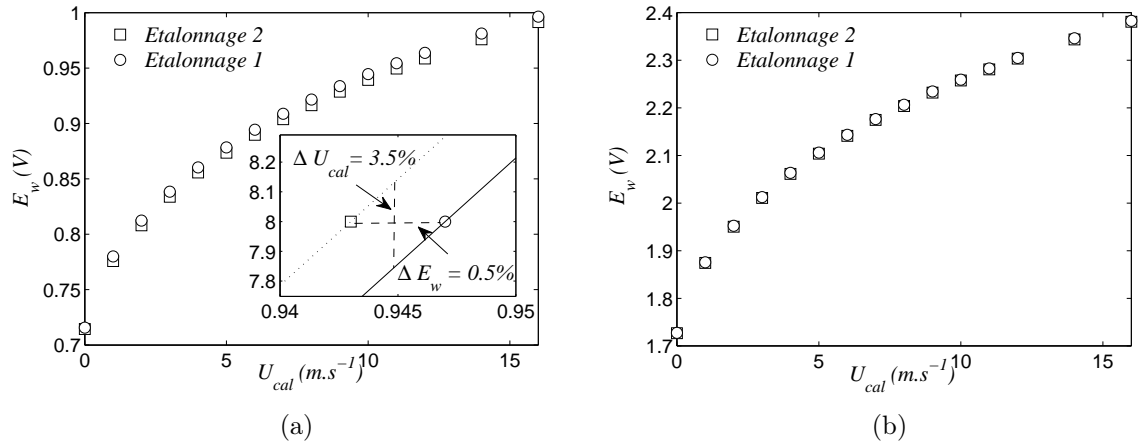
FIGURE 2.6 – Étalonage sans le système de régulation (a) Étalonage avec le système de régulation (b)
