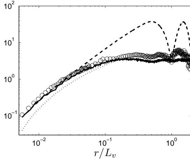
FIGURE 4.8 – Test d’isotropie locale sur les fonctions de structure d’ordre 2 en x = 7D \equiv x - l_f = 4.4D sur la ligne centrale du sillage, à un nombre de Reynolds de 3600. \cdots\cdots (\Delta u)^2 , - - - (\Delta v)^2 , — (\Delta w)^2 , \circ relation (4.18).
