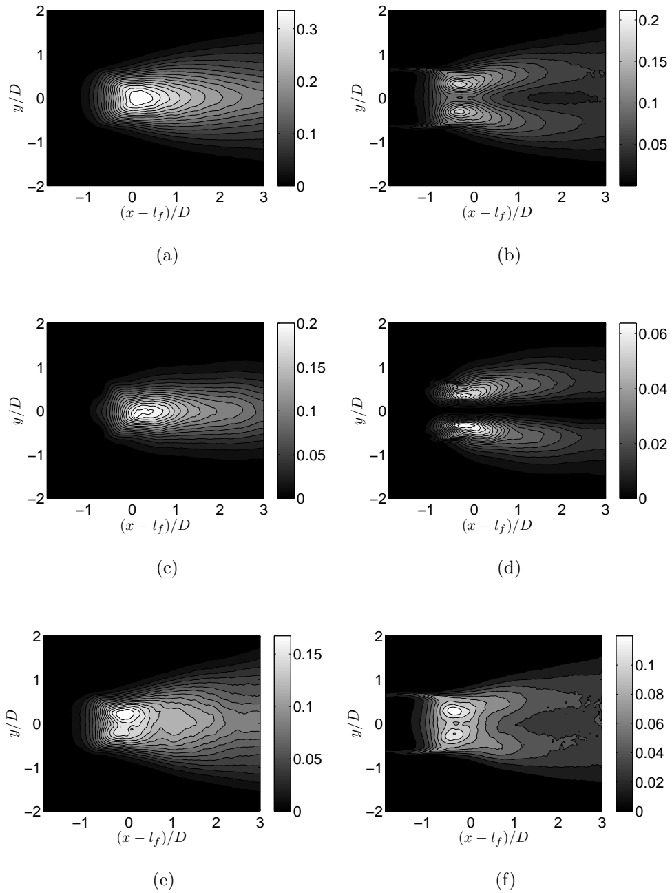
FIGURE 4.11 – Variance des fluctuations de vitesse totales, cohérentes et aléatoires issues de la technique TR-PIV2C à un nombre de Reynolds de 3600. (a) \overline{v^2}/U_0^2 , (b) \overline{u^2}/U_0^2 , (c) \overline{\tilde{v}^2}/U_0^2 , (d) \overline{\tilde{u}^2}/U_0^2 , (e) \overline{v'^2}/U_0^2 , (f) \overline{u'^2}/U_0^2
