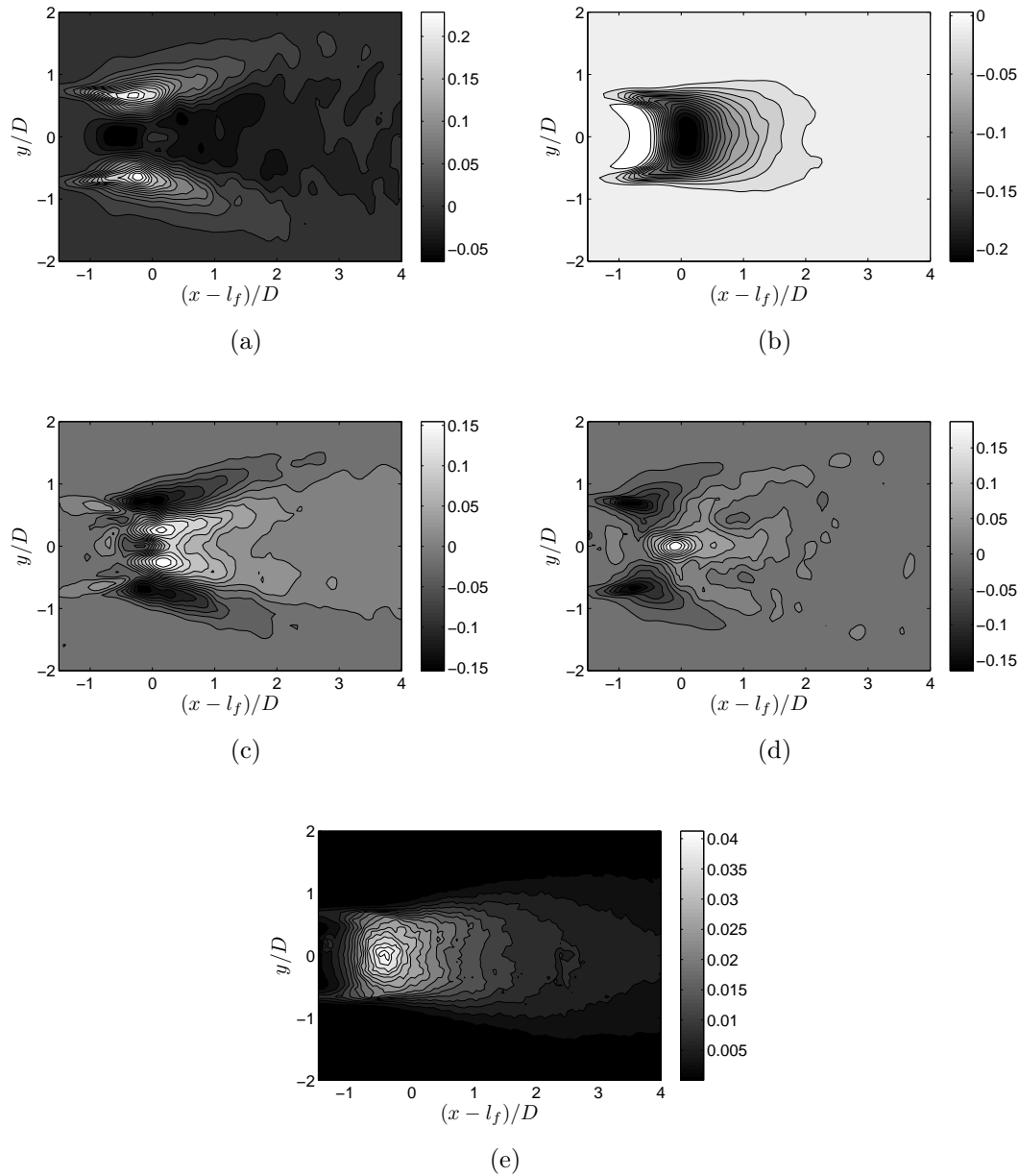
FIGURE 4.10 – Termes du bilan d'énergie cinétique turbulente mesurés par la PIV2C à un nombre de Reynolds 3600. Chaque terme est multiplié par D/U_0^3 . (a) Advection \frac{1}{2}\overline{U}_j \frac{\partial q^2}{\partial x_j} . (b) Production \overline{u_i u_j} \frac{\partial \overline{U}_i}{\partial x_j} . (c) Diffusion turbulente \frac{\partial \overline{u_j q^2}}{\partial x_j} . (d) Diffusion par la pression \frac{\partial \overline{u_j p}}{\partial x_j} . (e) Dissipation estimée par la relation \alpha_{PIV} \overline{\epsilon}_{PIV}
