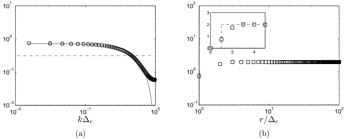
FIGURE 2.11 – (a) Réponse spectrale à un bruit blanc. Trait d'axe : Réponse -3dB \circ : E_{uu}(k_x) , \square E_{vv}(k_x) , — sinus cardinal. (b) Réponse "physique" à un bruit blanc \circ : (\Delta u)^2 , \square (\Delta v)^2 , - - - fonction créneau.
