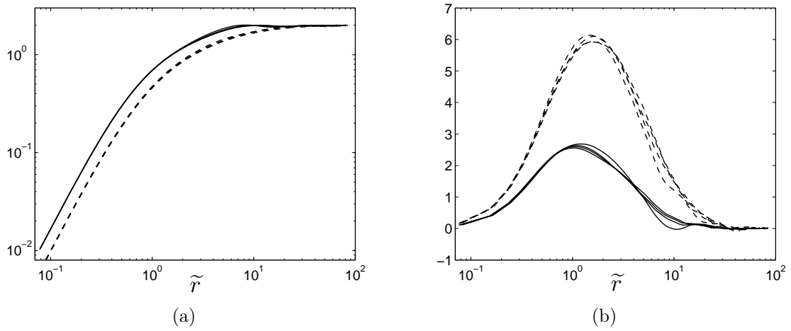
FIGURE 5.2 – (a) Fonctions de structure d'ordre 2 représentées en fonction \tilde{r} = r/\lambda pour x/D = 50, 70, 90, 110 . - - - - : f_u = \overline{(\Delta u)^2}/\overline{u^2} et ——— : f_q = \overline{(\Delta q)^2}/\overline{q^2} . (b) Fonctions de structure d'ordre 3 en fonction de \tilde{r} = r/\lambda pour x/d = 50, 70, 90, 110 . - - - - : g_u \tilde{r}^{-1} = -\overline{(\Delta u)^3} R_\lambda \left( \overline{u^2} \right)^{-3/2} \tilde{r}^{-1} et ——— : g_q \tilde{r}^{-1} = -\overline{\Delta u (\Delta q)^2} R_\lambda \left( \overline{q^2} \right)^{-3/2} \tilde{r}^{-1}
