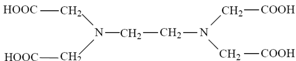
Figure 28 : Formule semi-développée de l'EDTA
